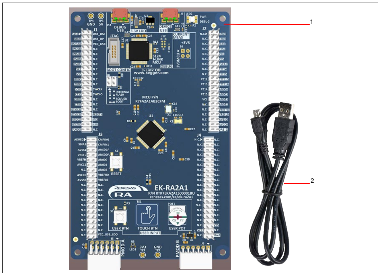
図 1 EK-RA2A1 評価キット構成
