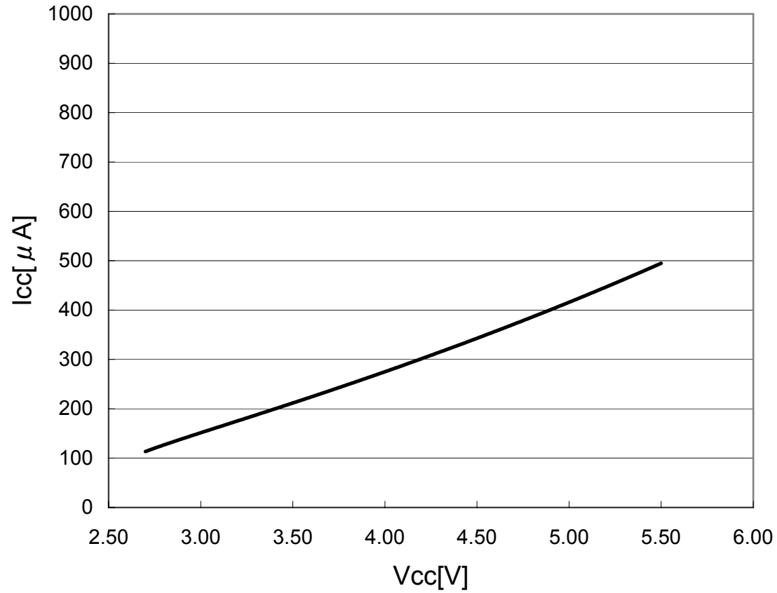
Vcc-Icc(Wait Mode)
