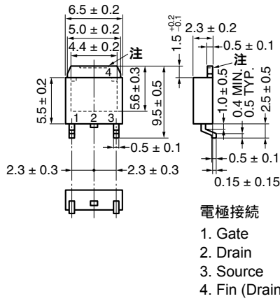
TO-252表面実装形 (MP-3Z)
