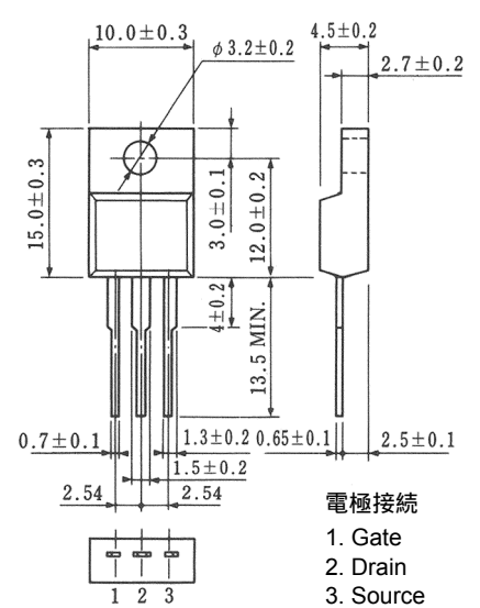
TO-220絶縁形 (MP-45F)
