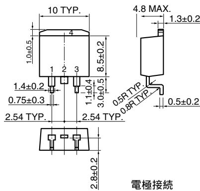
TO-220AB表面実装形 (MP-25Z)
