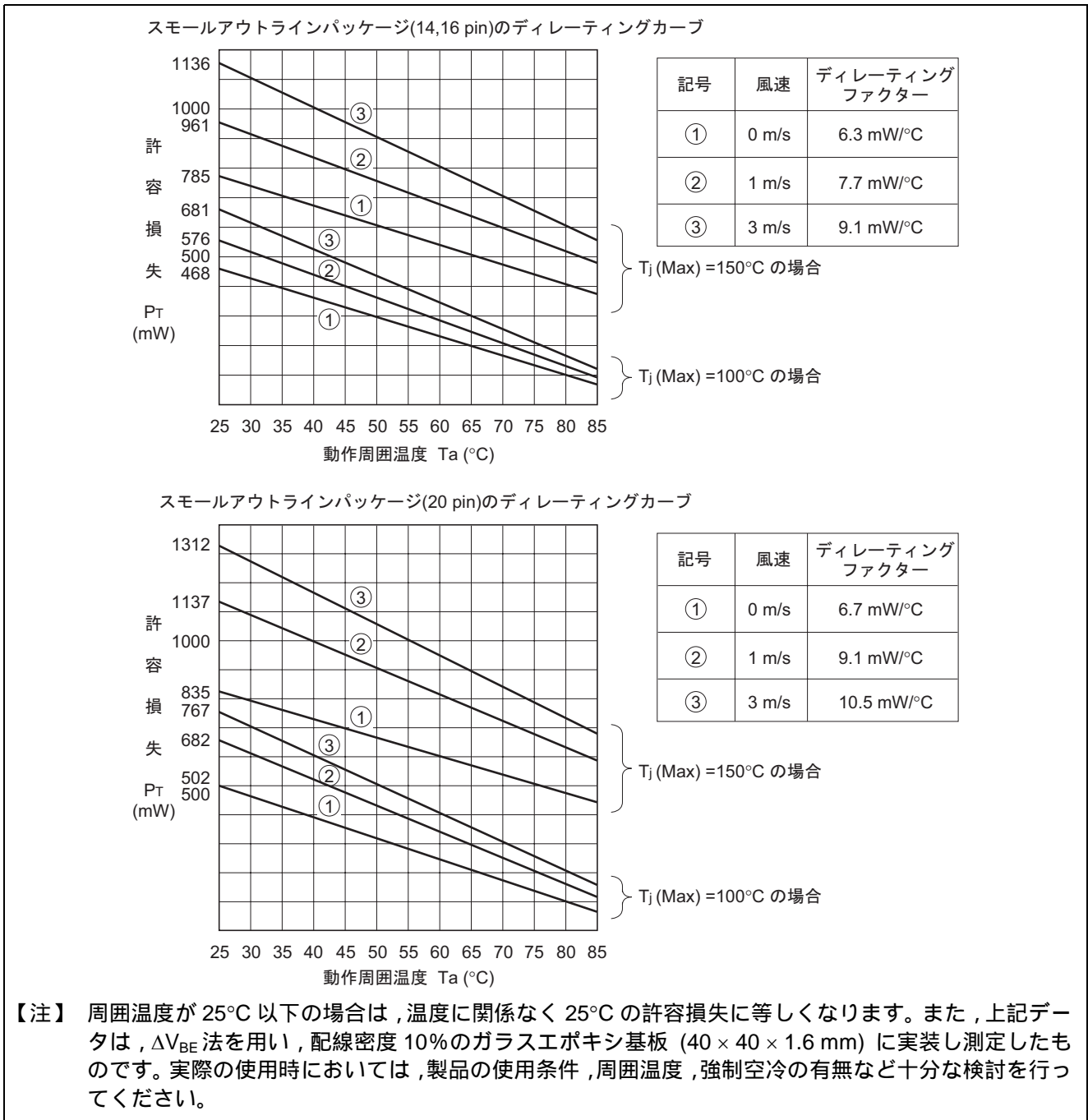
図 1 SOP のディレーティングカーブ
