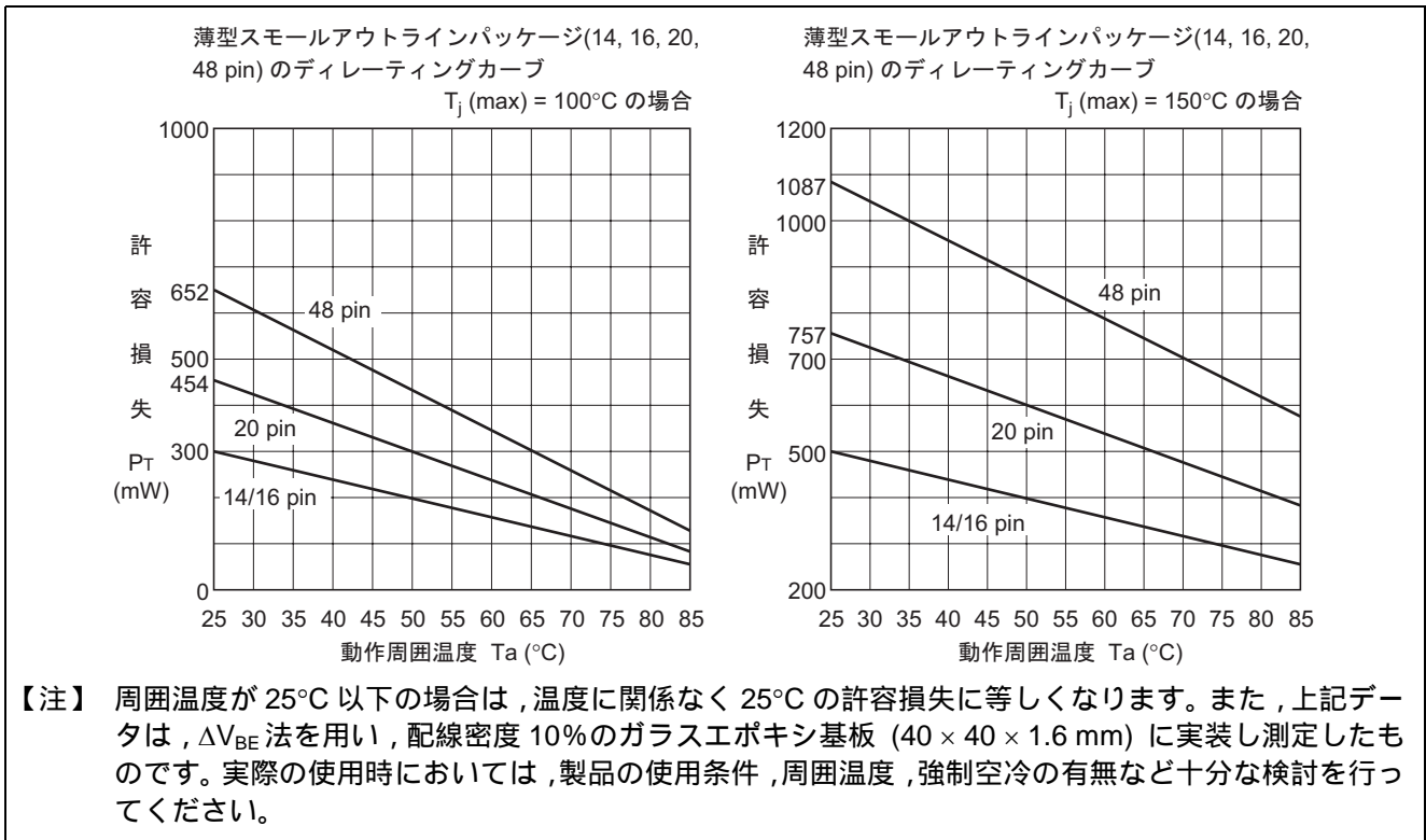
図2 TSSOP のディレーティングカーブ
