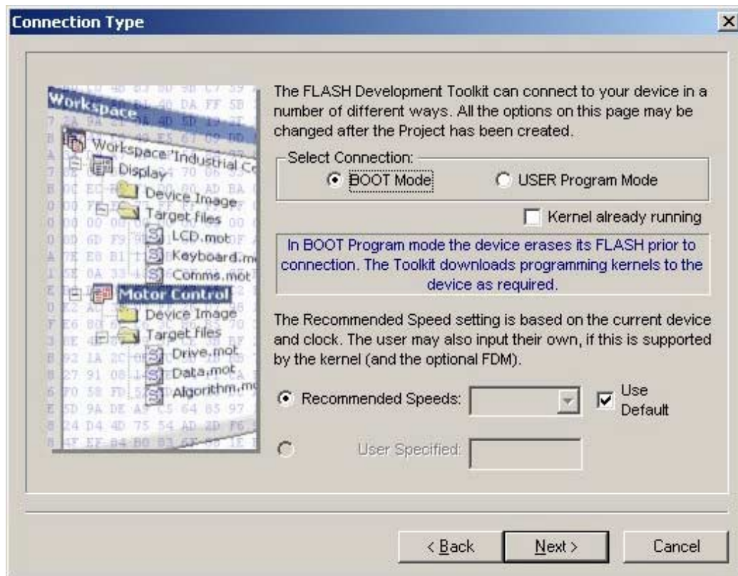
図 3-6 接続の種類
