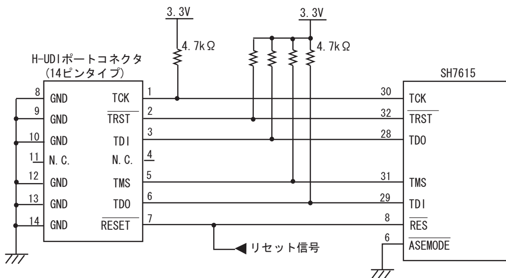
図 1.2 E10A 使用時の H-UDI ポートコネクタ - チップ間の推奨接続例(14 ピンタイプ)
