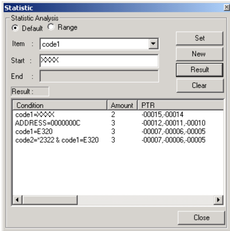
図 5-32 Trace Statistic ダイアログボックス
