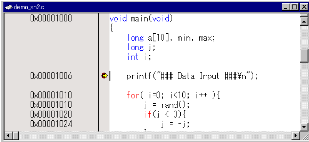
図 5-23 Source ウィンドウと address カラム
