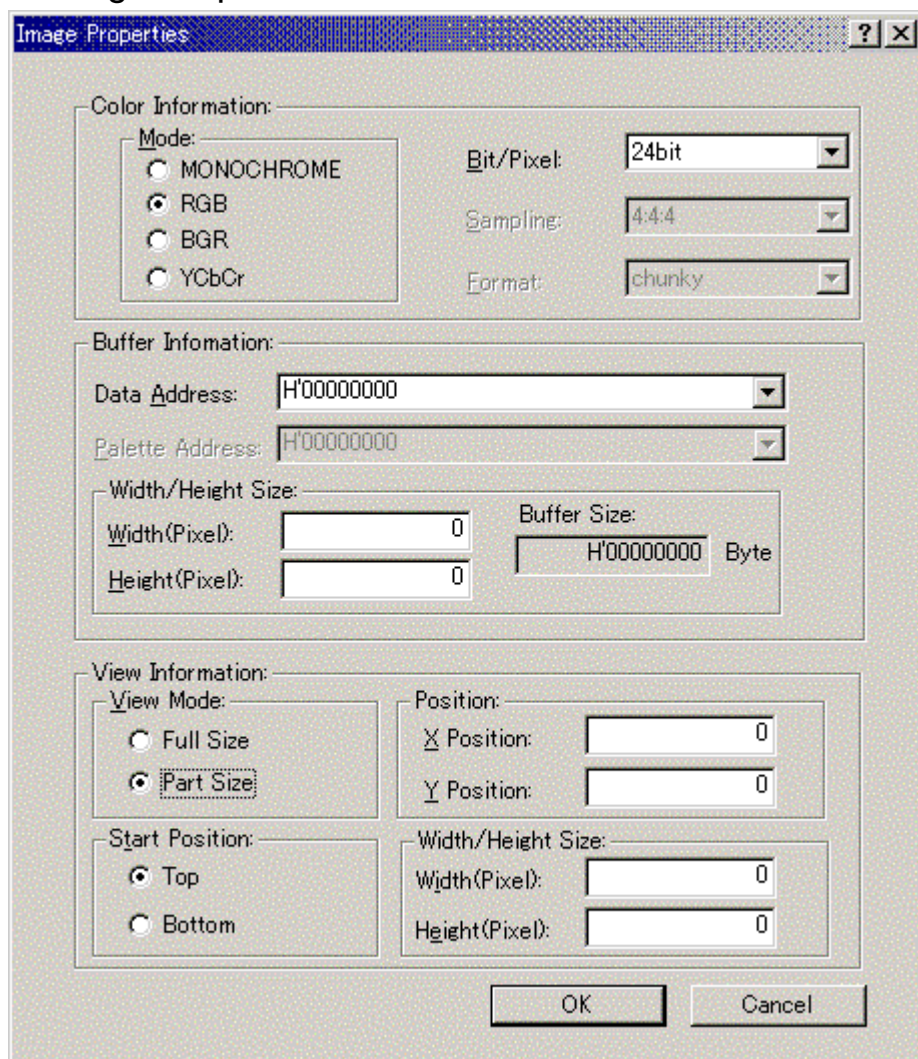
図 5-73 Image Properties ダイアログボックス
