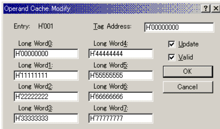
図 5-63 Operand Cache Modify ダイアログボックス (SH-4/SH-4BSC)
