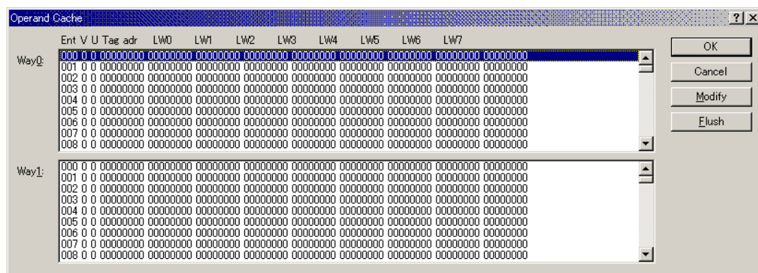
図 5-62 Operand Cache ダイアログボックス (SH-4 (SH7750R))
