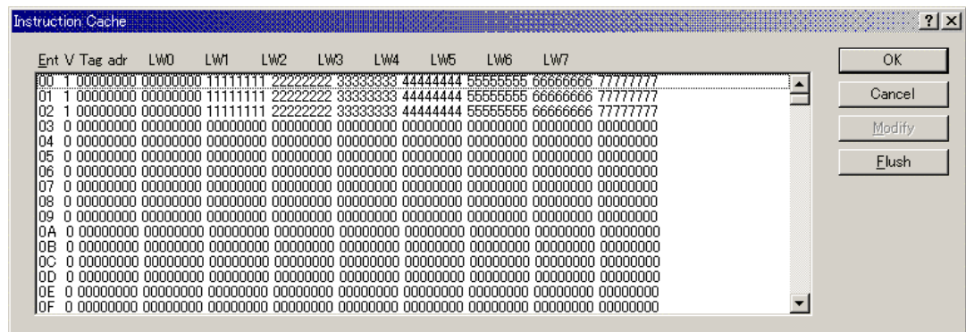
図 5-57 Instruction Cache ダイアログボックス (SH-4/SH-4BSC)
