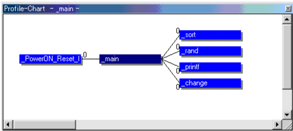
図 5-71 Profile-Chart ウィンドウ
