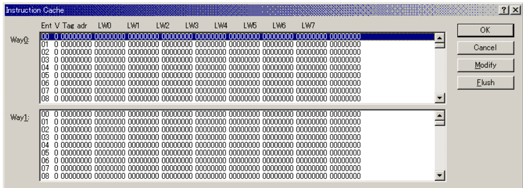
図 5-58 Instruction Cache ダイアログボックス ( SH-4 ( SH7750R ) )
