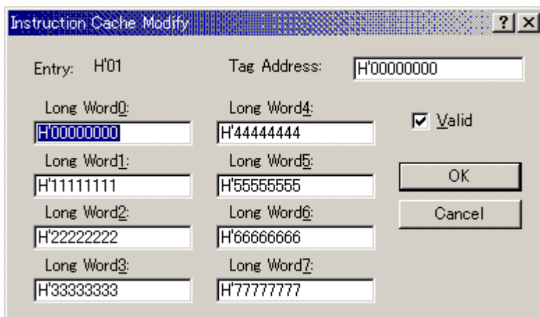
図 5-59 Instruction Cache Modify ダイアログボックス (SH-4/SH-4BSC)
