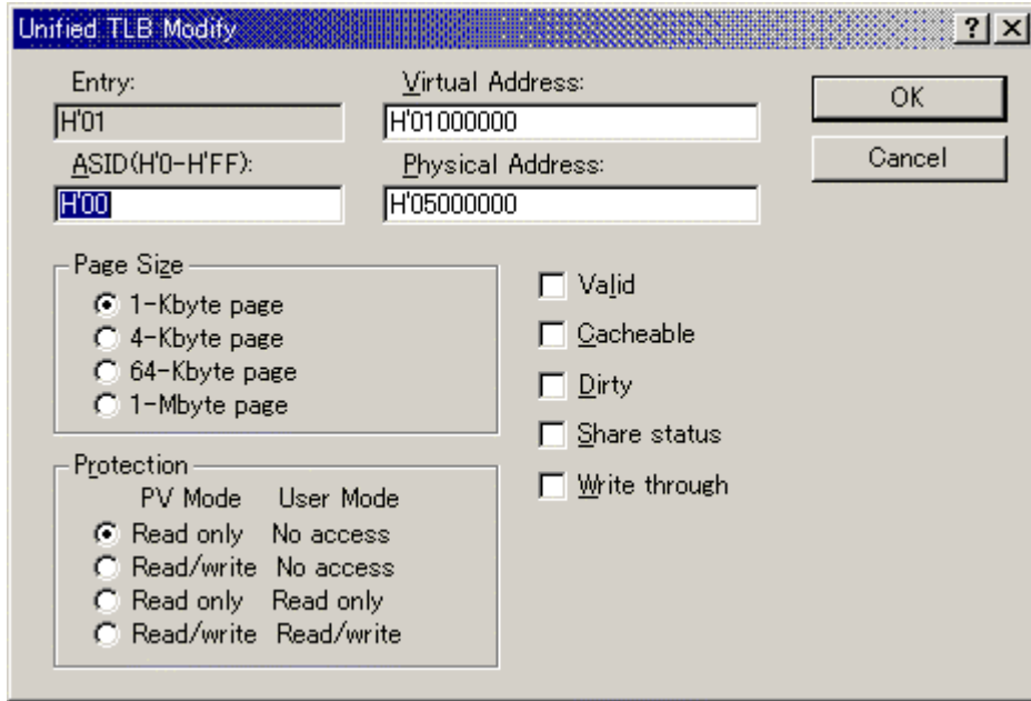
図 5-52 Unified TLB Modify ダイアログボックス
