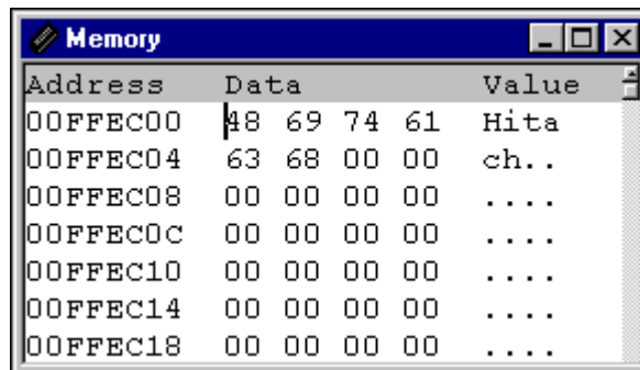
図 5-17 Memory ウィンドウ
