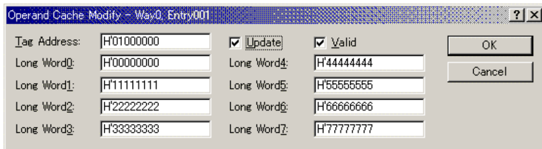
図 5-64 Operand Cache Modify ダイアログボックス ( SH-4 ( SH7750R ) )
