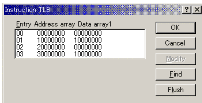
図 5-48 Instruction TLB ダイアログボックス
