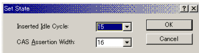
図 5-39 Set State ダイアログボックス (DRAM)
