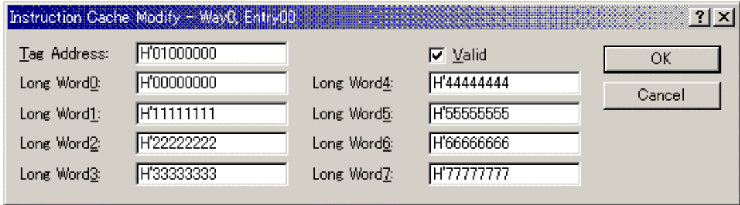
図 5-60 Instruction Cache Modify ダイアログボックス ( SH-4 ( SH7750R ) )
