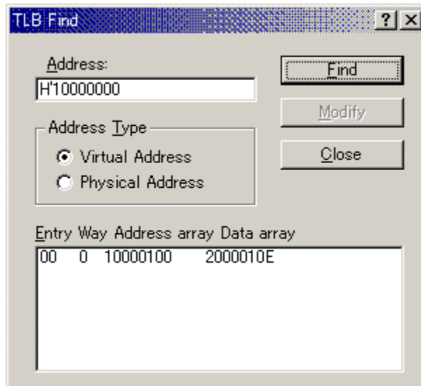
図 5-46 TLB Find ダイアログボックス
