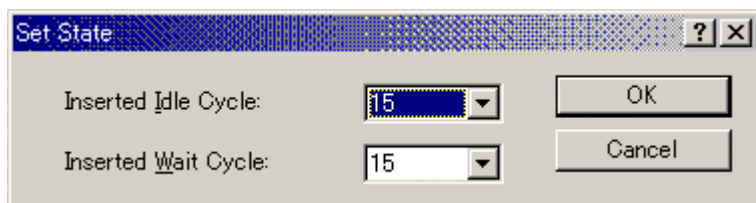
図 5-38 Set State ダイアログボックス (通常メモリ)
