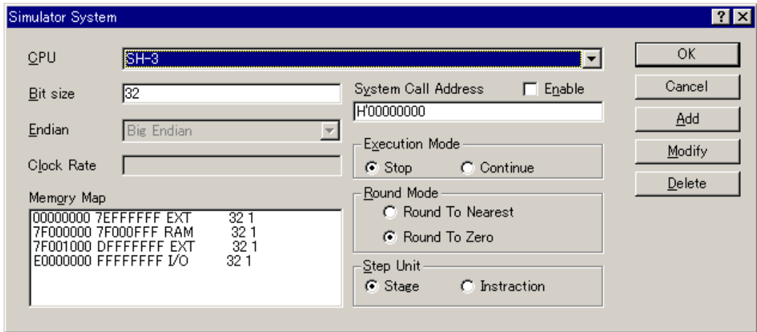
図 5-36 Simulator System ダイアログボックス
