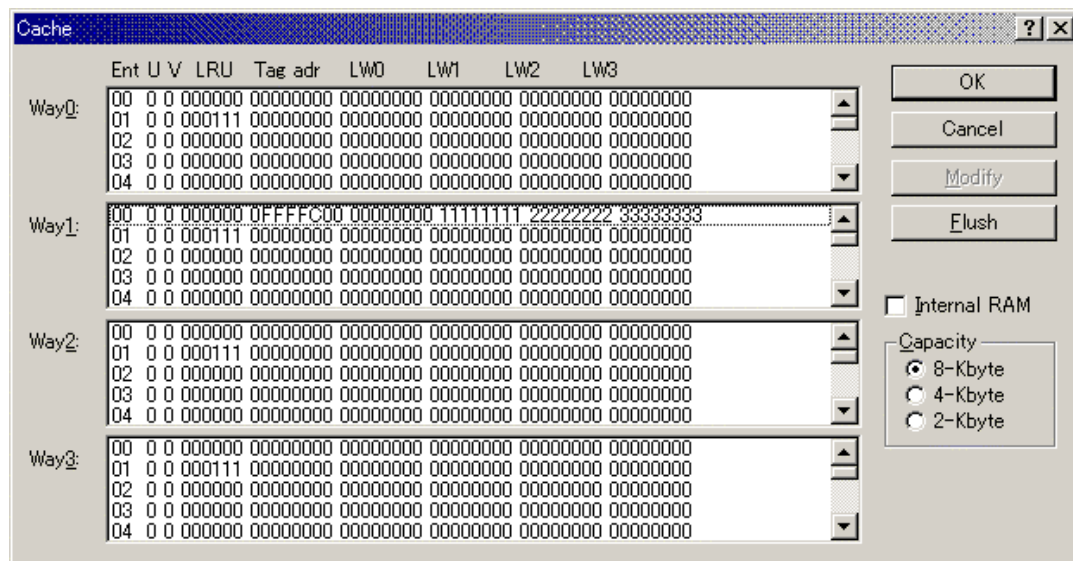
図 5-54 Cache ダイアログボックス (SH-3/SH-3E シリーズ)
