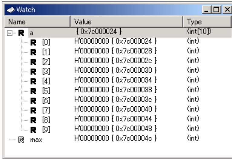
図 5-35 Watch ウィンドウ
