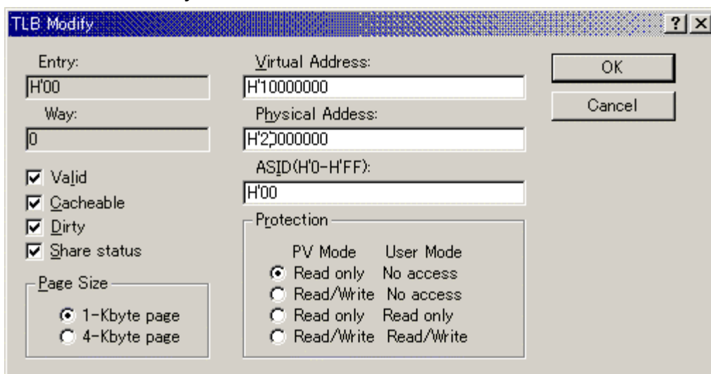
図 5-45 TLB Modify ダイアログボックス
