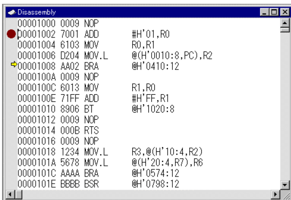
図 5-7 Disassembly ウィンドウ
