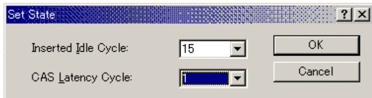
図 5-40 Set State ダイアログボックス (SDRAM)
