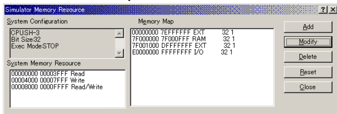
図 5-42 Simulator Memory Resource ダイアログボックス
