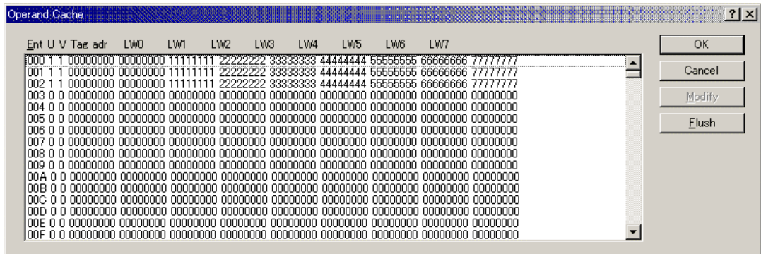
図 5-61 Operand Cache ダイアログボックス ( SH-4/SH-4BSC )
