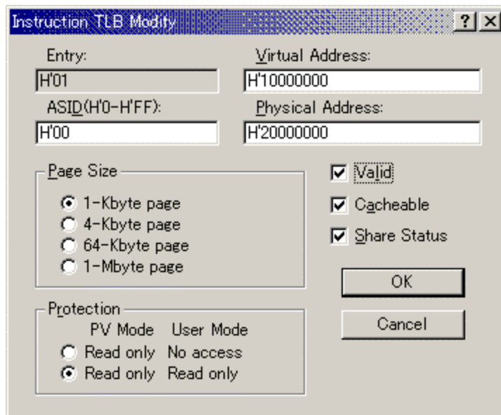
図 5-49 Instruction TLB Modify ダイアログボックス
