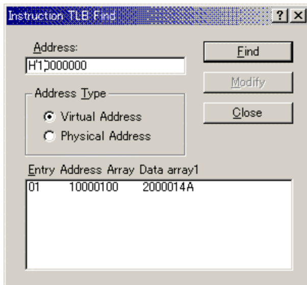
図 5-50 Instruction TLB Find ダイアログボックス
