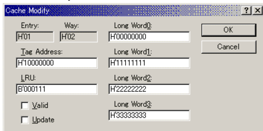
図 5-55 Cache Modify ダイアログボックス
