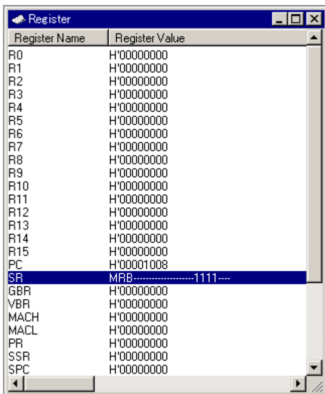
図 5-20 Registers ウィンドウ
