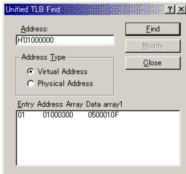
図 5-53 Unified TLB Find ダイアログボックス
