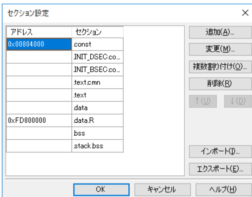
図 4-21 サブプロジェクトの設定(PE2)
