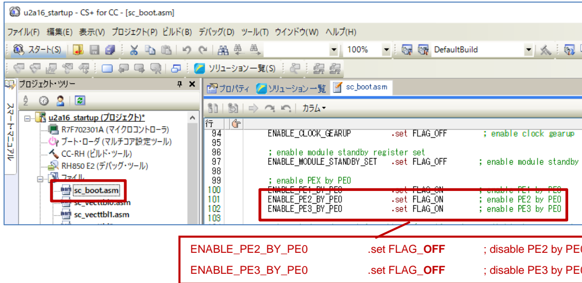
図 4-16 sc_boot.asm の修正
