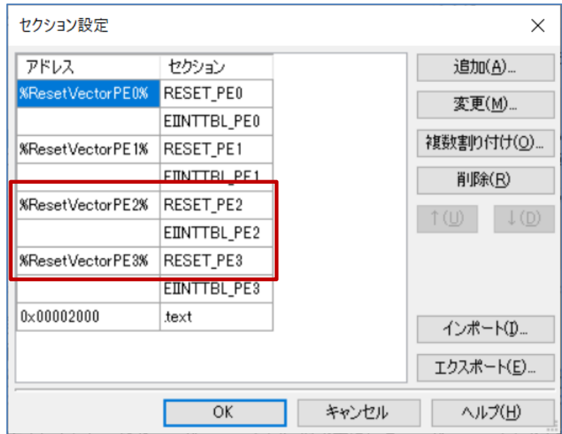
(α) 変更前
