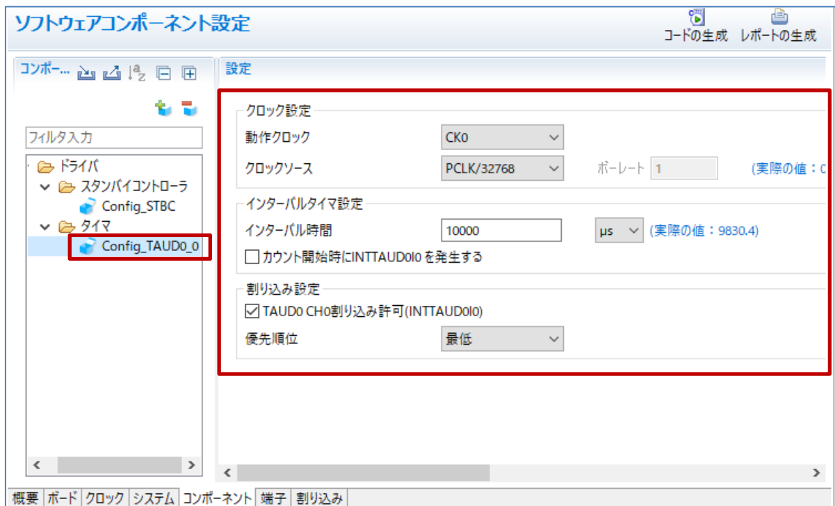
図 5-5 コンポーネントの設定
