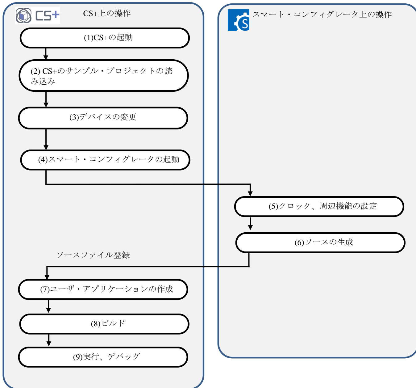
図 4-3 サンプル・プロジェクト 操作フロー
