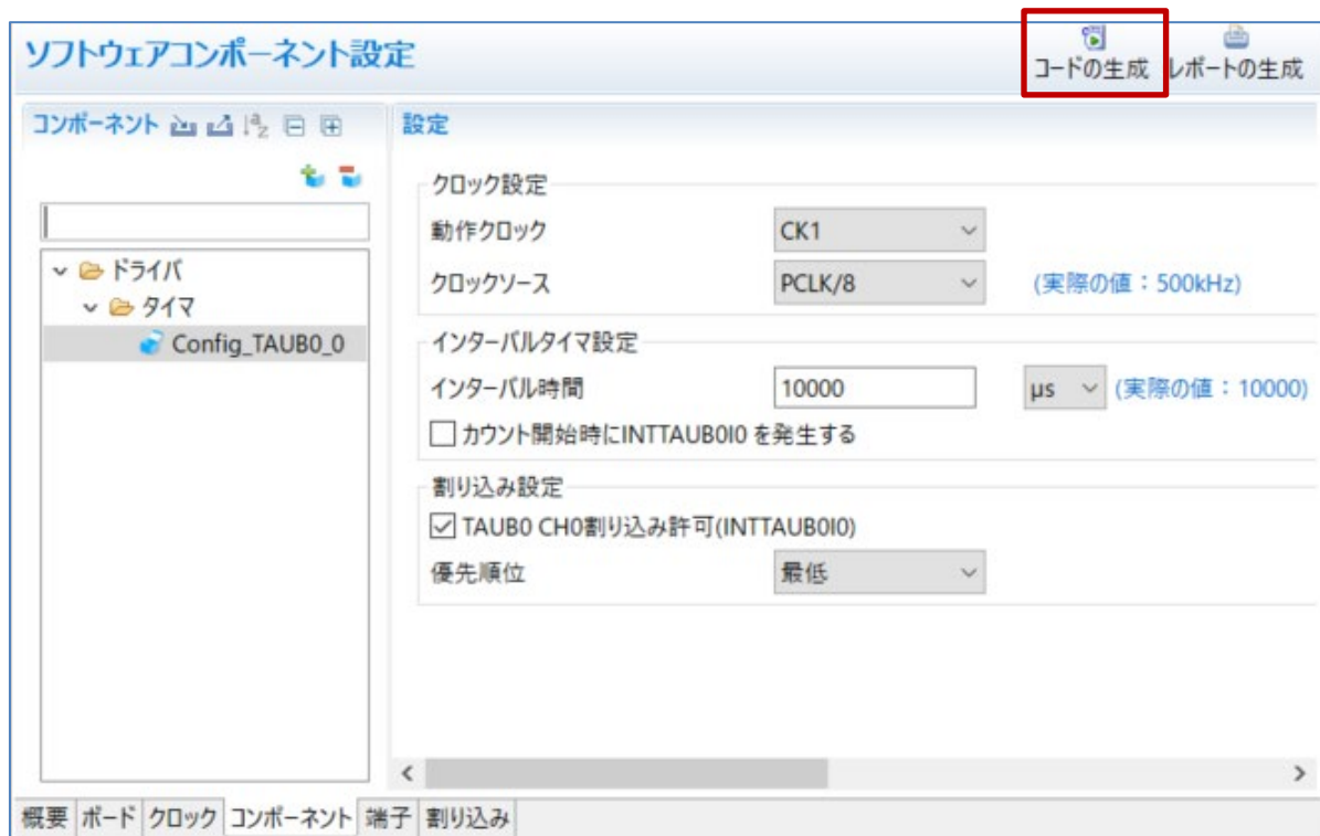
図 5-6 コード生成
