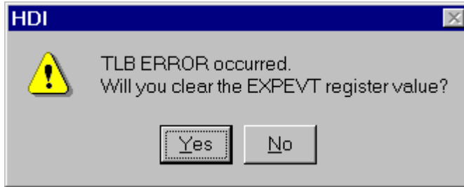
図 5.1 TLB エラーのメッセージボックス
