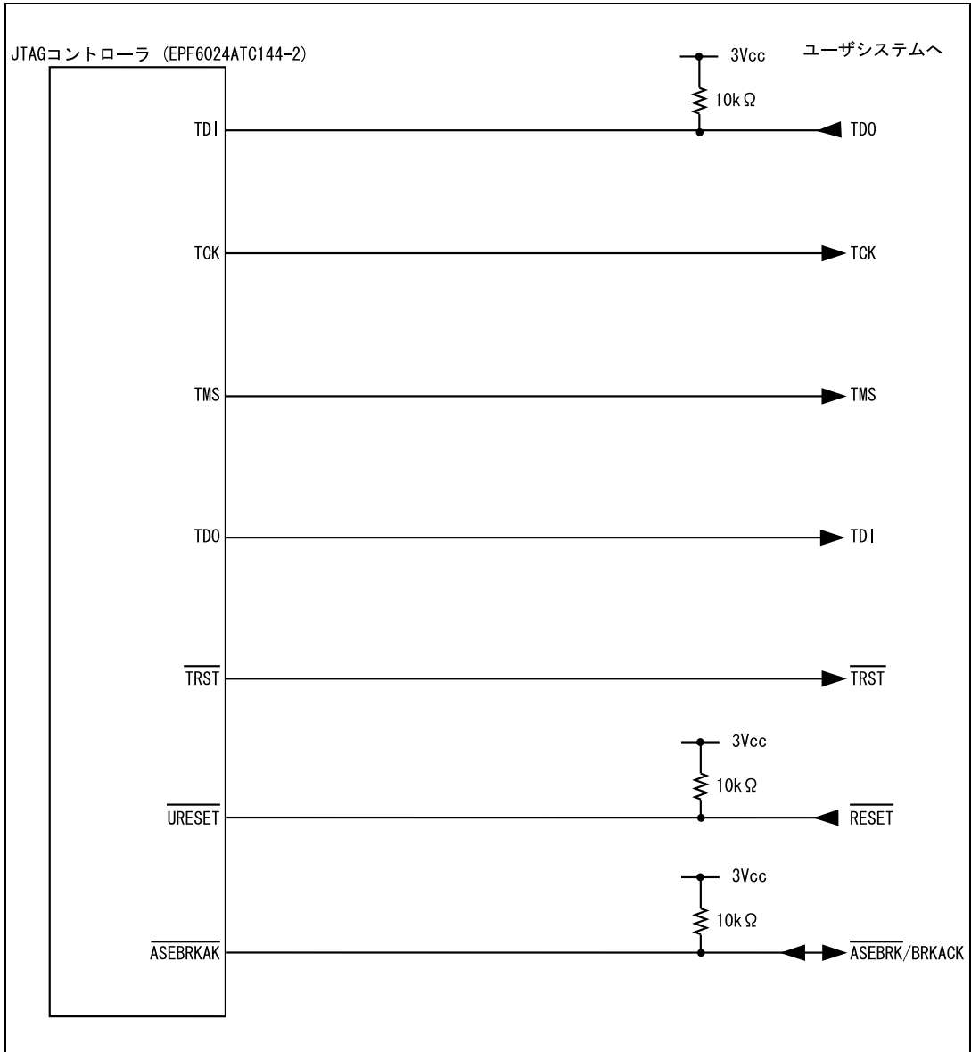
図 6.5 Hitachi-UDI 端子部分のユーザシステムインタフェース回路 (HS7760KCM02H) (Model 名 : HS0005KCM04H)
