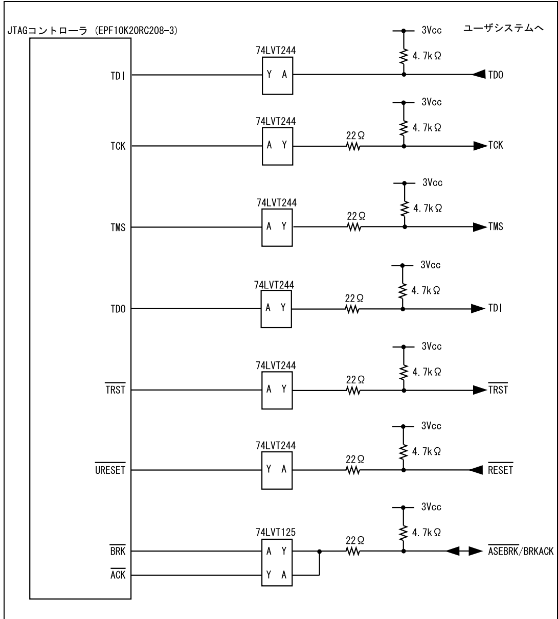
図 6.7 ユーザシステムインタフェース回路 (HS7760KCI01H) (Model名: HS0005KCI03H)
