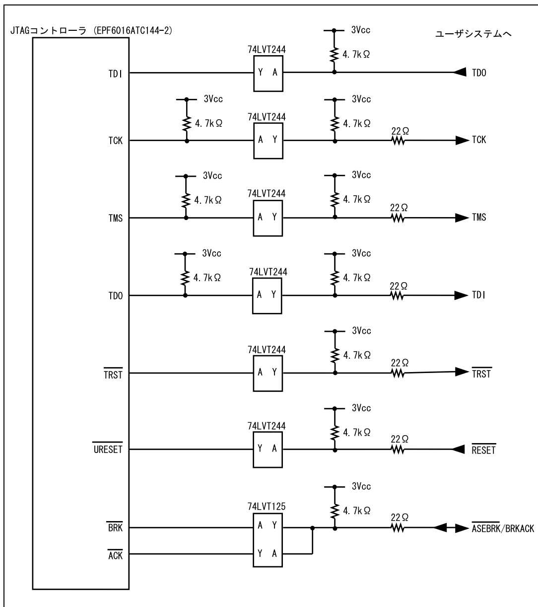
図 6.4 ユーザシステムインタフェース回路 (HS7760KCM01H) (Model 名 : HS0005KCM03H)
