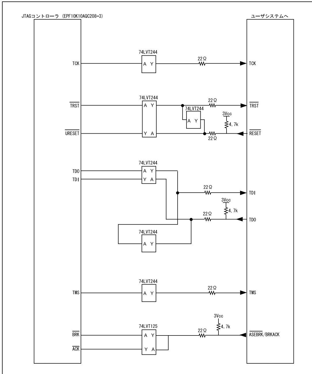
図 6.8 Hitachi-UDI 端子部分のユーザシステムインタフェース回路 (HS7760KCI02H) ( Model 名 : HS0005KCI04H )
