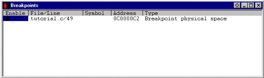
図 3.39 [ Breakpoints ] ウィンドウ (ソフトウェアブレイク設定時)
