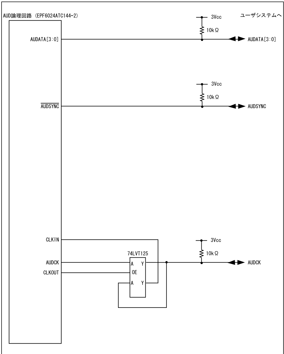
図 6.6 AUD 端子部分のユーザシステムインタフェース回路 (HS7760KCM02H) (Model 名 : HS0005KCM04H)
