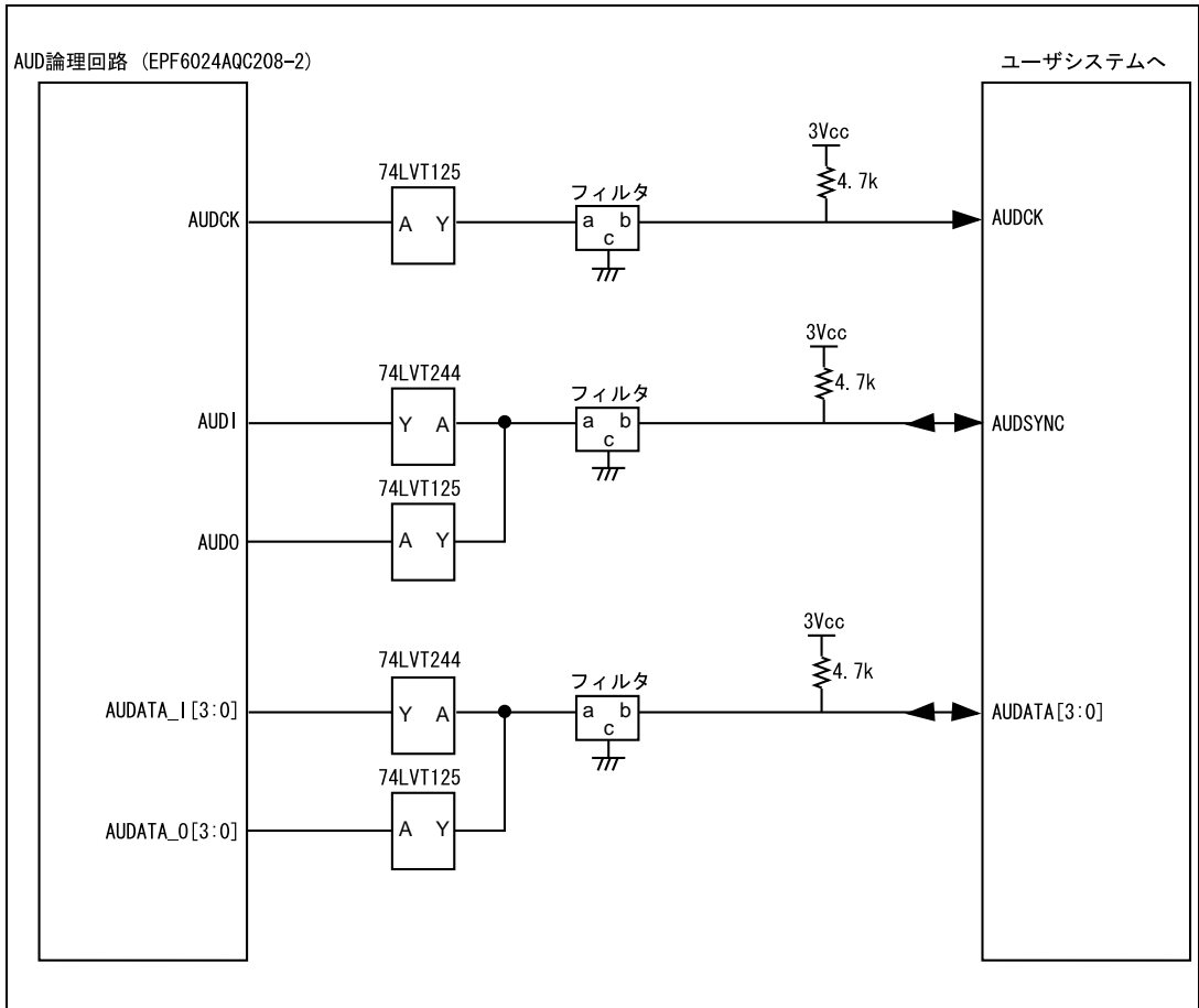
図 6.9 AUD 端子部分のユーザシステムインタフェース回路 (HS7760KCI02H) ( Model 名 : HS0005KCI04H )
