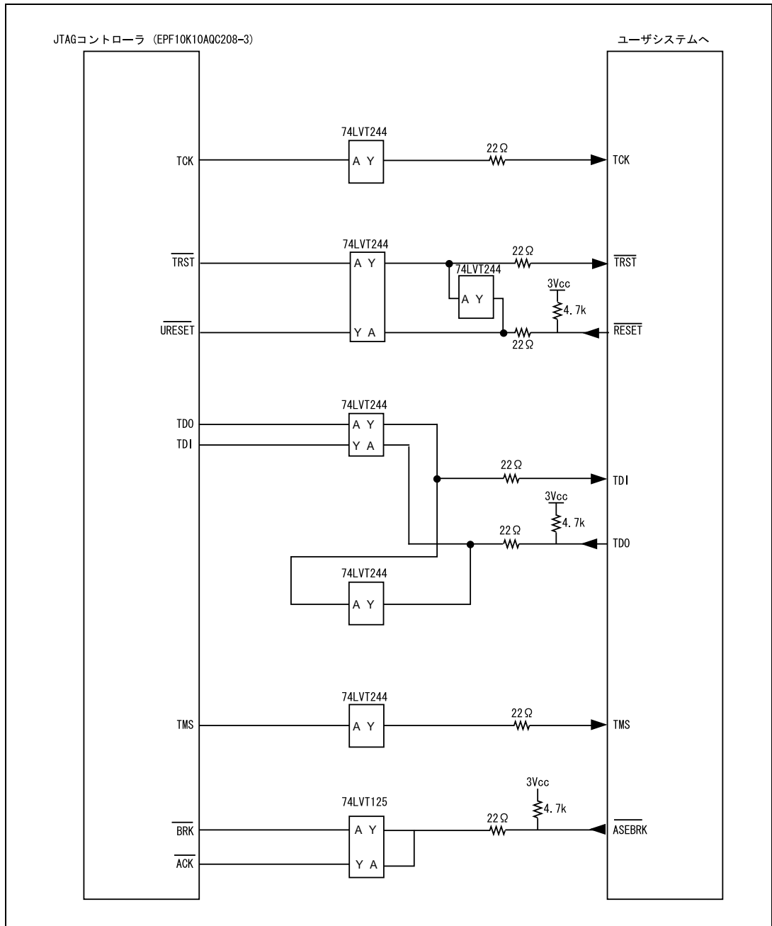
図 6.8 Hitachi-UDI 端子部分のユーザシステムインタフェース回路 (HS7751RKCI02H) (Model 名 : HS0005KCI04H)
