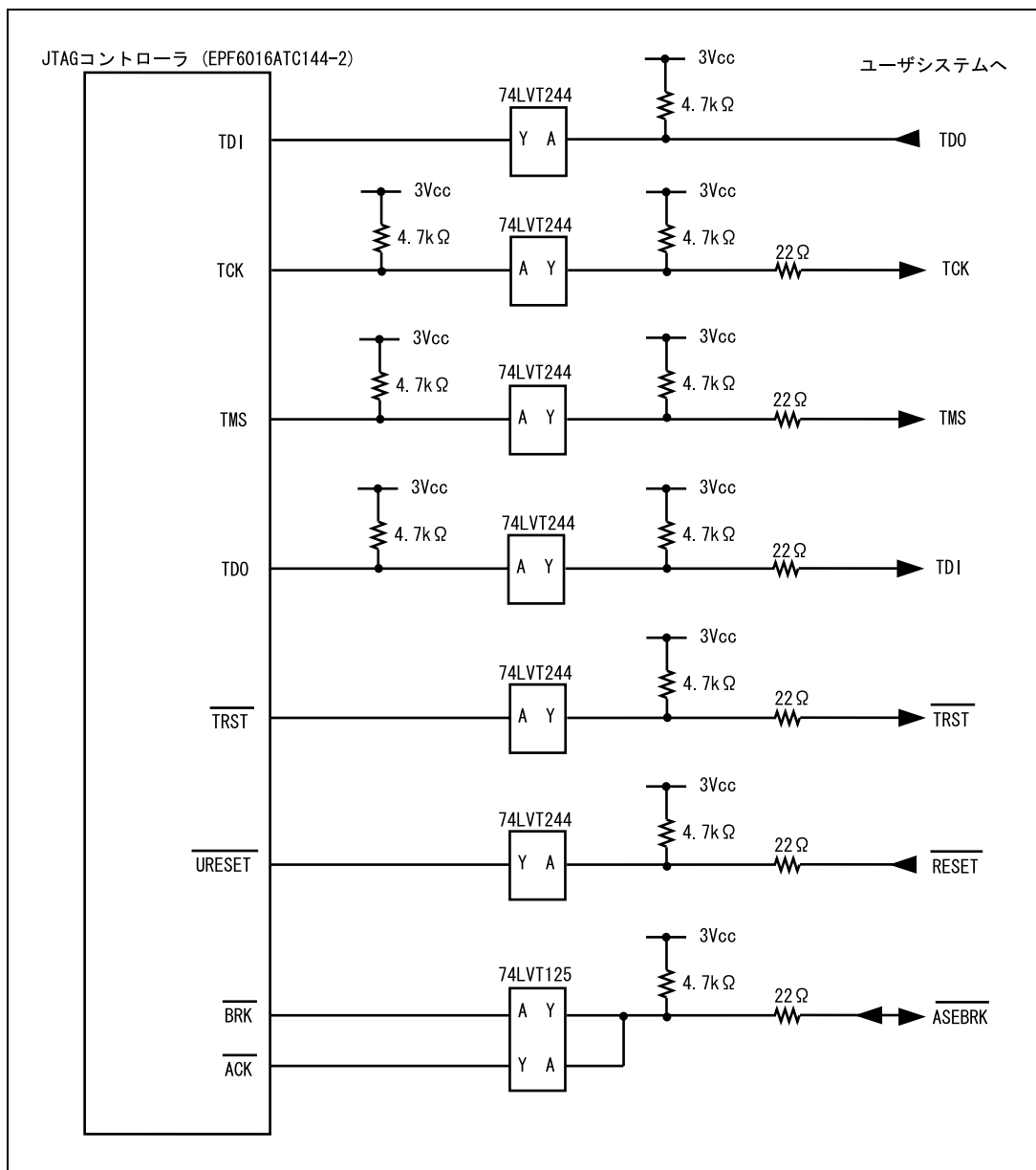
図 6.4 ユーザシステムインタフェース回路 (HS7751RKCM01H) (Model 名 : HS0005KCM03H)
