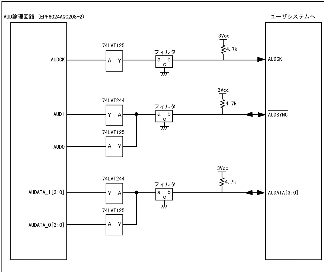
図 6.9 AUD 端子部分のユーザシステムインタフェース回路 (HS7751RKCI02H) ( Model 名 : HS0005KCI04H )
