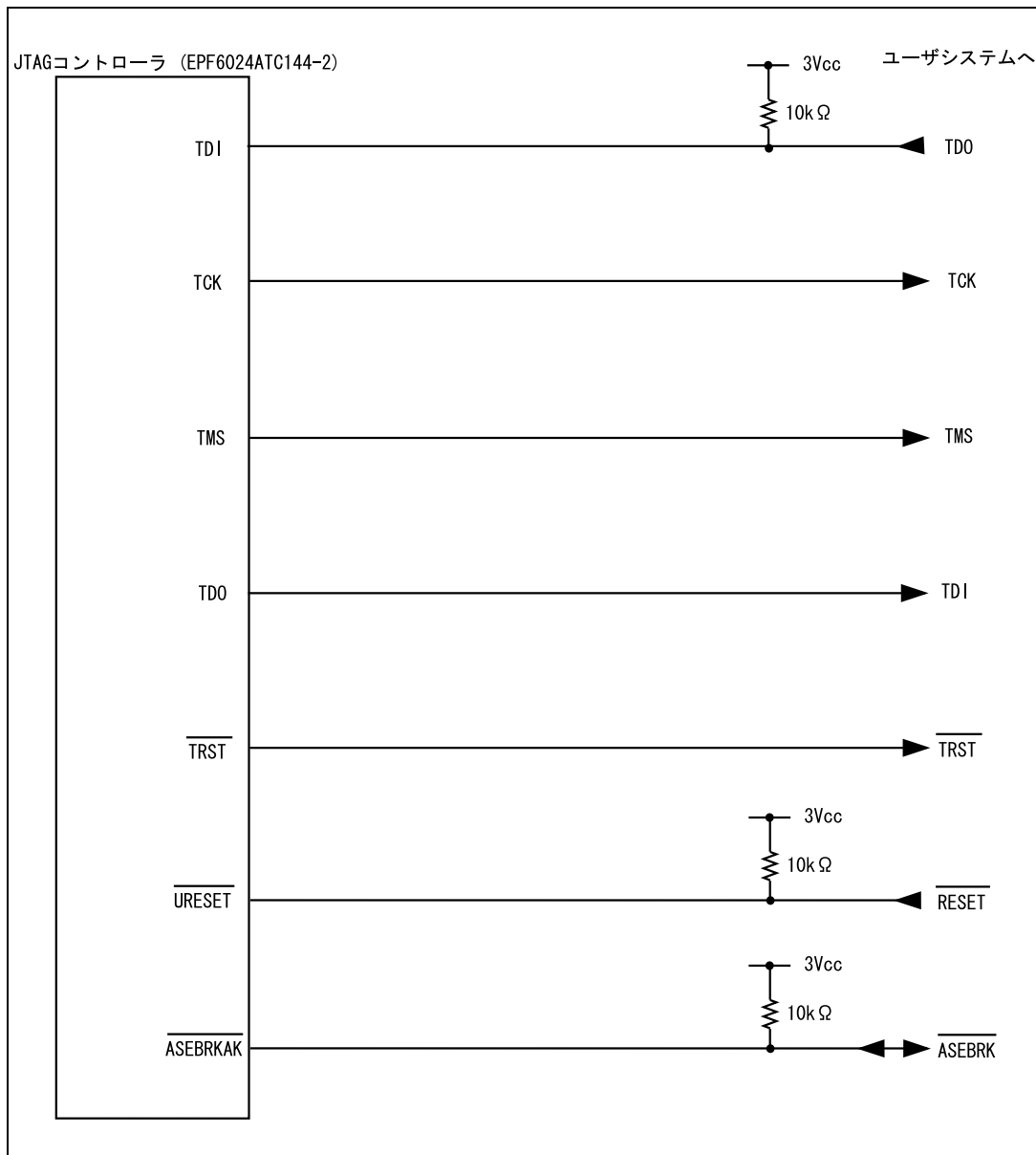
図 6.5 Hitachi-UDI 端子部分のユーザシステムインタフェース回路 (HS7751RKCM02H) (Model 名 : HS0005KCM04H)
