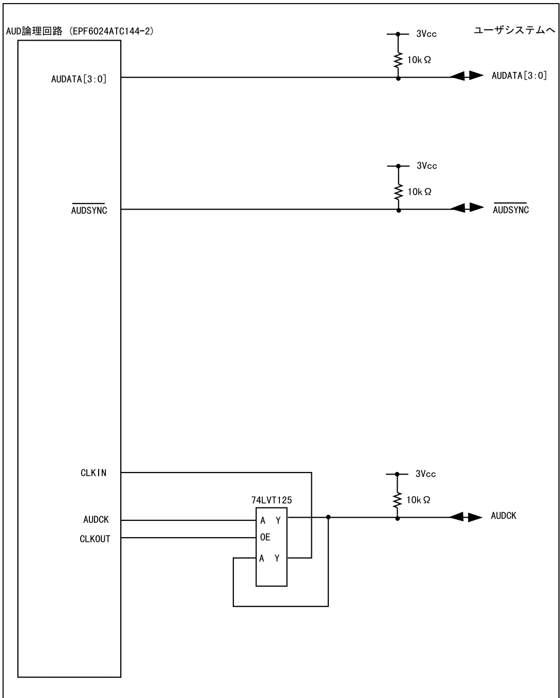
図 6.6 AUD 端子部分のユーザシステムインタフェース回路 (SH7751RKCM02H) (Model 名 : HS0005KCM04H)
