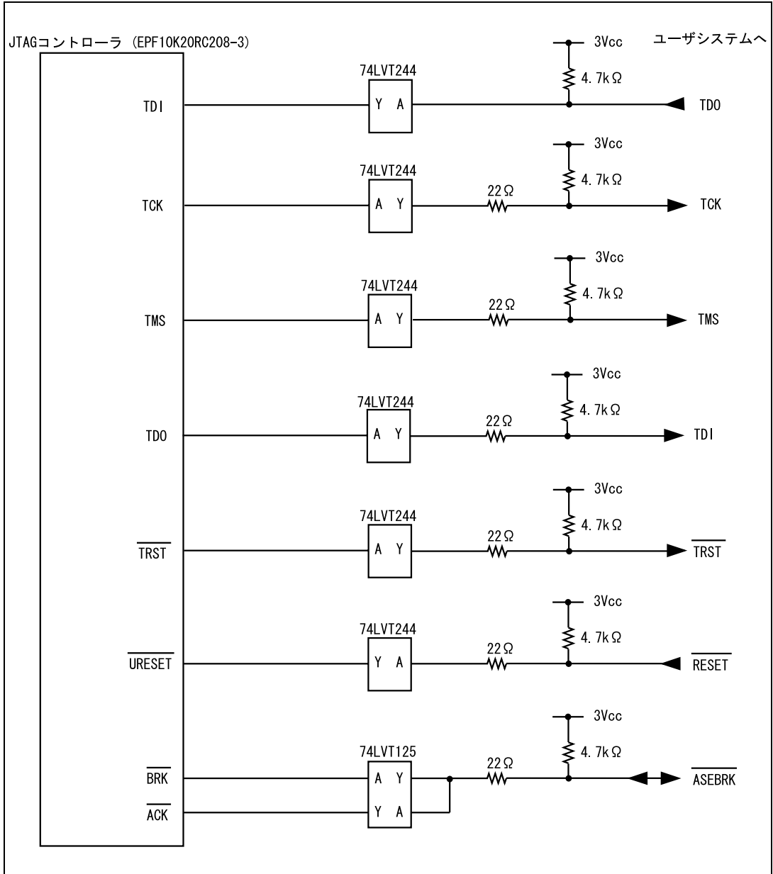
図 6.7 ユーザシステムインタフェース回路 (HS7751RKCI01H) (Model名: HS0005KCI03H)
