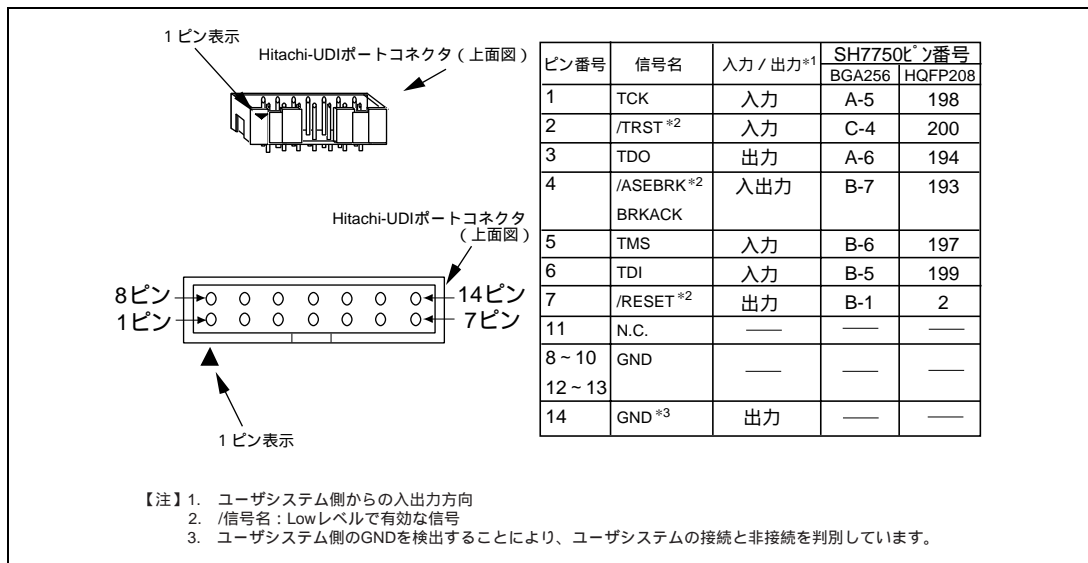
図 6.1 Hitachi-UDI ポートコネクタのピン配置
