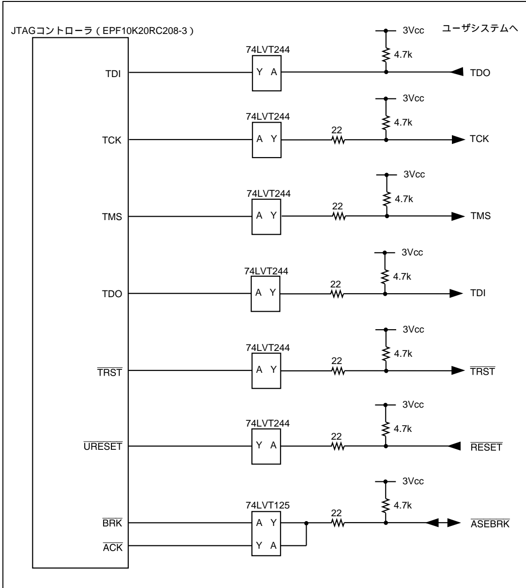
図 6.3 ユーザシステムインタフェース回路 (HS7750KCI01H) ( Model 名 : HS0005KCI03H )
