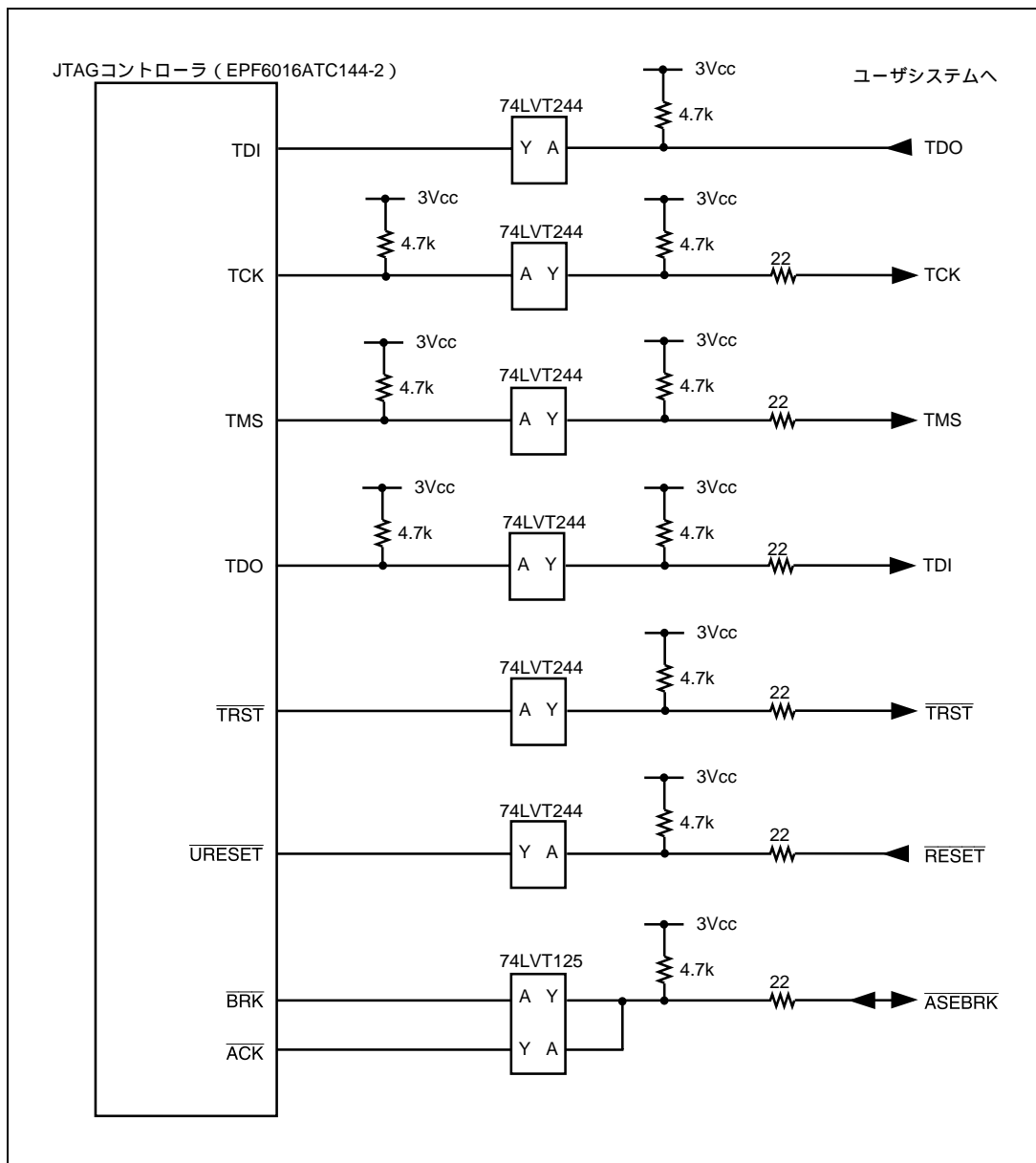
図 6.2 ユーザシステムインタフェース回路 (HS7750KCM01H) (Model 名 : HS0005KCM03H)
