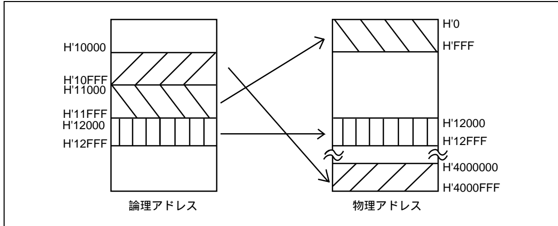
図 3.58 VP_MAP テーブルによるアドレス変換
