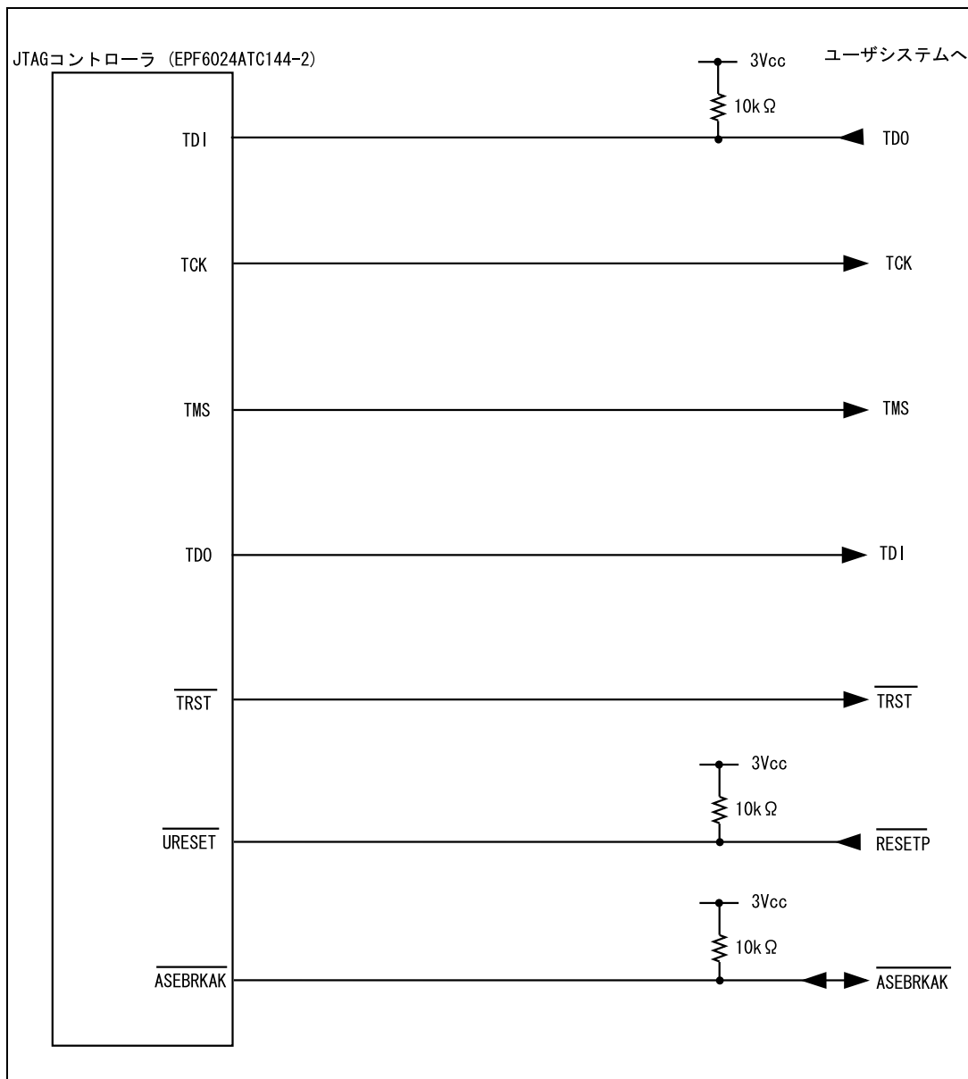
図 6.5 Hitachi-UDI 端子部分のユーザシステムインタフェース回路 (HS7729RKCM02H) (Model 名: HS0005KCM02H)
