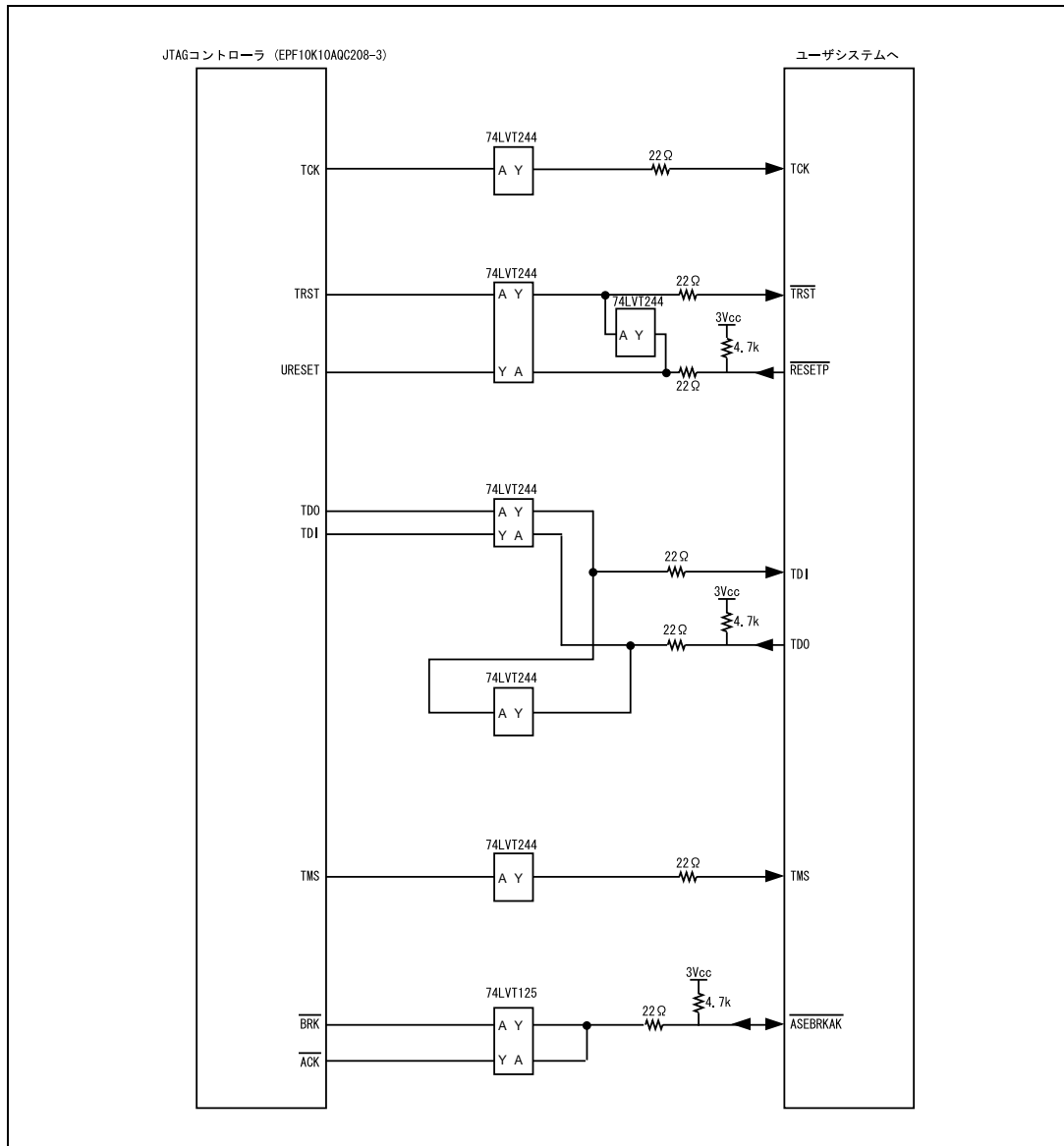
図 6.8 Hitachi-UDI 端子部分のユーザシステムインタフェース回路 (HS7729RKC102H) (Model 名 : HS0005KC104H)
