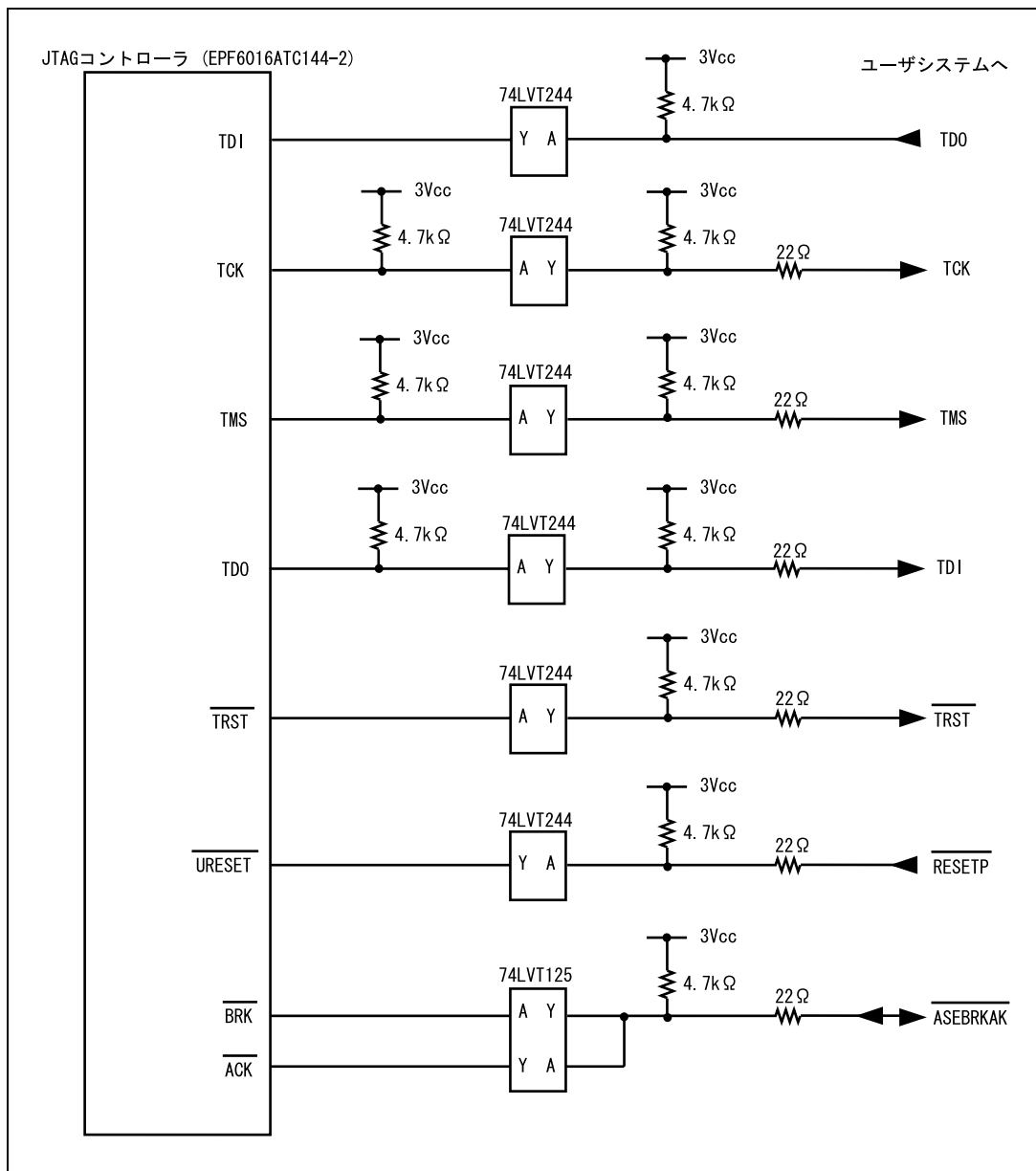
図 6.4 ユーザシステムインタフェース回路 ( HS7729RKCM01H ) ( Model 名 : HS0005KCM03H )
