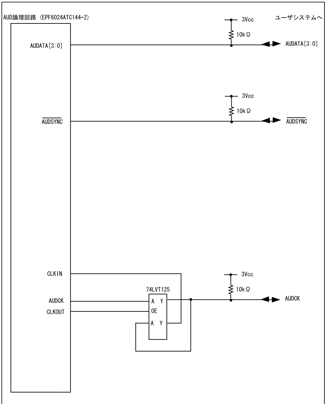
図 6.6 AUD 端子部分のユーザシステムインタフェース回路 (HS7729RKCM02H) (Model 名 : HS0005KCM02H)
