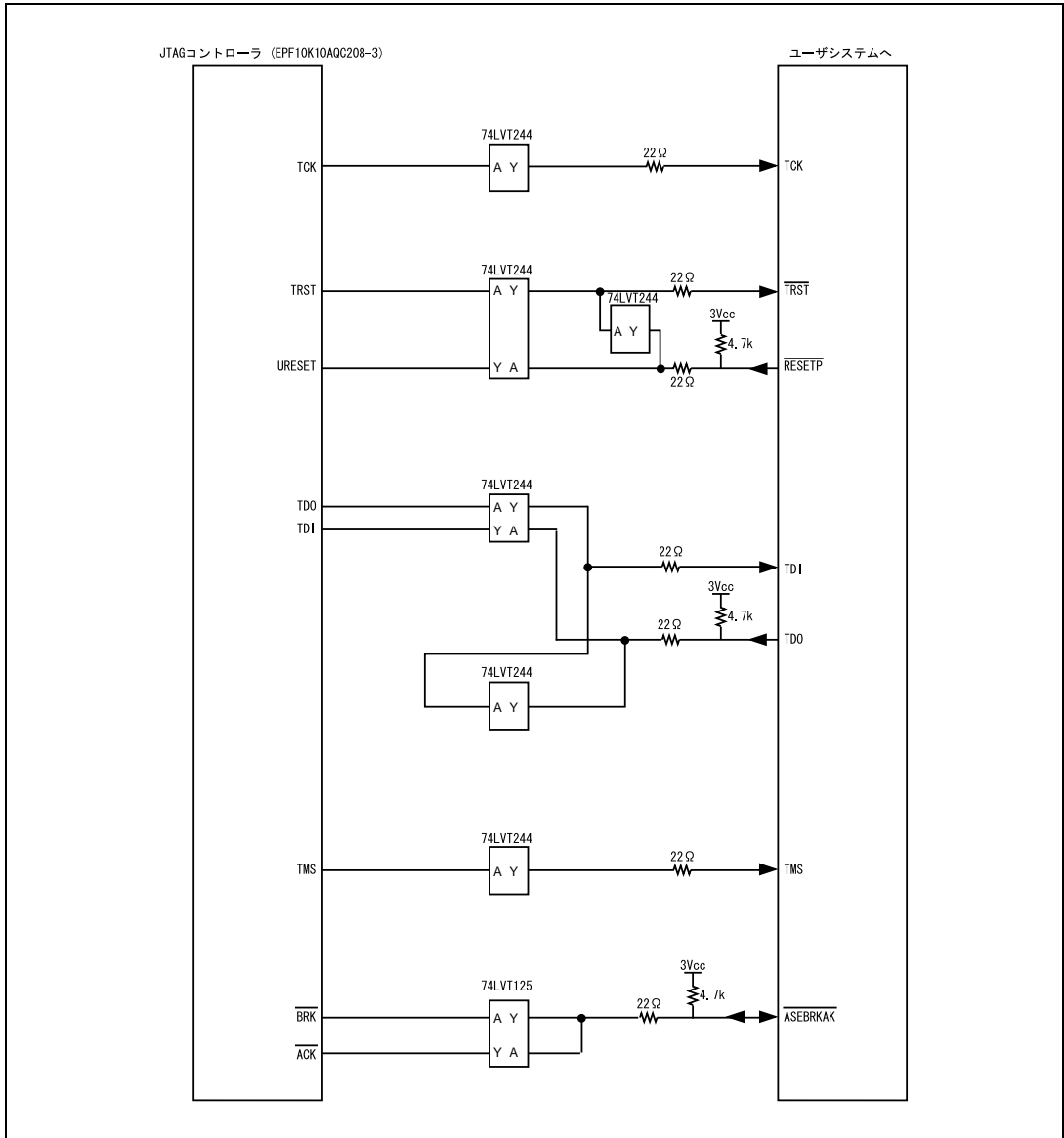
図 6.8 Hitachi-UDI 端子部分のユーザシステムインタフェース回路 (HS7706KCI02H) ( Model 名 : HS0005KCI04H )
