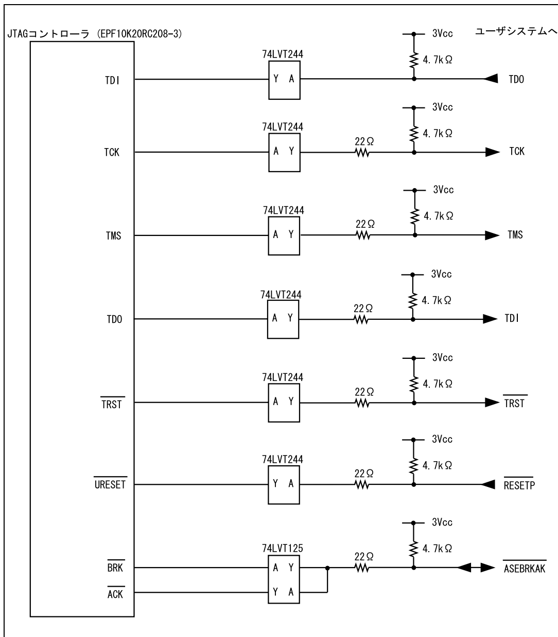
図 6.7 ユーザシステムインタフェース回路 (HS7706KCI01H) ( Model 名 : HS0005KCI03H )
