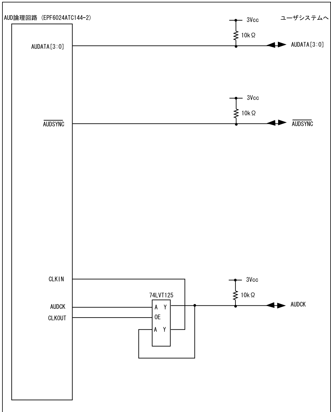
図 6.6 AUD 端子部分のユーザシステムインタフェース回路 (HS7706KCM02H) (Model 名 : HS0005KCM02H)
