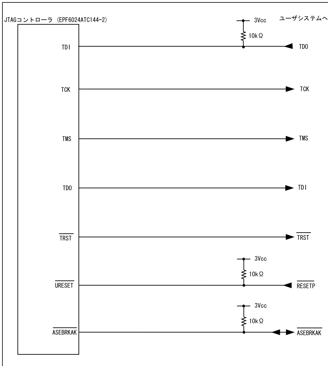
図 6.5 Hitachi-UDI 端子部分のユーザシステムインタフェース回路 (HS7706KCM02H) ( Model 名 : HS0005KCM02H )
