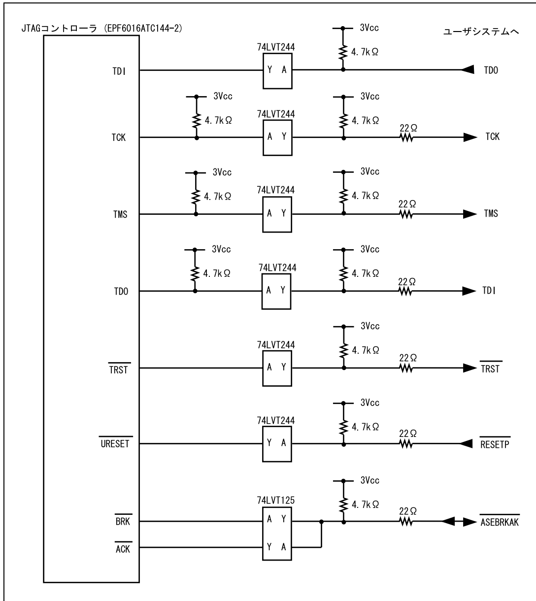
図 6.4 ユーザシステムインタフェース回路 (HS7706KCM01H) (Model 名 : HS0005KCM03H)
