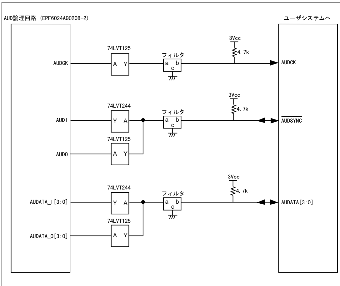
図 6.9 AUD 端子部分のユーザシステムインタフェース回路 (HS7706KCI02H) ( Model 名 : HS0005KCI04H )
