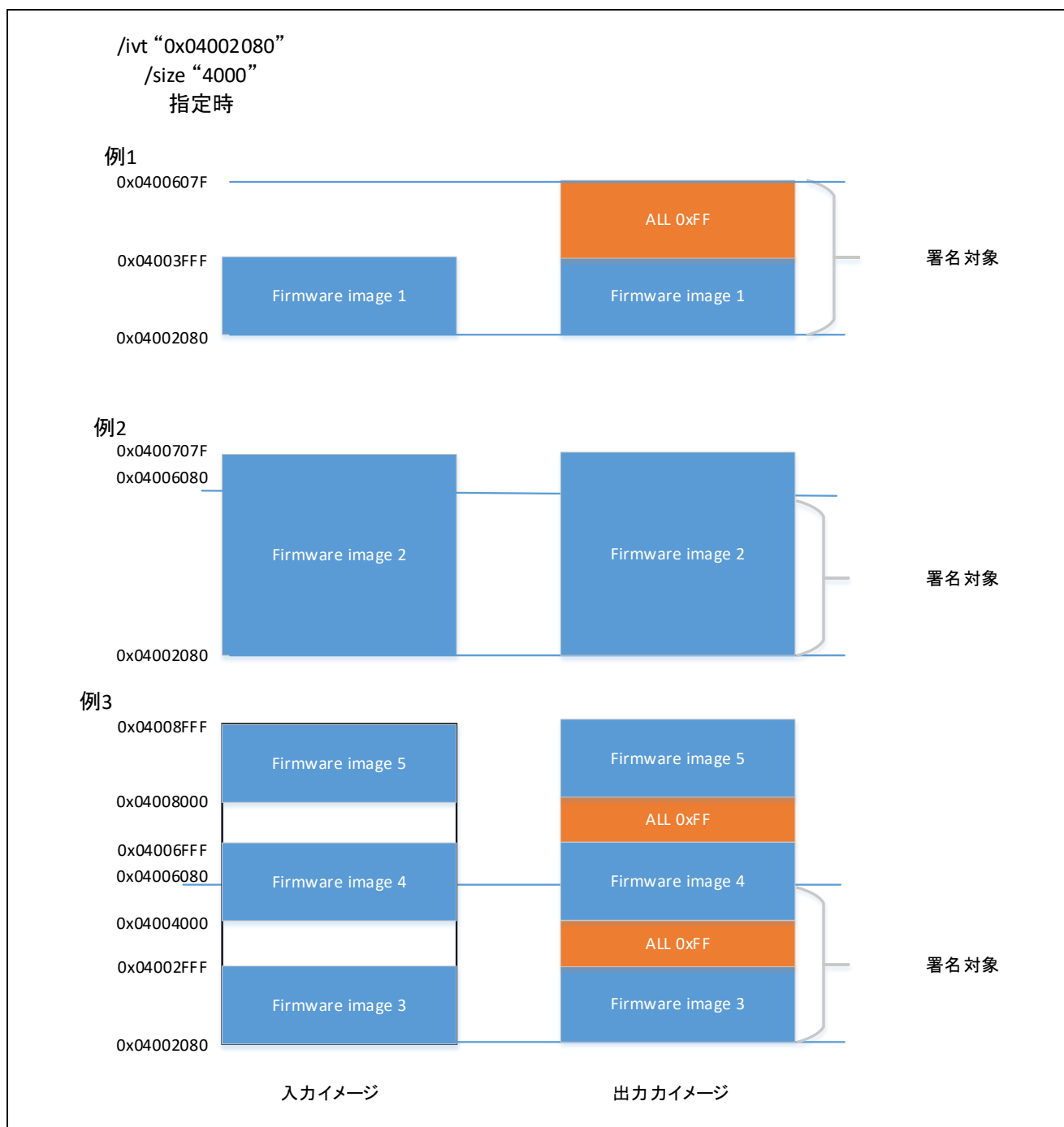
図 4.11 入力されるファームウェアイメージに Motorola Hex ファイル指定時に size オプションを指定した場合の署名対象と出力イメージ
