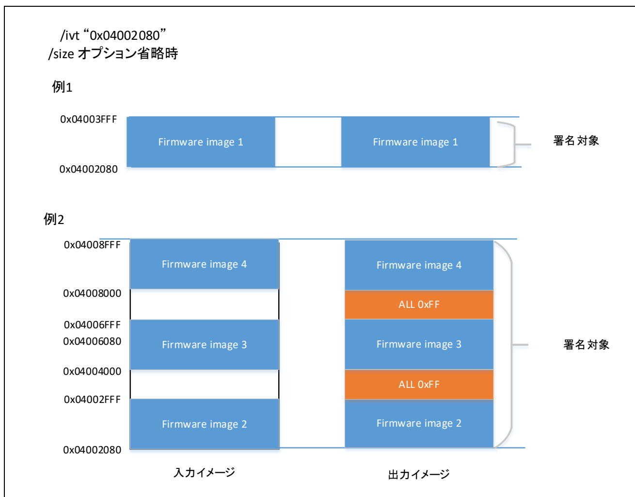
図 4.10 入力されるファームウェアイメージに Motorola Hex ファイル指定時に size オプションを省略した場合の署名対象と出力イメージ
