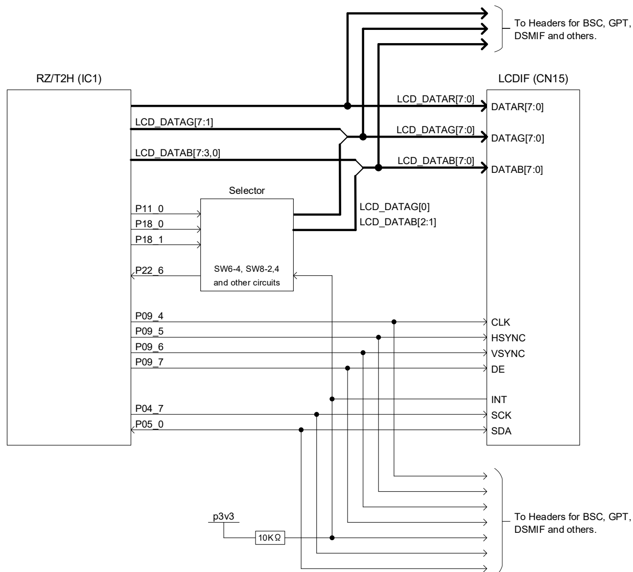
図 7-25 LCD インタフェース回路構成
