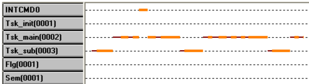
図 A—8 実行遷移図 (簡易モード)
