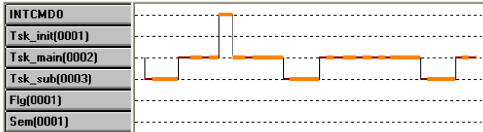
図A—9 実行遷移図（標準モード）
