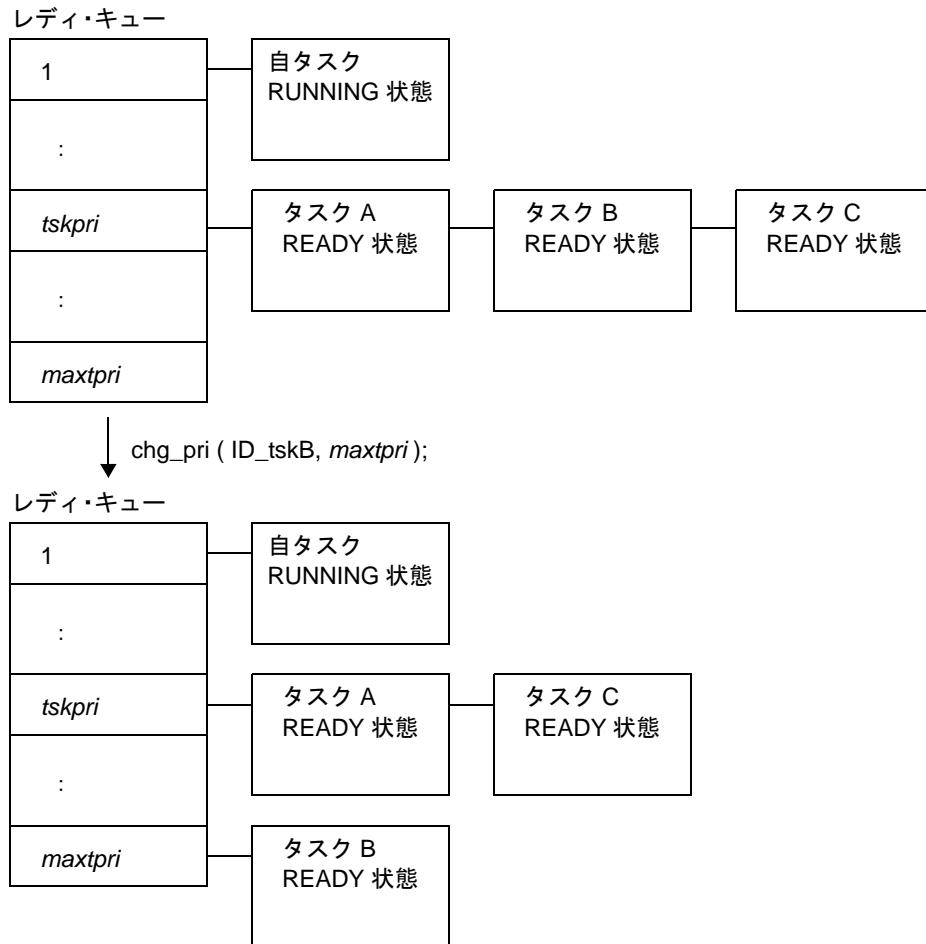
図 11 - 3 優先度の変更
