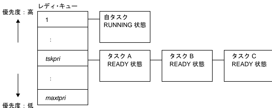
図 11 - 1 スケジューリング方式 (優先度方式、FCFS 方式) の実現
