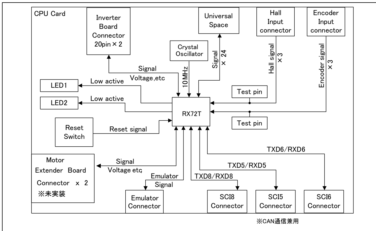
図 2.1 RX72T CPU カードブロック図
