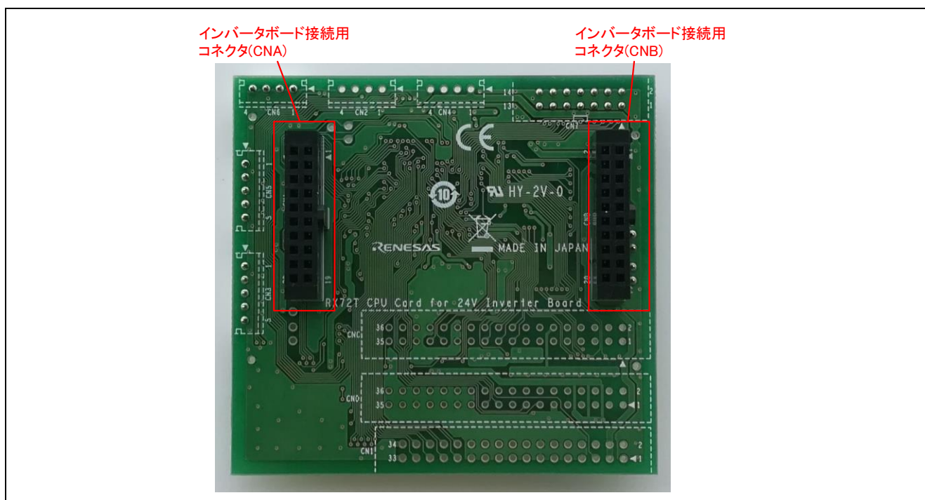
図 3.2 RX72T CPU カードレイアウト（裏面）
