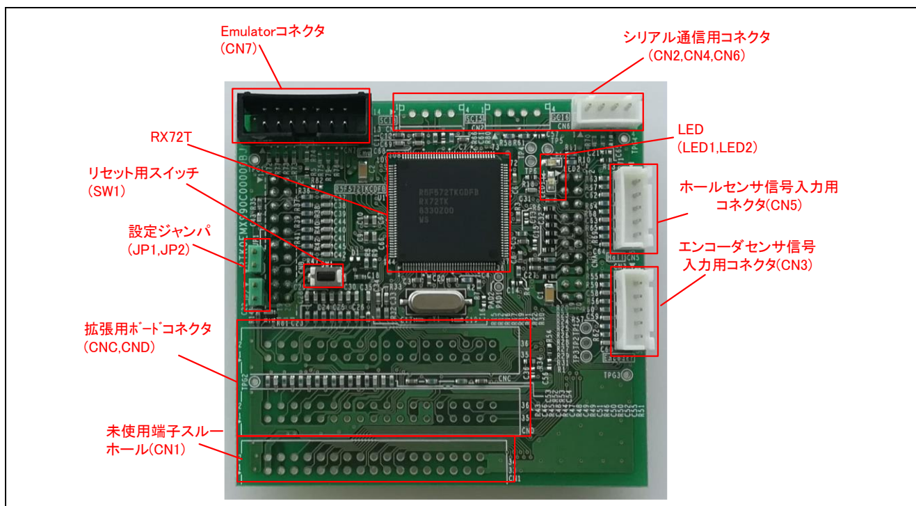
図 3.1 RX72T CPU カードレイアウト（表面）
