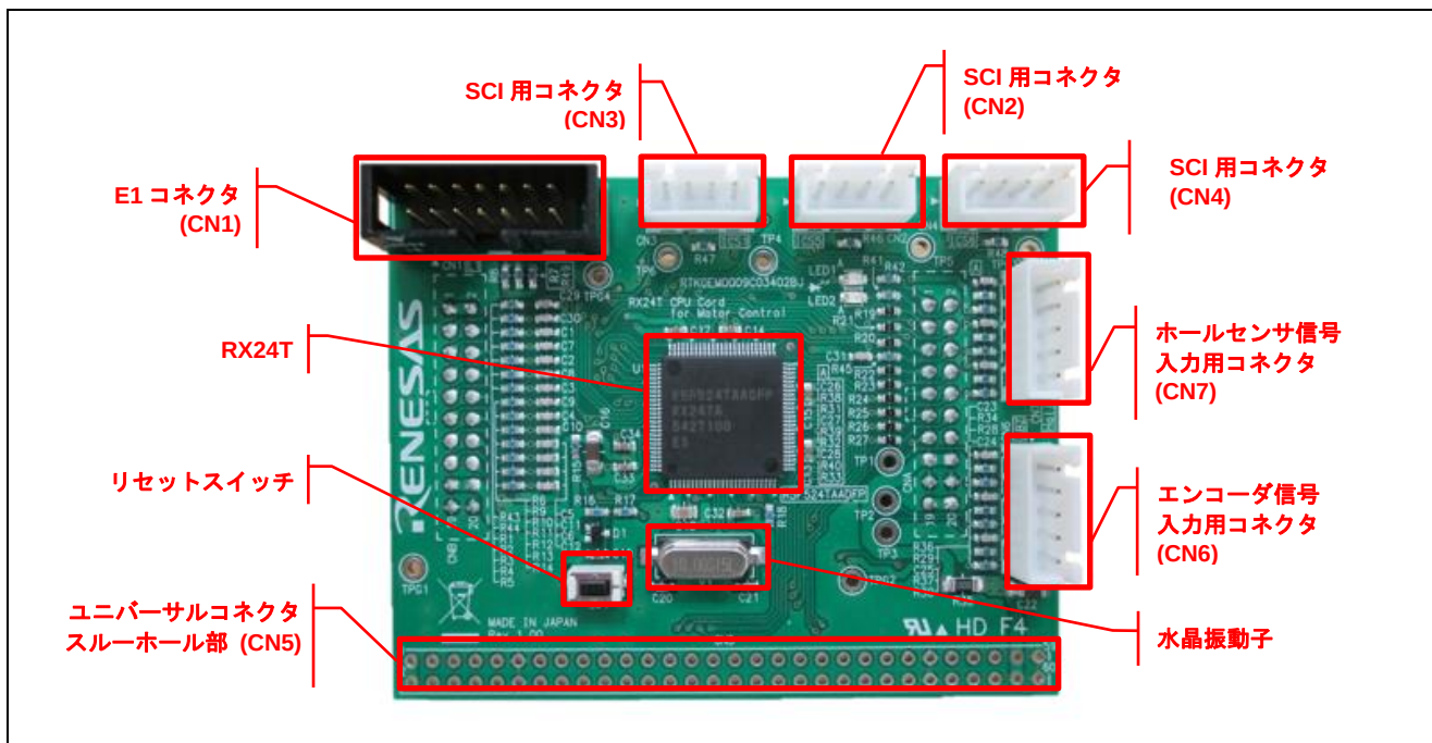
図 3.1 RX24T CPU カードレイアウト（表面）
