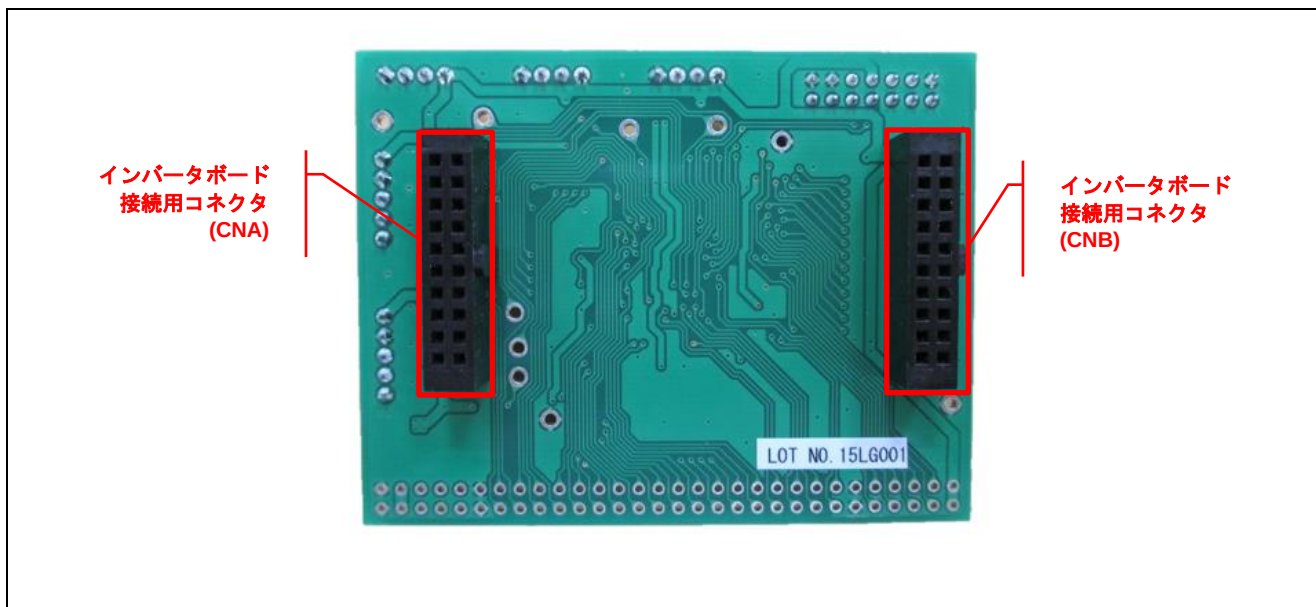
図 3.2 RX24T CPU カードレイアウト（裏面）
