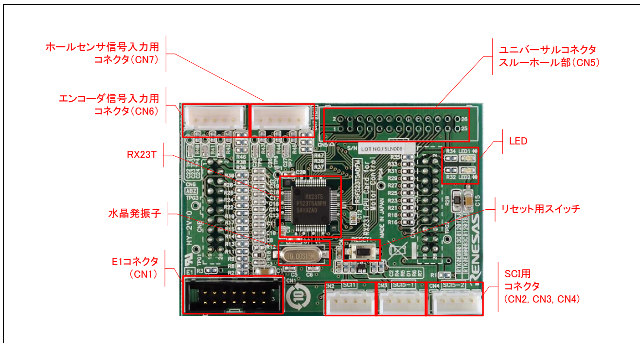
図 3.1 RX23T CPU カードレイアウト (表面)
