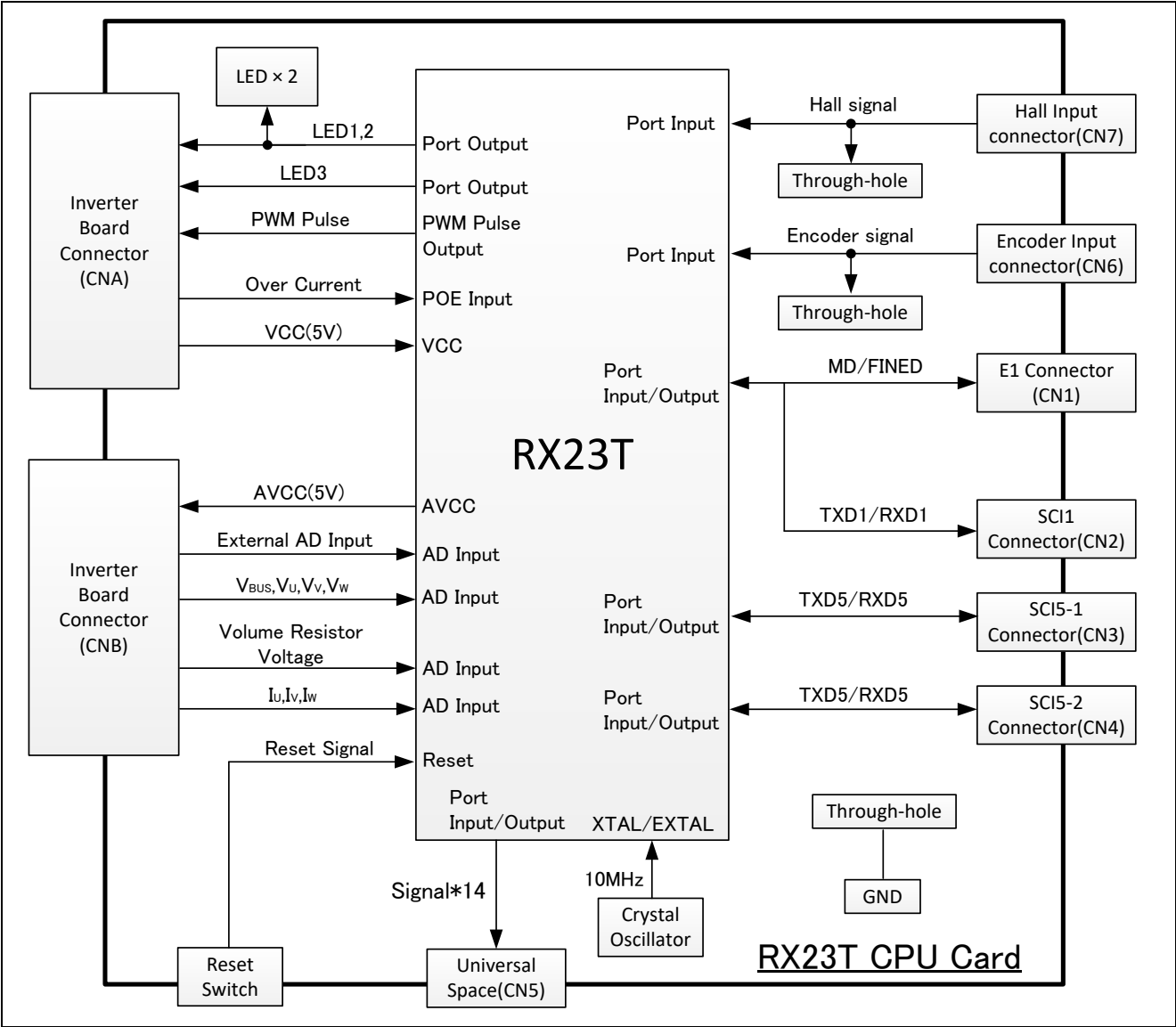
図 2.1 RX23T CPU カードブロック図
