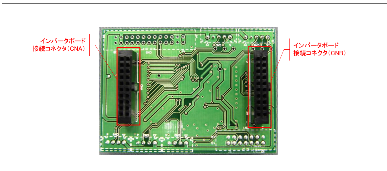
図 3.2 RX23T CPU カードレイアウト (裏面)
