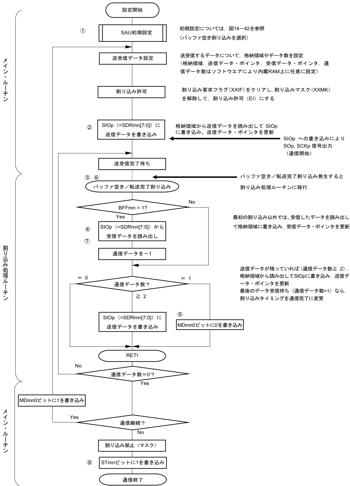
図14-48 マスタ送受信（連続送受信モード時）のフロー・チャート
