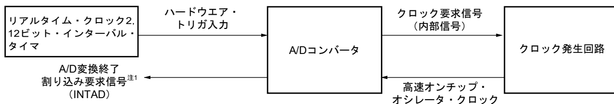
図12-28 SNOOZEモード機能時のブロック図
