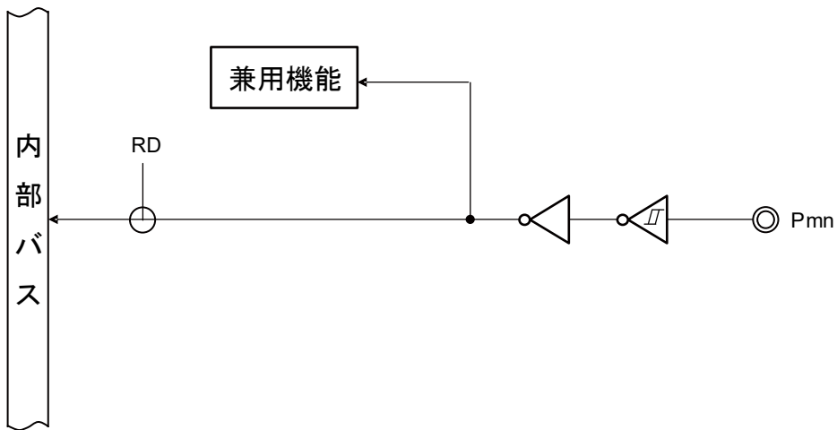
図2-2 端子タイプ 2-1-2 の端子ブロック図
