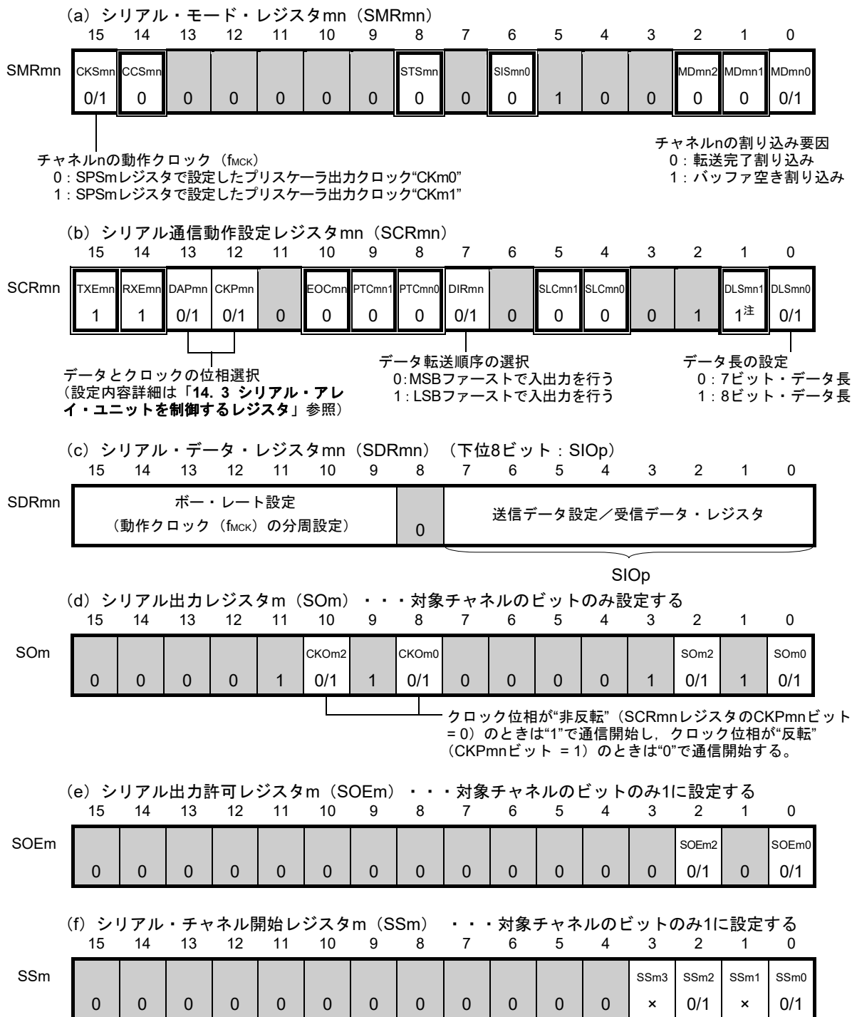
図14-41 簡易SPI (CSI00, CSI10) のマスタ送受信時のレジスタ設定内容例
