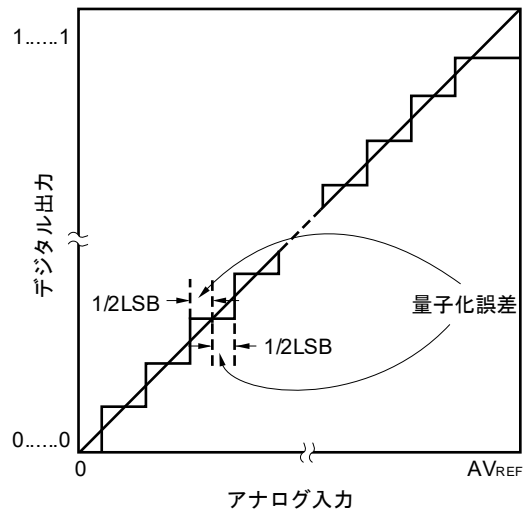
図12-33 量子化誤差
