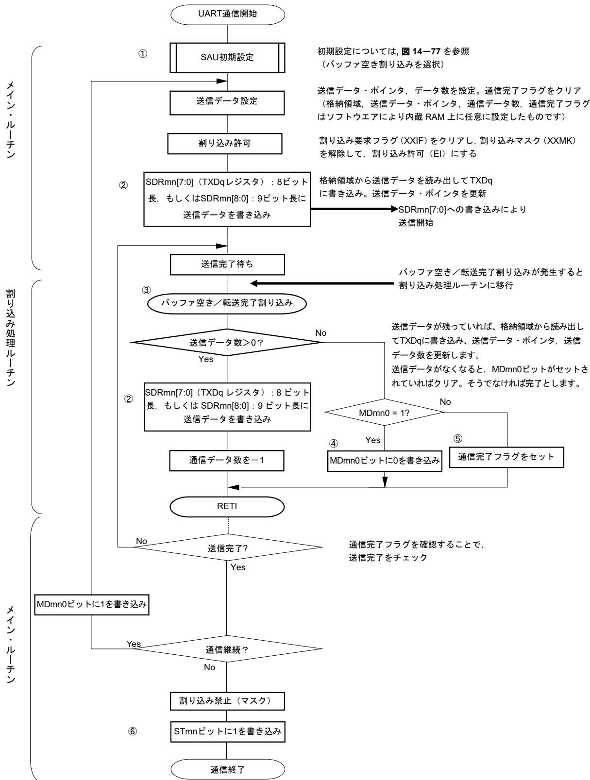
図14-83 UART送信（連続送信モード時）のフロー・チャート
