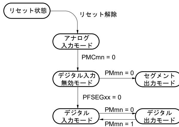
図4-13 ANIxx/SEGxx/ポート端子機能の状態遷移図
