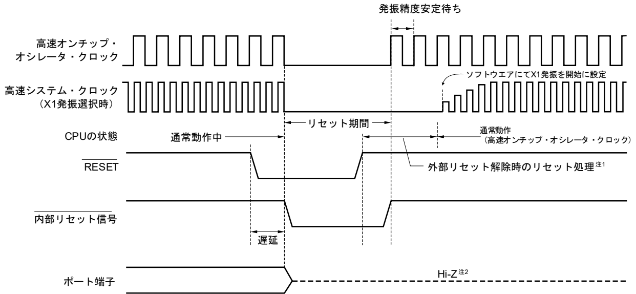
図22-2 \overline{\text{RESET}} 入力によるリセット・タイミング
