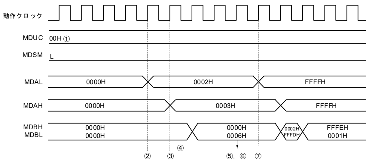
図17-6 乗算（符号なし）動作のタイミング図（ 2 \times 3 = 6 ）
