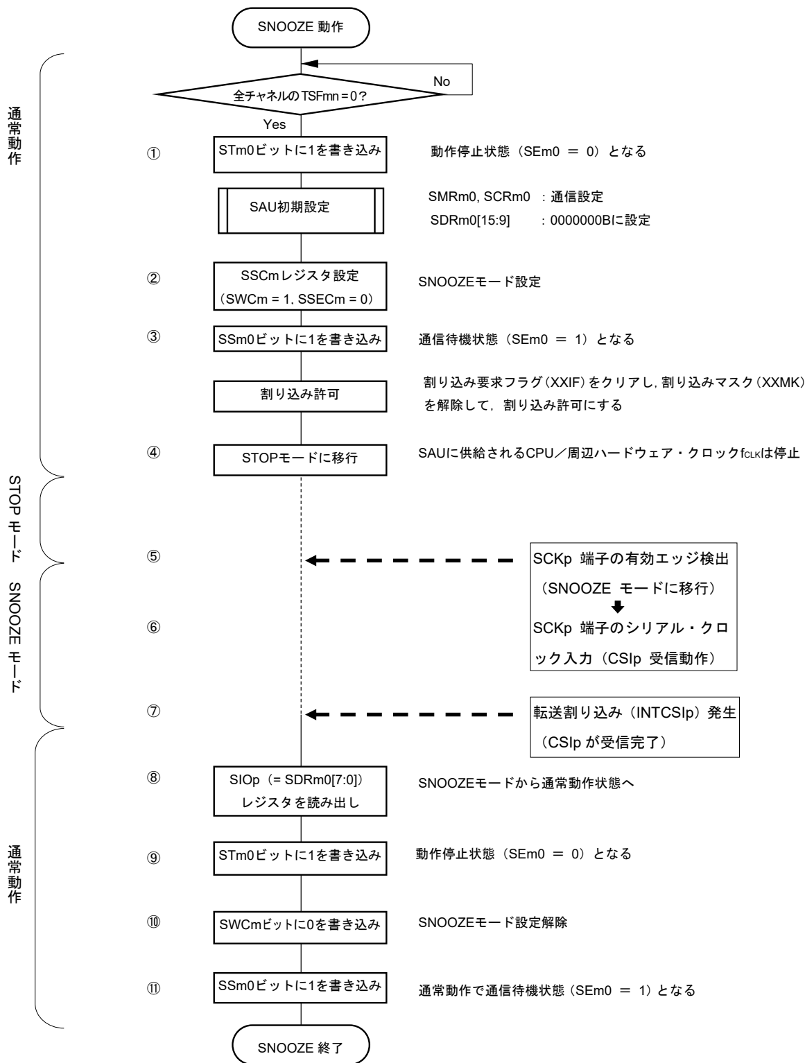
図14-72 SNOOZEモード動作（1回起動）時のフロー・チャート
