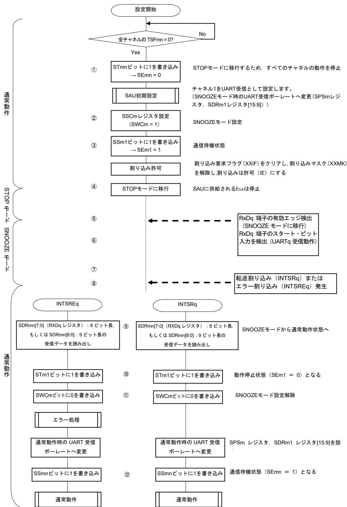
図14-92 SNOOZEモード動作 (EOCm1 = 0, SSECm = 0/1もしくはEOCm1 = 1, SSECm = 0) 時の フロー・チャート
