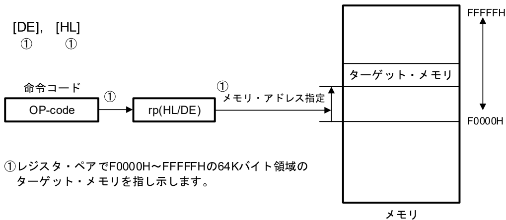
図3-26 [DE], [HL]の例
