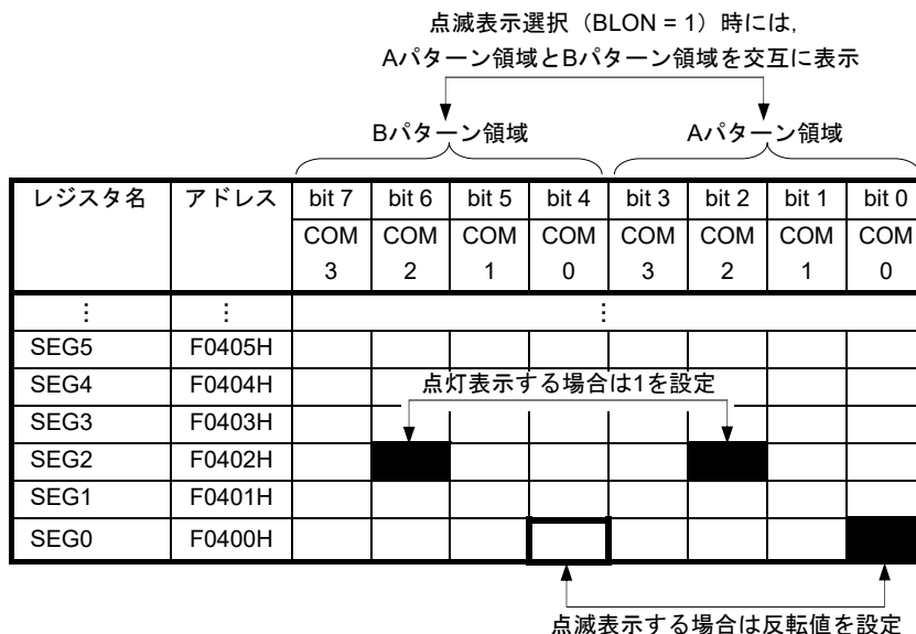
図16-14 パターン切り替え表示時のLCD表示レジスタの設定例
