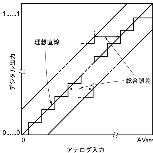
図12-32 総合誤差
