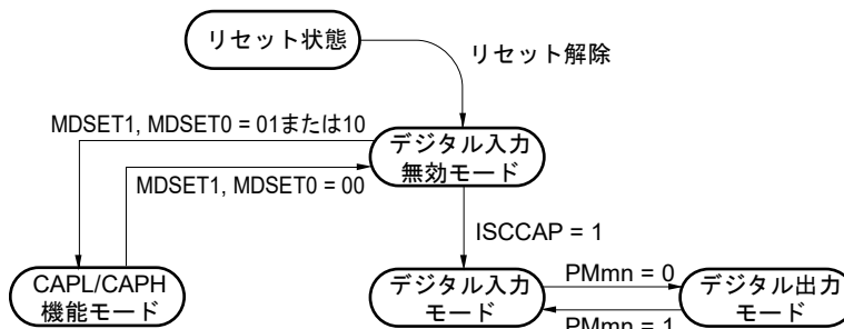
図16-9 CAPL/P126, CAPH/P127端子機能の状態遷移図
