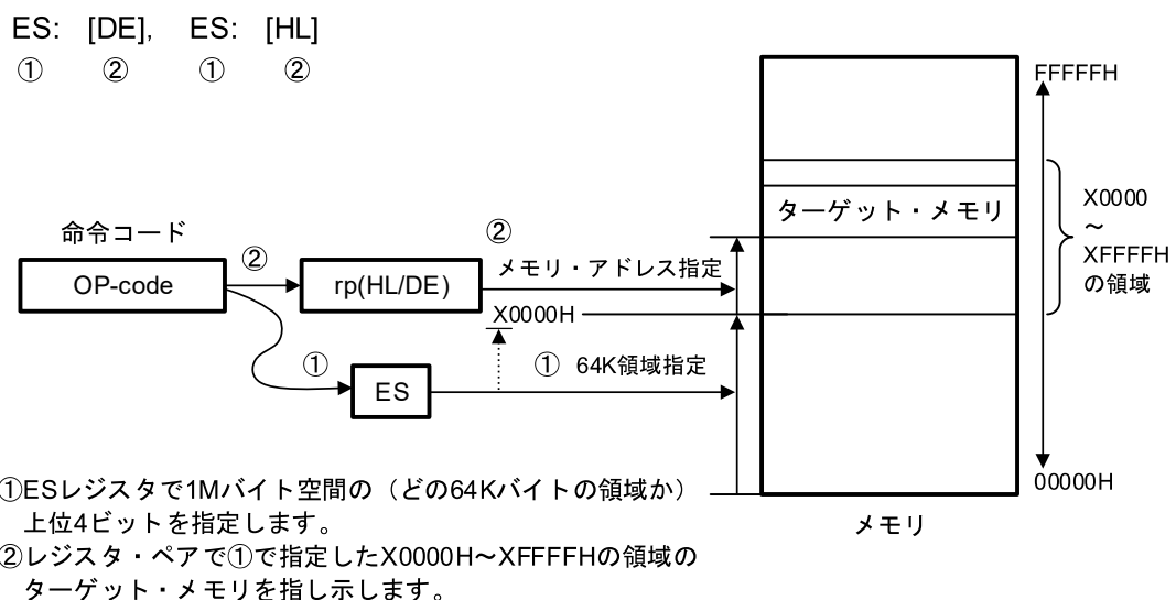
図3-27 ES:[DE], ES:[HL]の例
