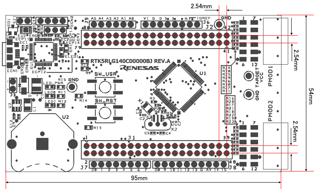
図 3-1: 部品配置図
