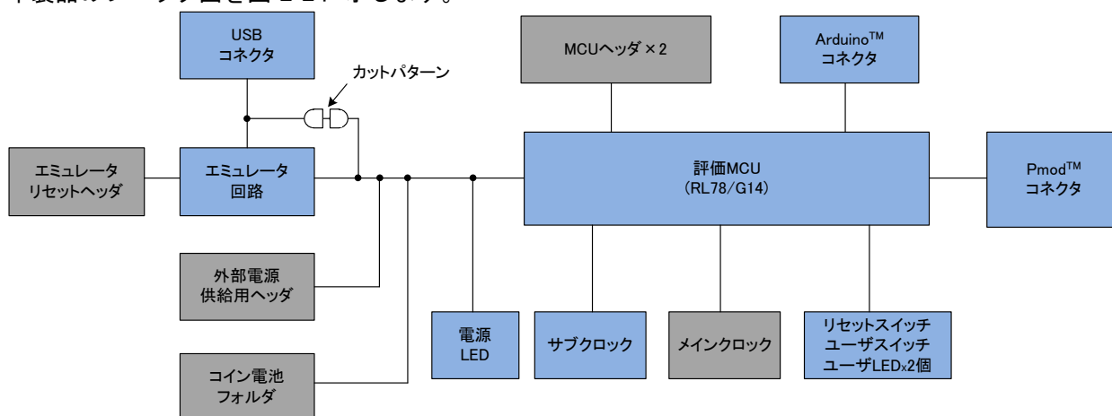
図 1-1: ブロック図
