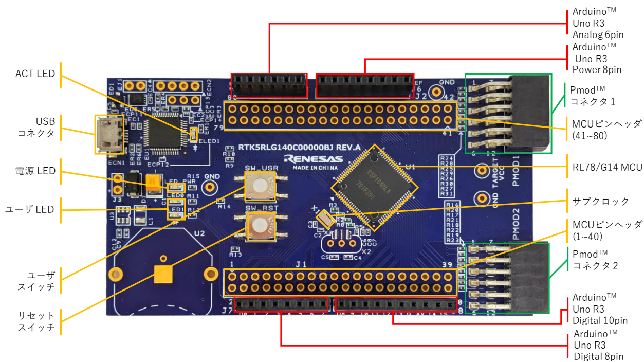
図 2-1: 部品面外観図
