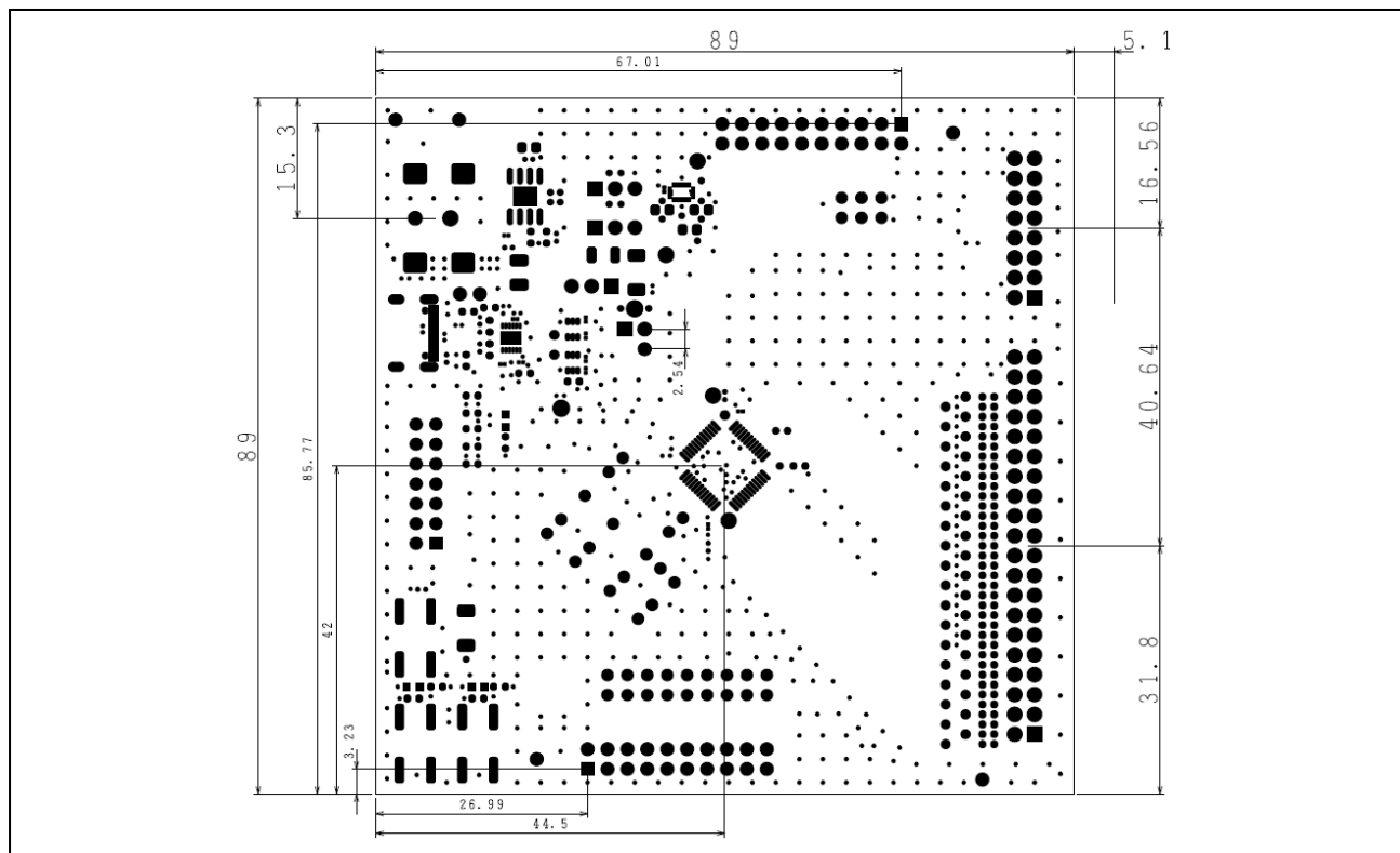
図 2-3 寸法図
