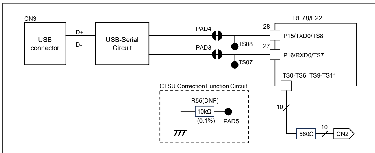
図 2-9 MCU と USB シリアル変換回路間のインタフェース・CTSUS 補正回路(オプション)
