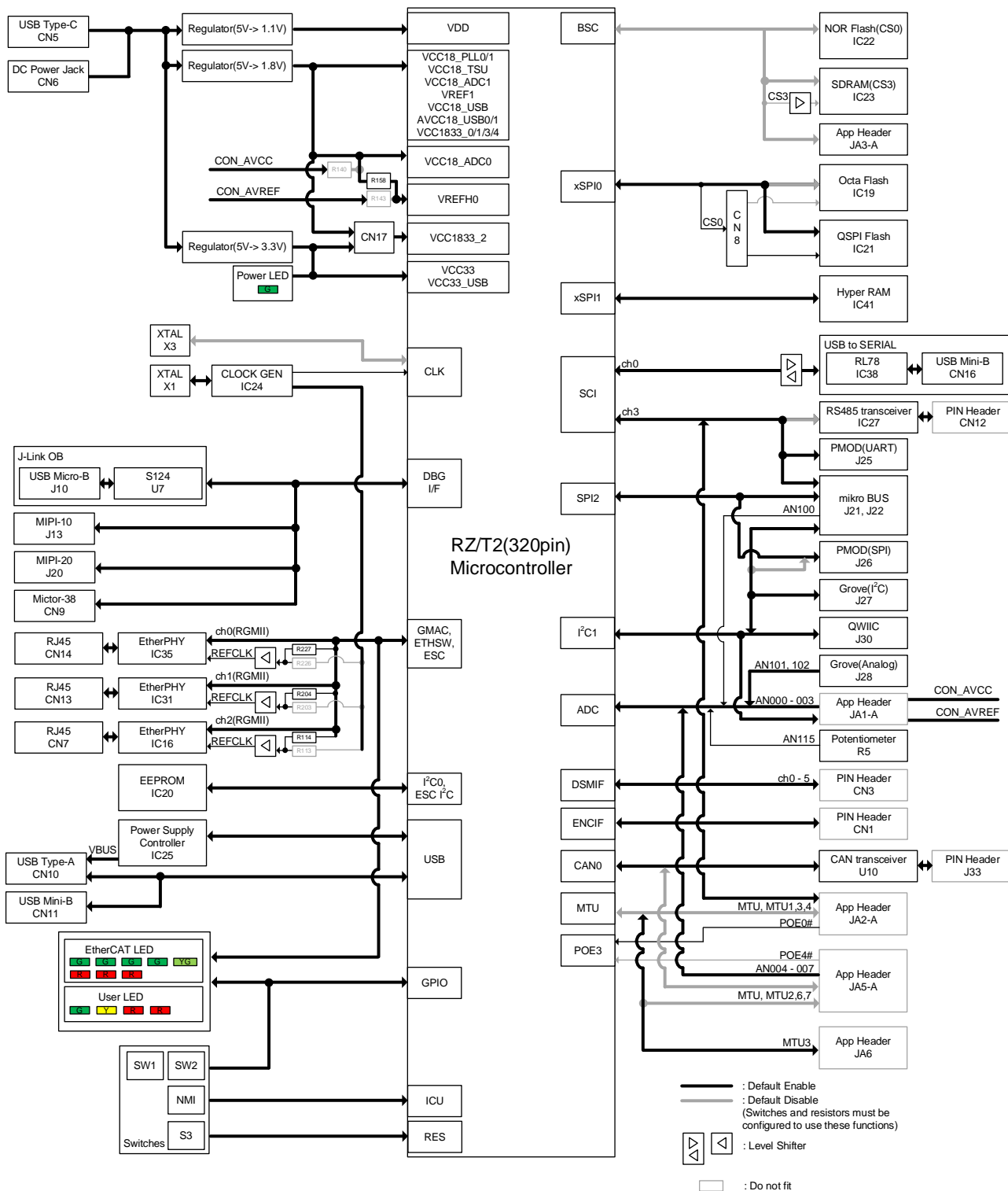
図 4-1: ボード内部の接続関係
