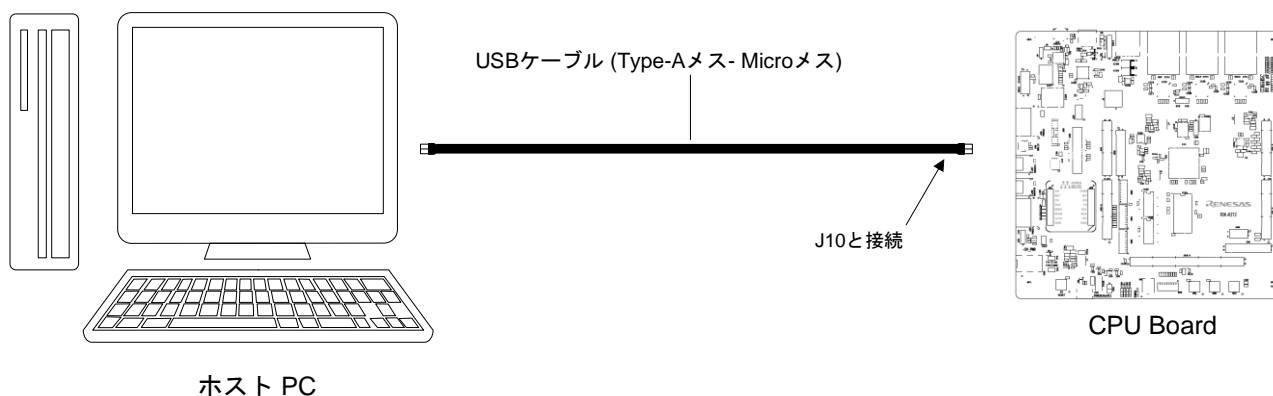
図 4-3: デバッグ環境の接続関係(J-Link® OB)
