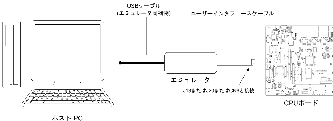
図 4-2: デバッグ環境の接続関係(エミュレータ)
