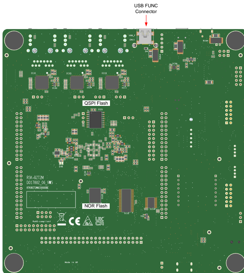
図 3-2: ボードレイアウト(ハンダ面)
