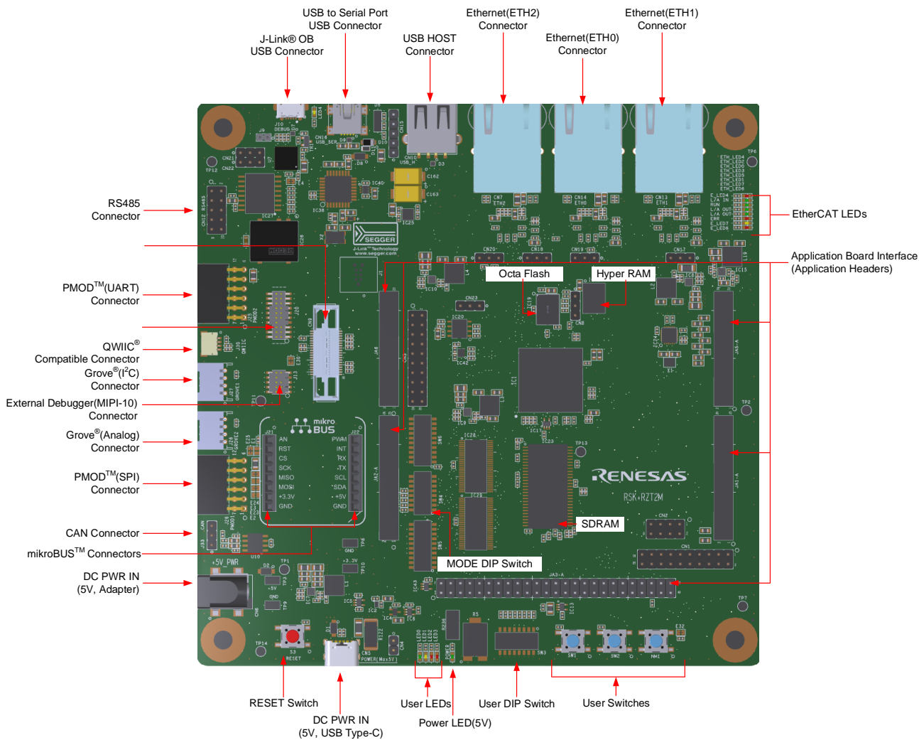
図 3-1: ボードレイアウト(部品面)
