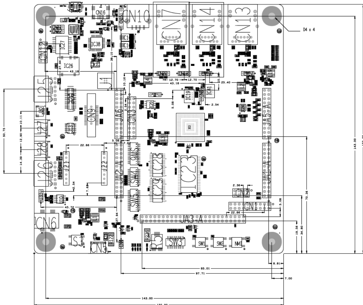
図 3-3: ボード寸法図 (単位: mm)
