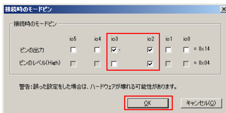
図1-5 [接続時のモードピン]ダイアログ
