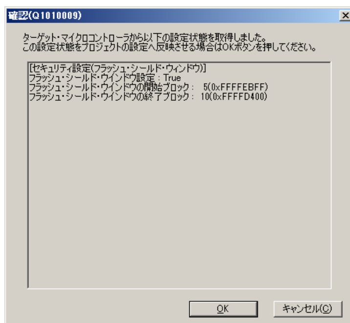
図2-34 [フラッシュオプションの取得(I)]コマンド
