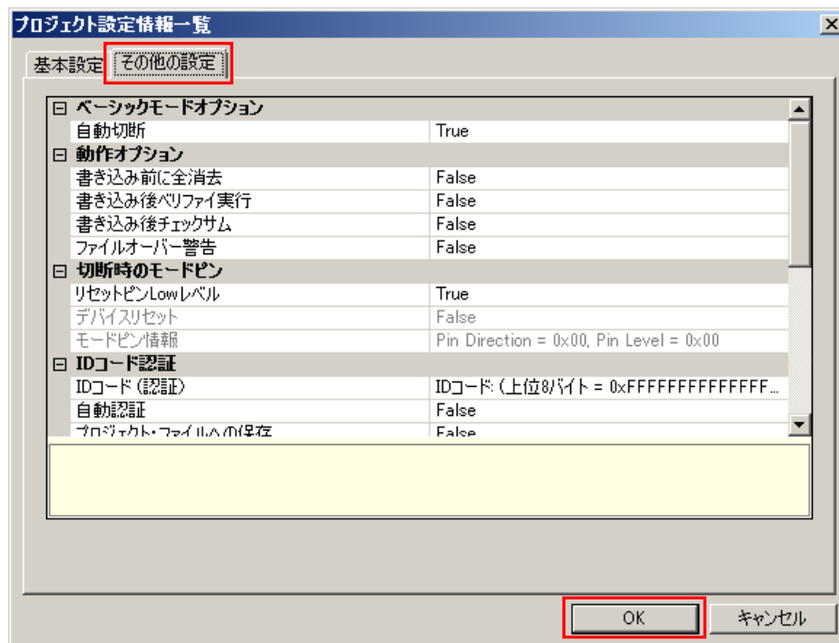
図1-12 [プロジェクト設定情報一覧]ダイアログ[その他の設定]タブ
