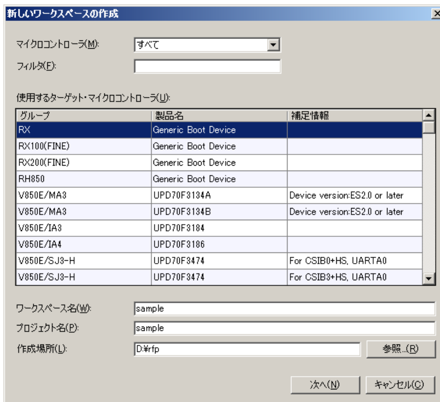
図2-23 [新しいワークスペースの作成]ダイアログ
