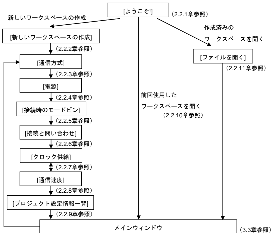
図3-1 起動までのダイアログの流れ
