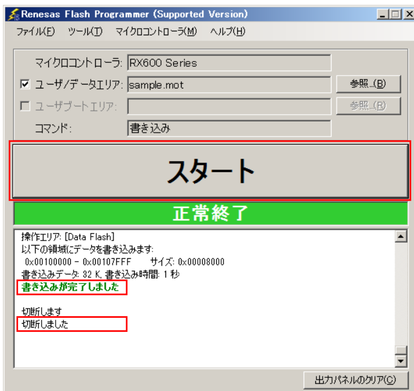
図1-16 [書き込み(P)]コマンド実行結果
