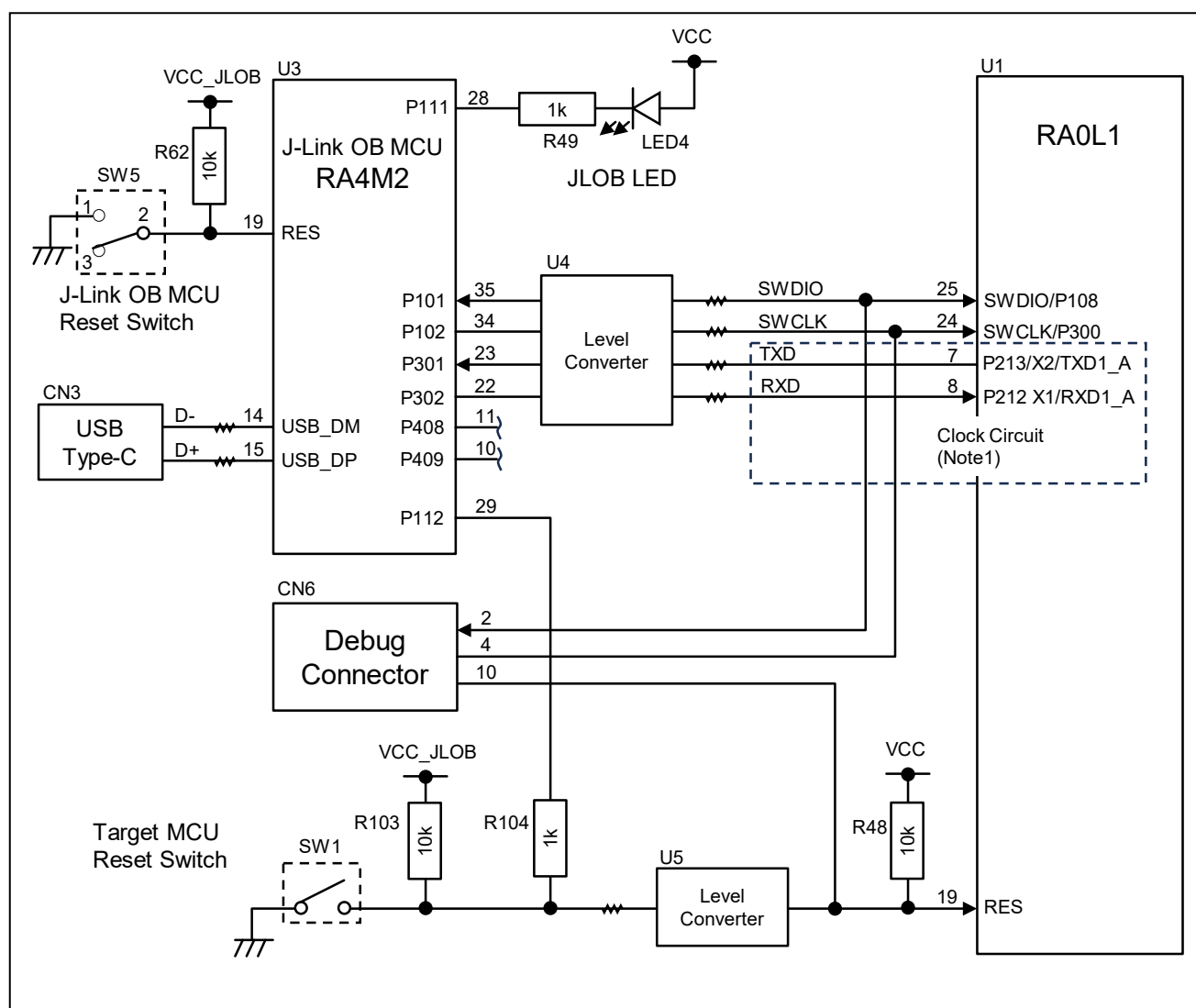
図 8 リセット回路・デバッグインタフェース
