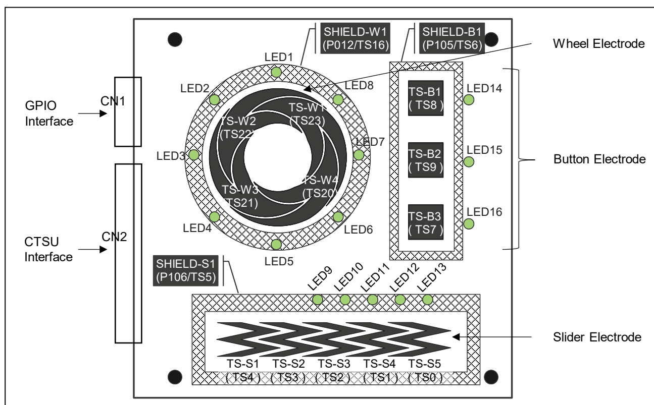
図 11 静電容量タッチアプリケーションボード (RA0L1 Cap Touch CPUボード接続時)
