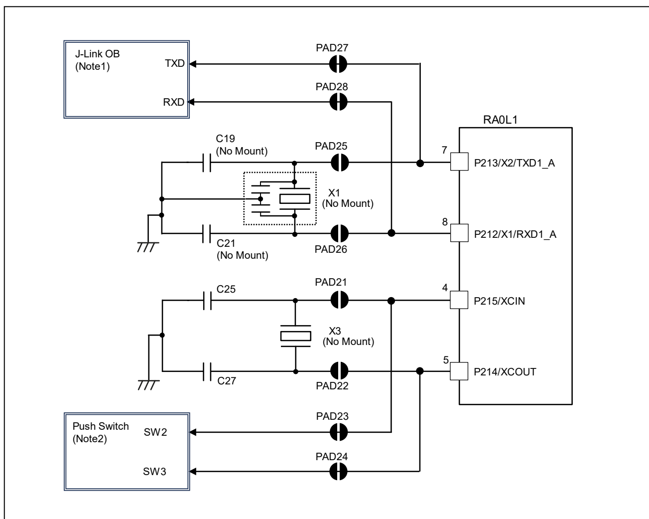
図 7 クロック回路
