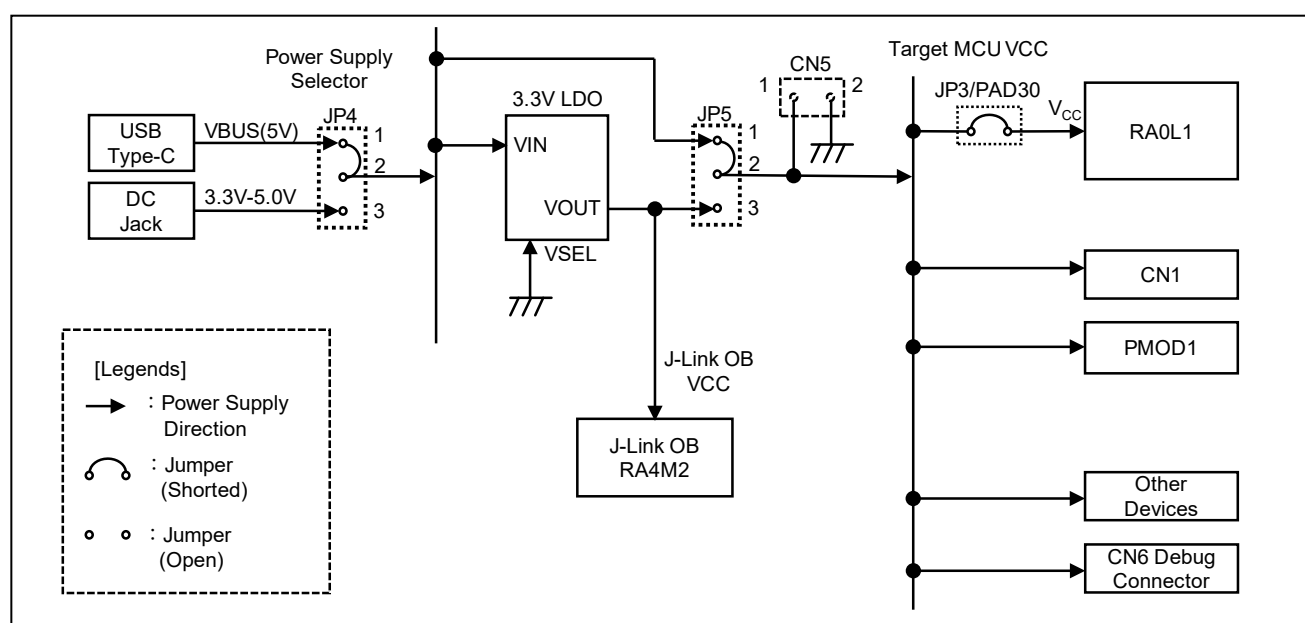
図 6 電源系統図
