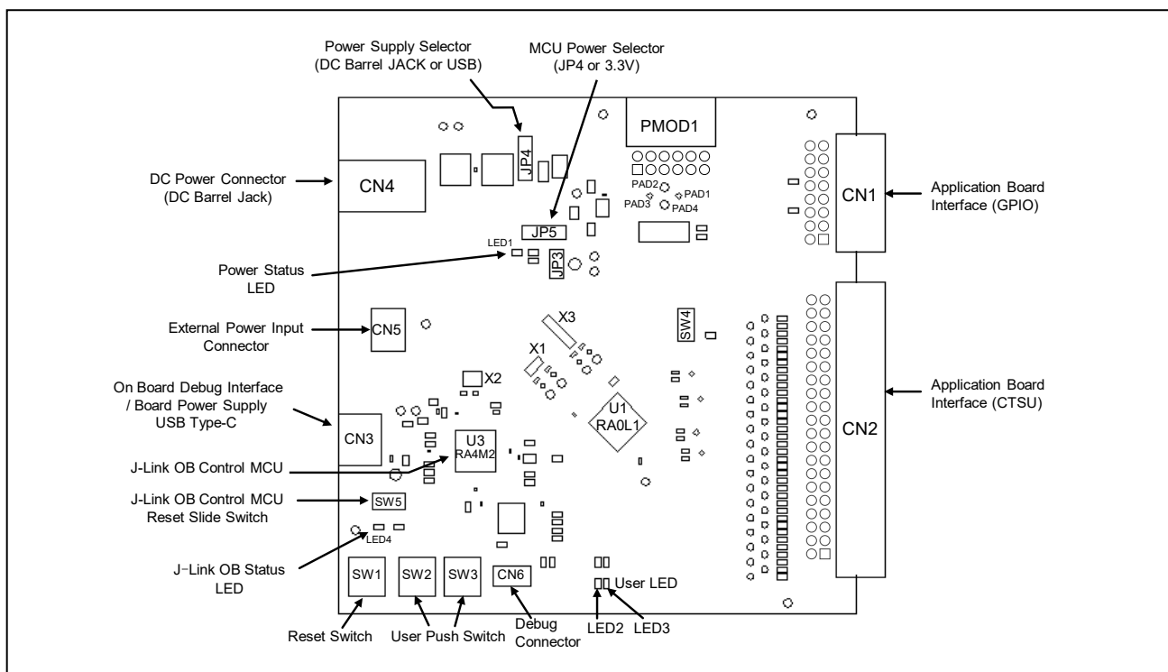
図 1 RA0L1 Cap Touch CPUボード
