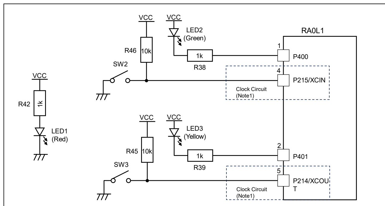
図 9 プッシュスイッチとLED回路
