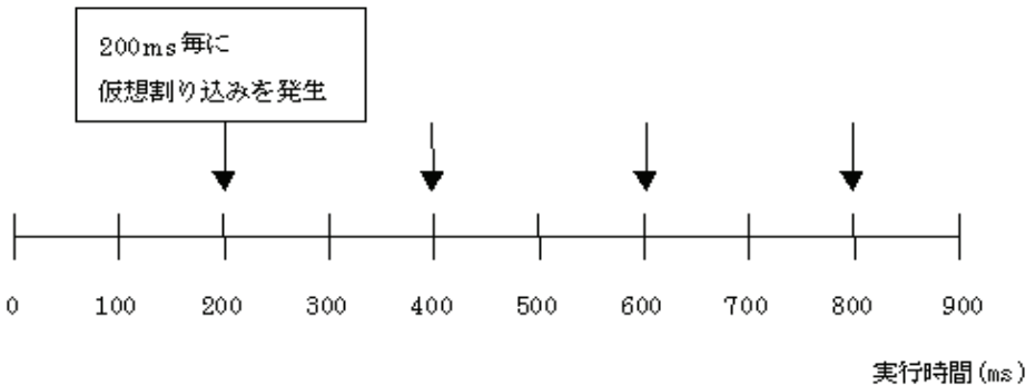
「ソフトウェア割り込み番号 21 番(タイマ A0)の仮想割り込みの定義例」
