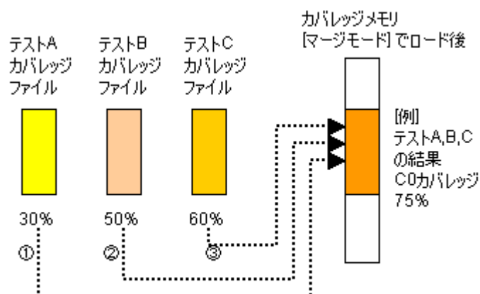
図5.101 [マージ] モードの応用例時の動作概略
