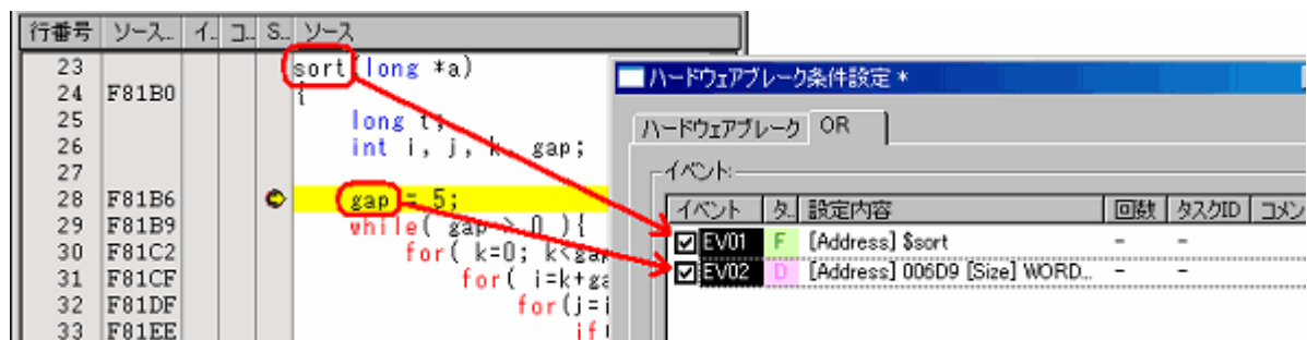
図5.32 【エディタ】ウィンドウと[ハードウェアブレイク条件設定]ダイアログボックス
