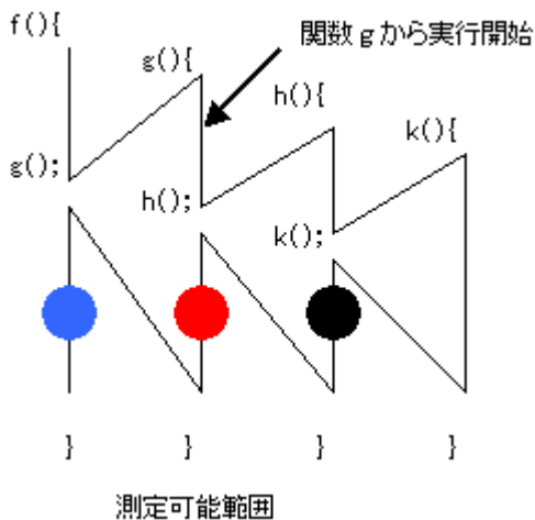
図5.129 測定可能な範囲について
