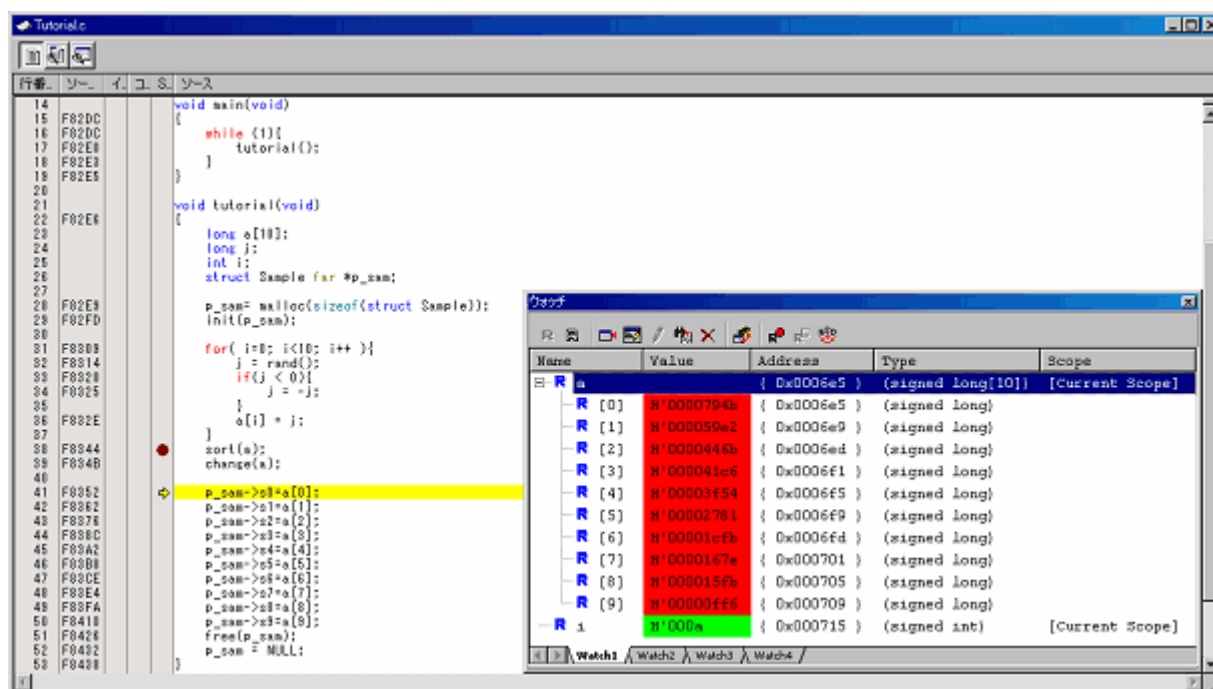
図3.24 [エディタ]ウィンドウ (ステップオーバ)
