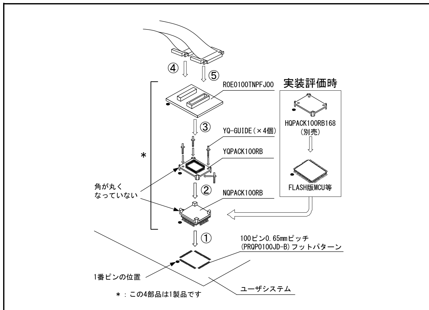
図2.11 100ピン0.65mmピッチフットパターンへの接続
