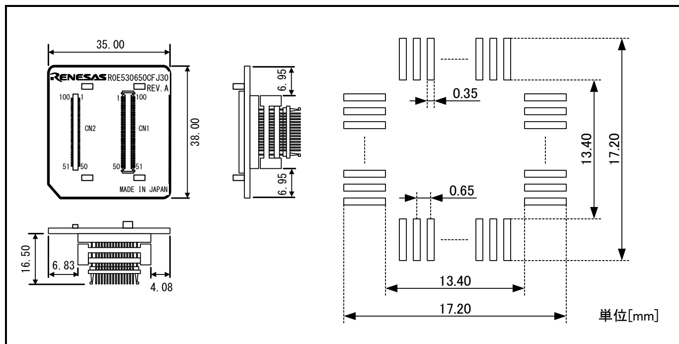
図7.5 R0E530650CFJ30ユーザシステム接続部の寸法図および参考フットパターン
