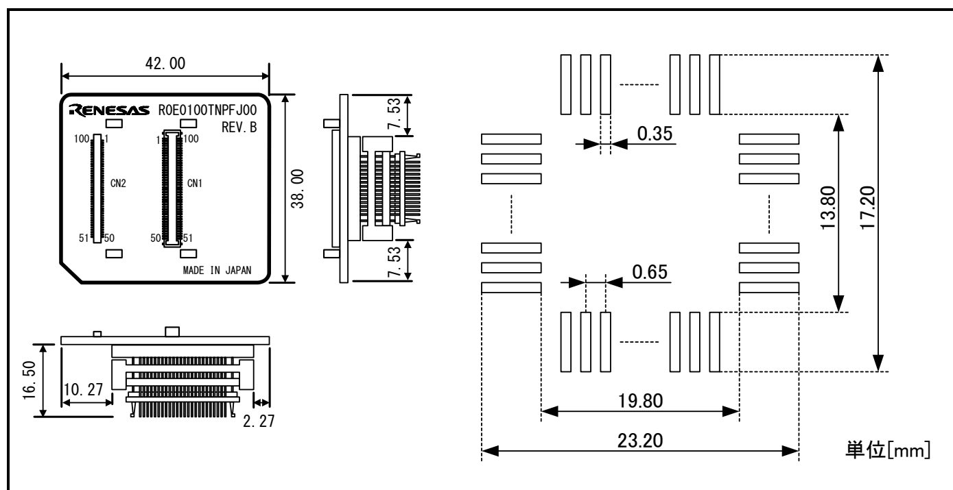
図7.3 R0E0100TNPFJ00ユーザシステム接続部の寸法図および参考フットパターン
