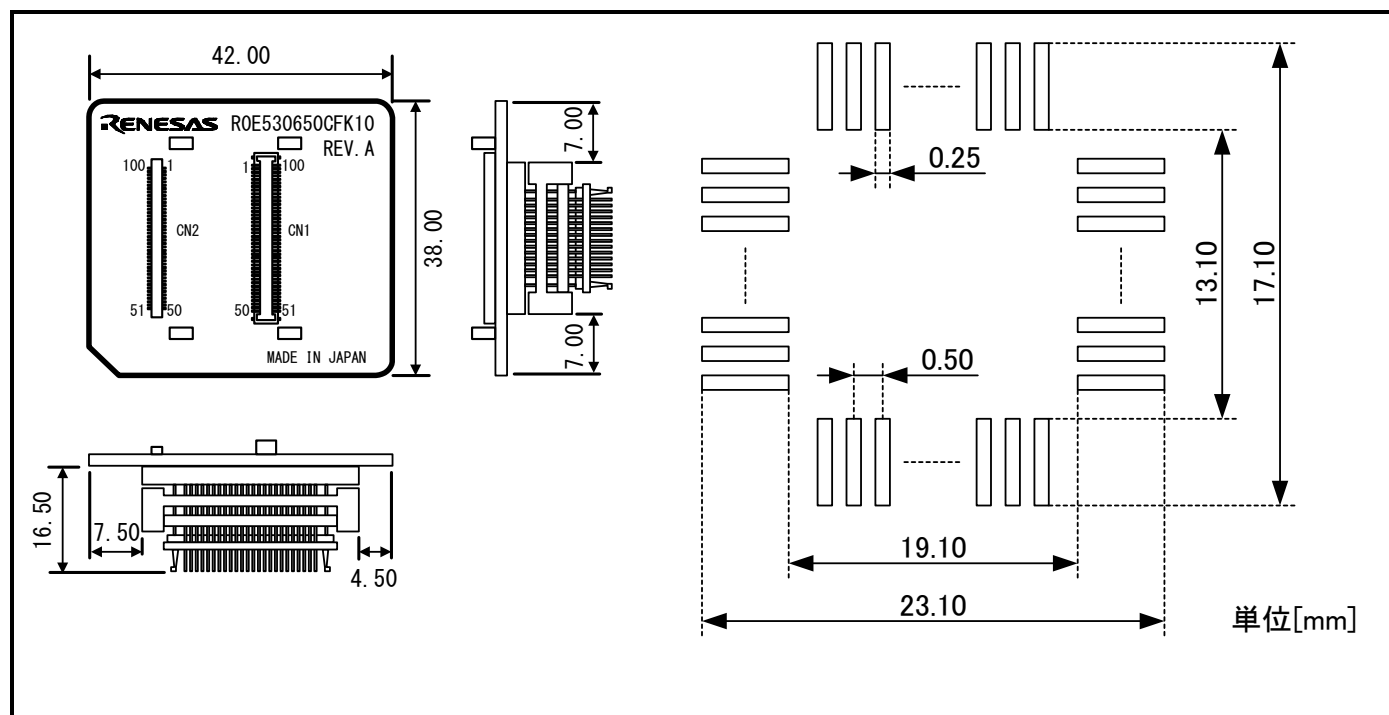
図7.6 R0E530650CFK10ユーザシステム接続部の寸法図および参考フットパターン
