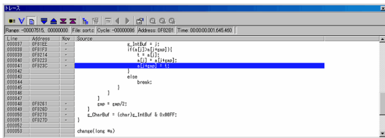
図5.59 ソース表示画面
