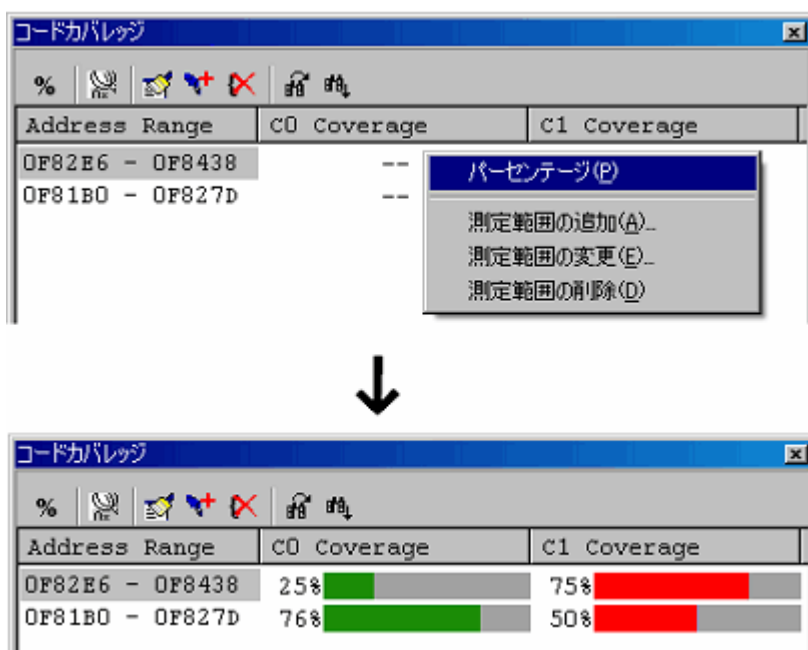
図5.93 [コードカバレッジ] ウィンドウ
