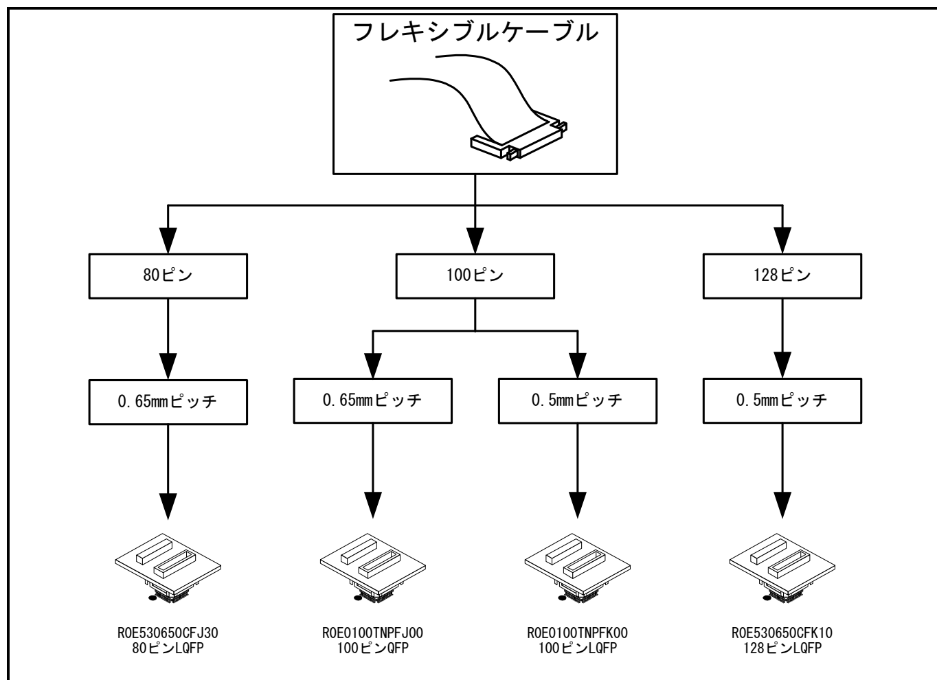
図2.10 本製品とユーザシステムとの接続
