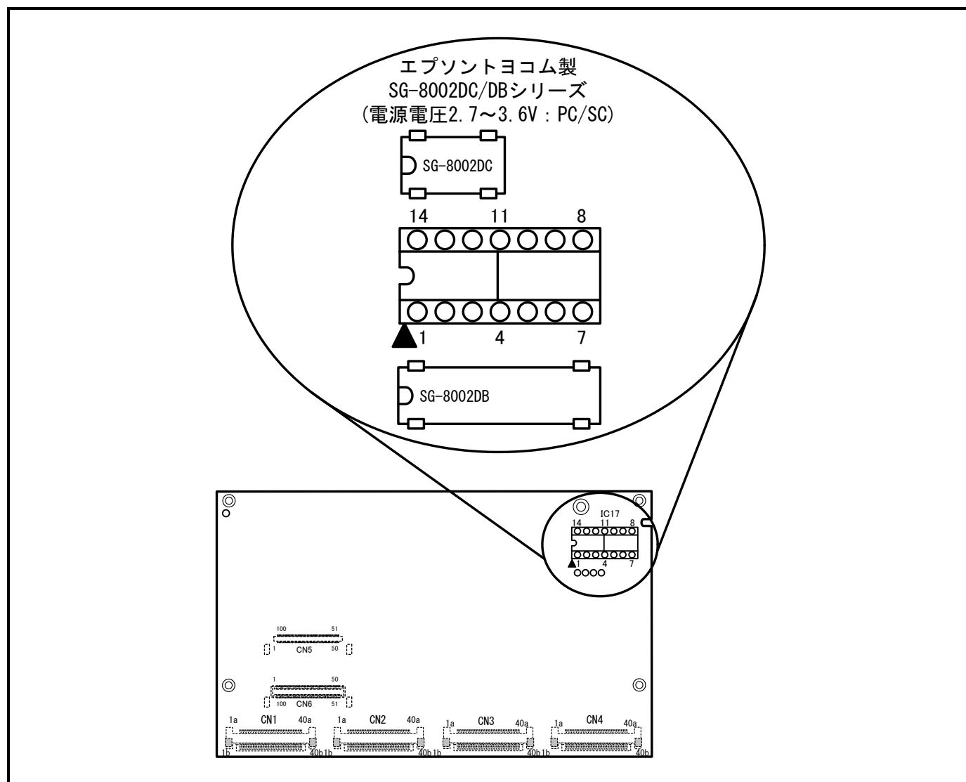
図2.7 発振モジュール交換
