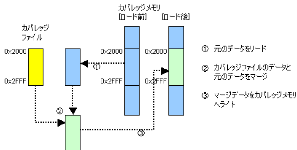
図5.100 [マージ] 選択時のロードモード動作概略
