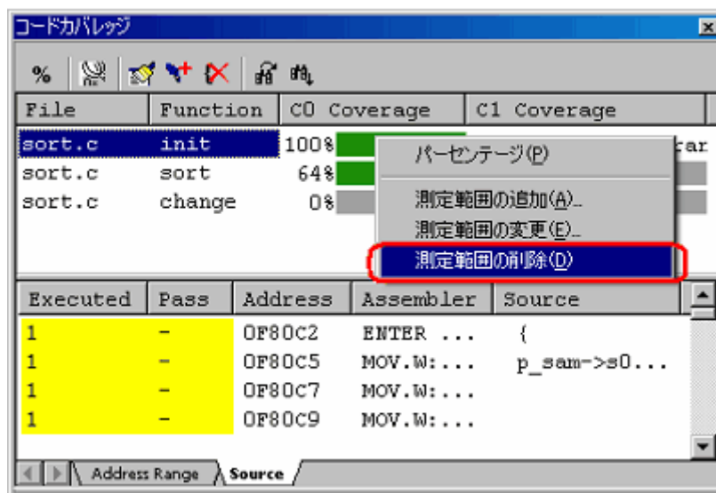
図5.90 [コードカバレッジ] ウィンドウ
