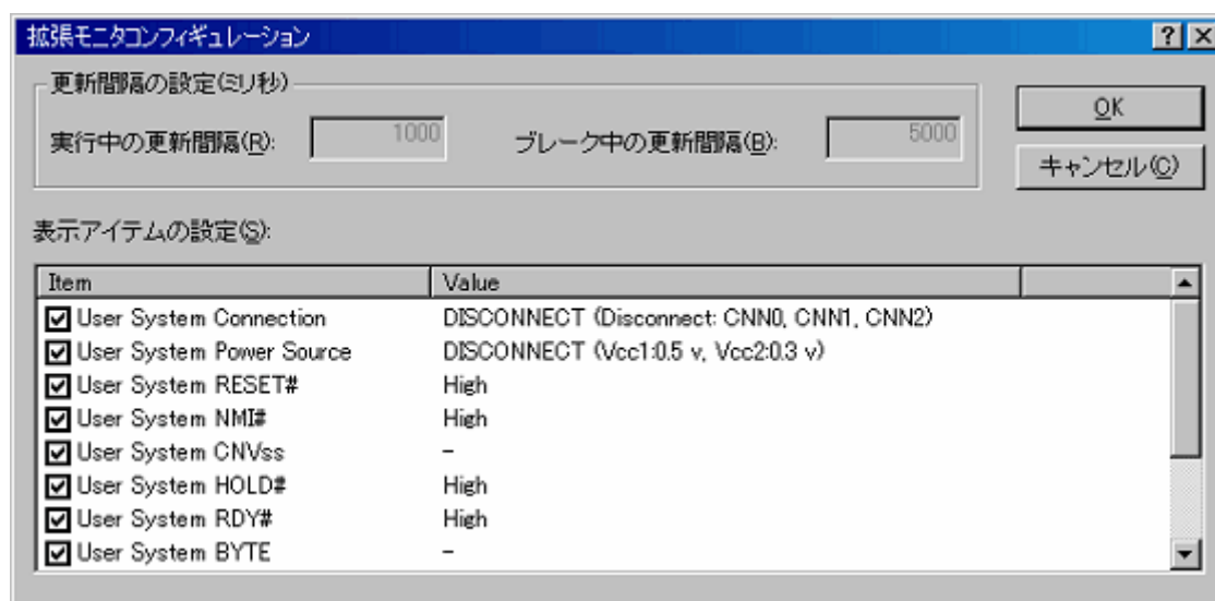
図5.18 [拡張モニタコンフィギュレーション] ダイアログボックス
