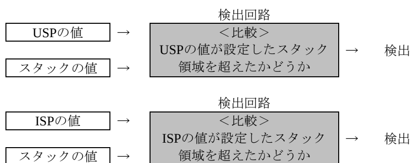
図5.146 スタックアクセス違反検出方法の概要
