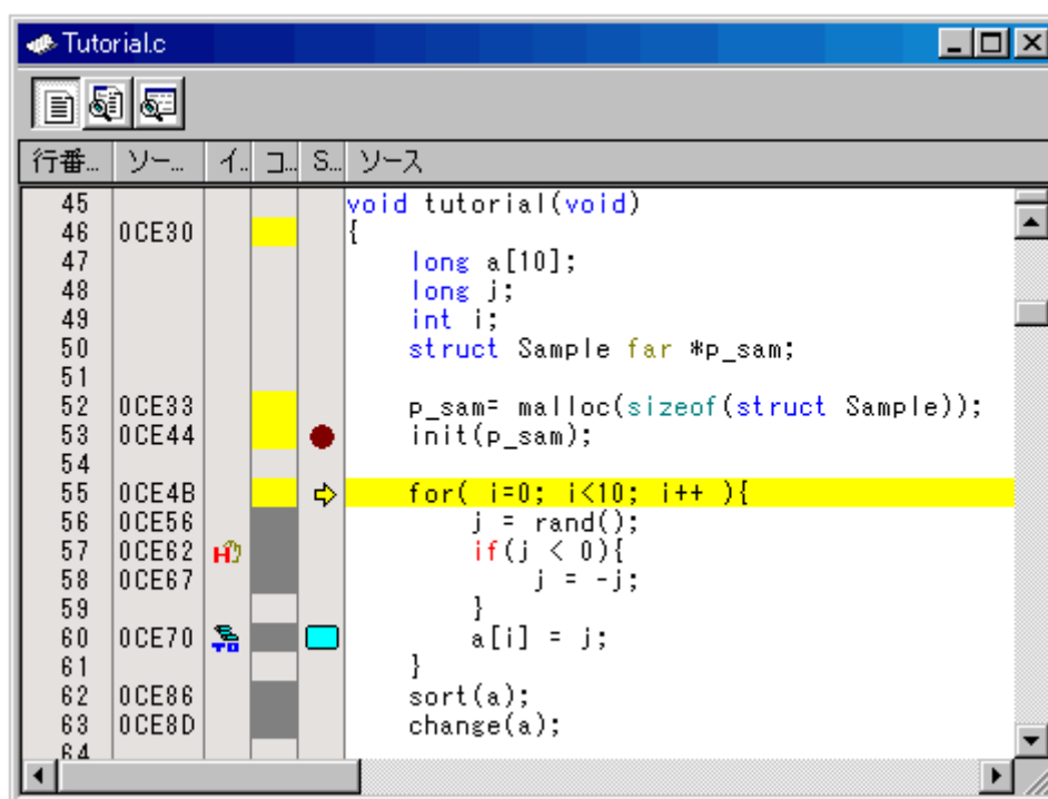
図5.7 [エディタ] ウィンドウ
