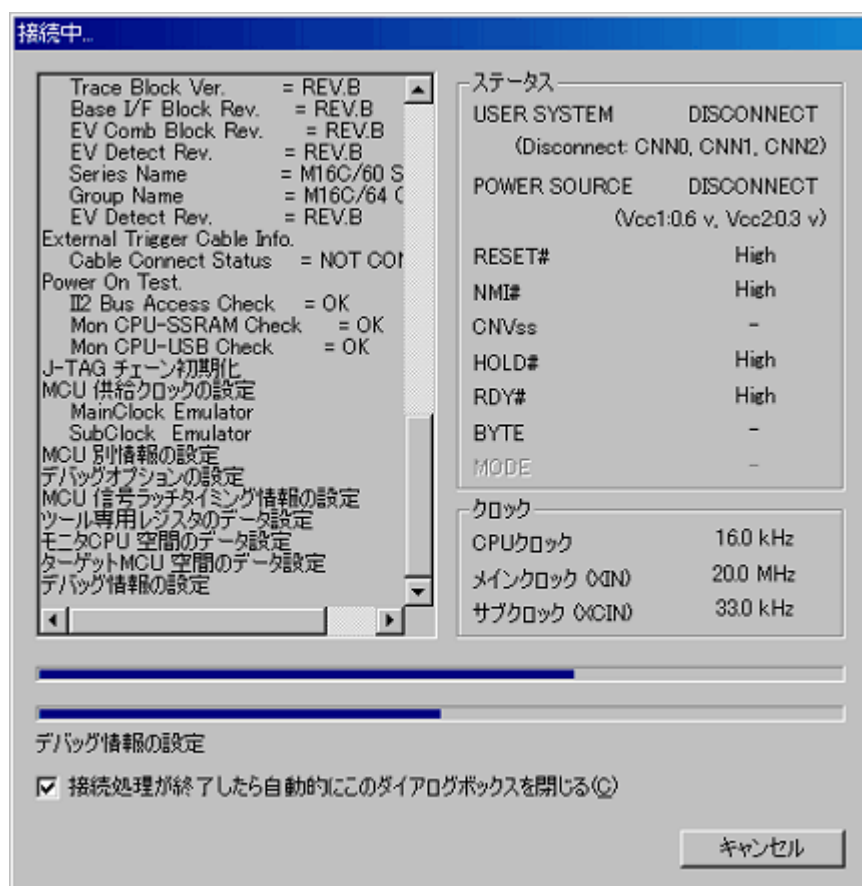
図5.6 [接続] ダイアログボックス
