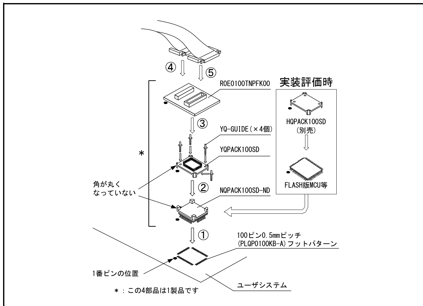
図2.12 100ピン0.5mmピッチフットパターンへの接続
