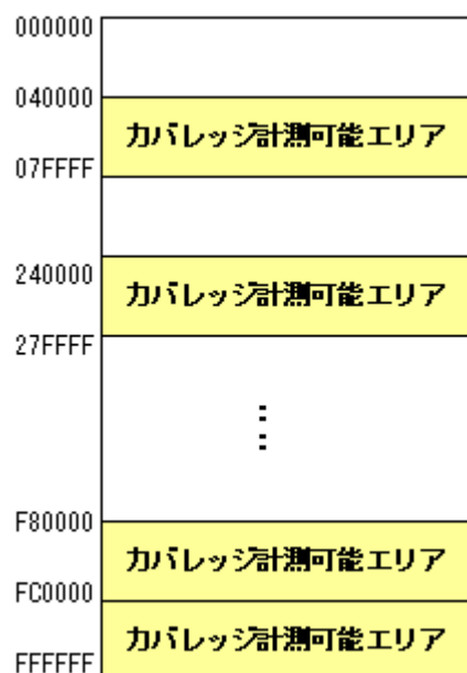
図5.74 [コードカバレレッジメモリ] の割り当て概略図
