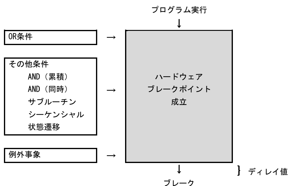
図5.42 ハードウェアブレイク概要
