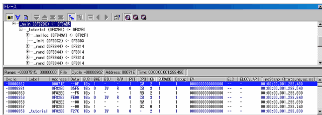
図5.64 [トレース] ウィンドウ
