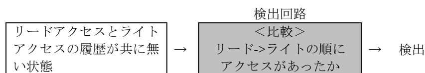
図 5.145 初期化抜け検出方法の概要
