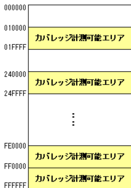
図5.105 [データカバレッジメモリ] の割り当て概略図
