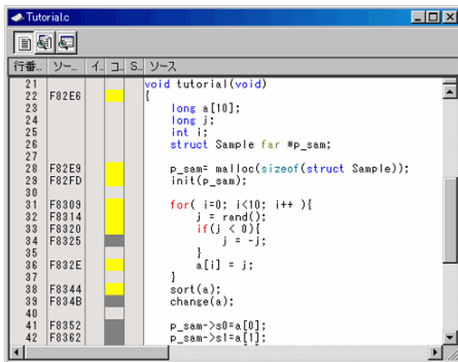
図5.102 コードカバレッジ結果の表示例
