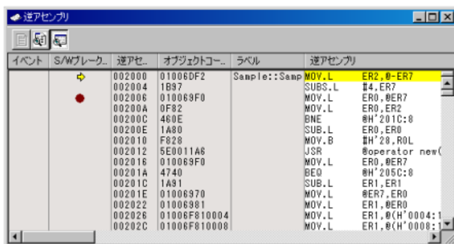
図5.10 [逆アセンブリ] ウィンドウ
