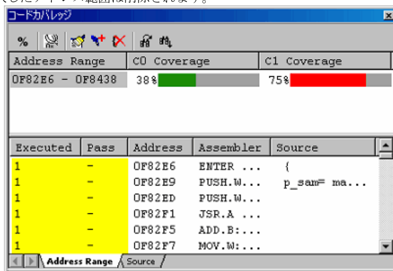
図5.85 「コードカバレッジ」ウィンドウ
