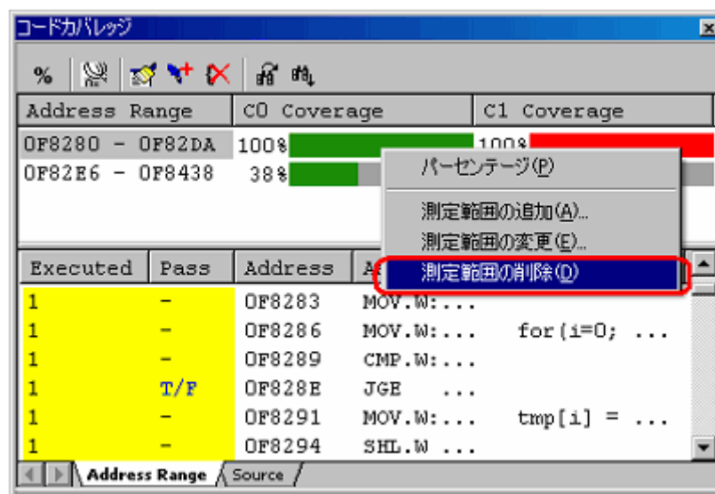
図5.83 [コードカバレッジ] ウィンドウ
