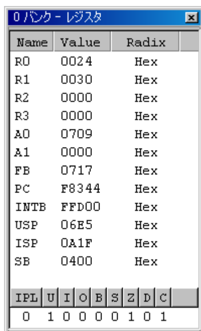
図3.8 [レジスタ]ウィンドウ
