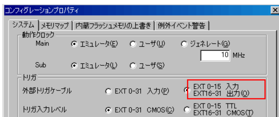
図5.154 [コンフィグレーションプロパティ]ダイアログボックス—システムページ
