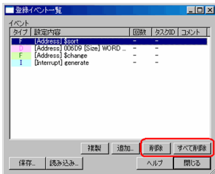
図5. 35 [登録イベント一覧] ダイアログボックス
