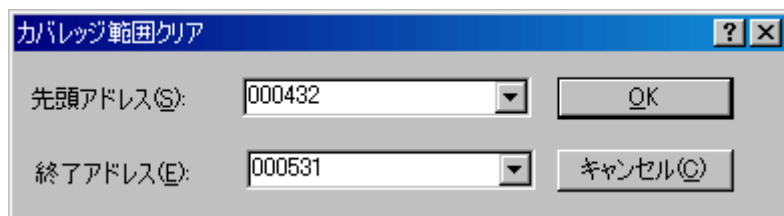
図5.125 [カバレッジ範囲クリア] ダイアログボックス
