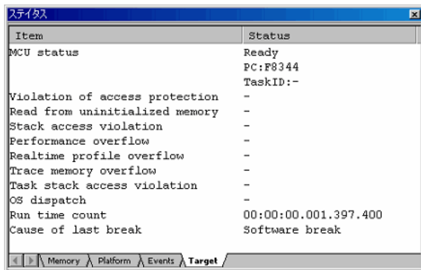
図3.6 [ステイタス]ウィンドウ
