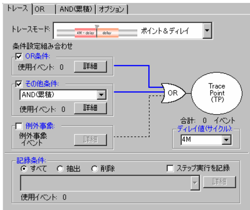
図5.52 [トレース条件設定] ダイアログボックス
