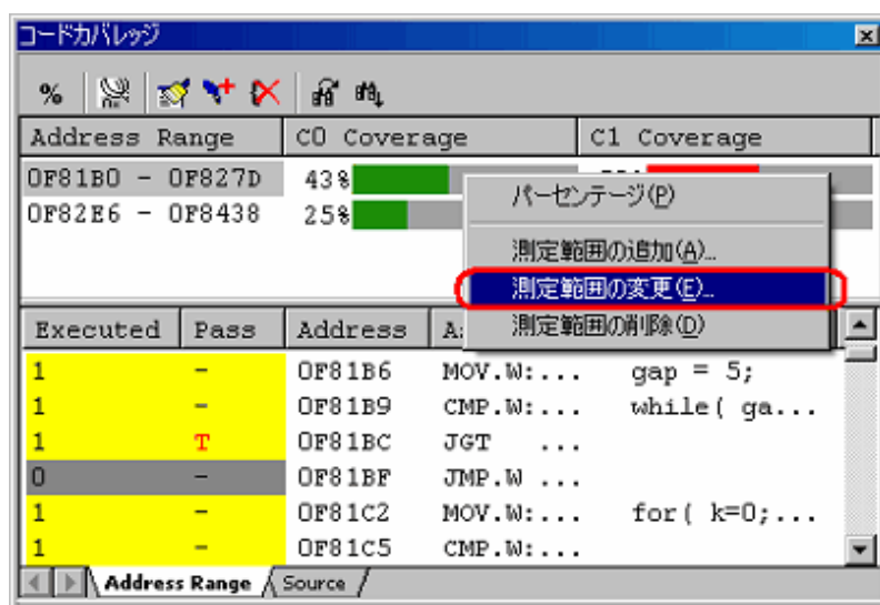
図5.80 [コードカバレッジ] ウィンドウ
