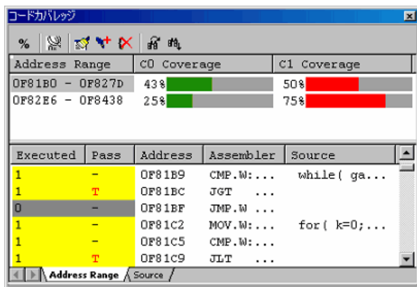
図5.76 [コードカバレッジ] ウィンドウ（アドレス指定）
