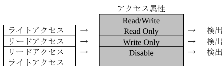
図5.137 検出方法のNGパターン
