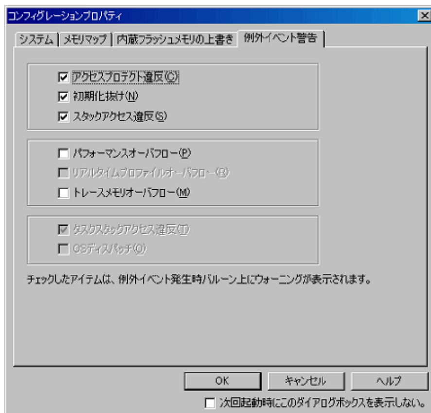
図5.5 ［コンフィグレーションプロパティ］ダイアログボックス－例外イベント警告ページ
