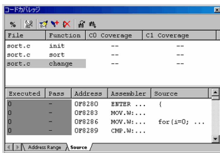
図5.89 [コードカバレッジ] ウィンドウ
