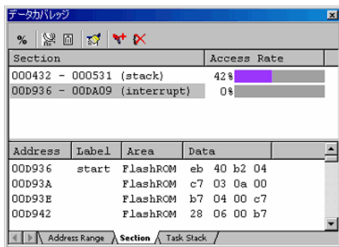
図5.123 [データカバレッジ] ウィンドウ
