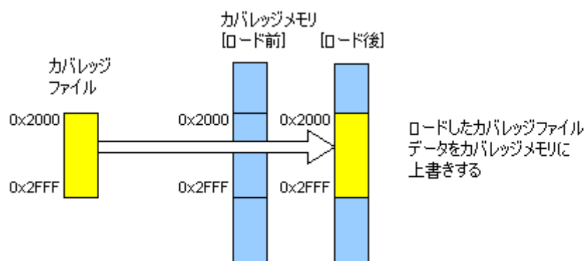
図5.99 [上書き] 選択時のロードモード動作概略
