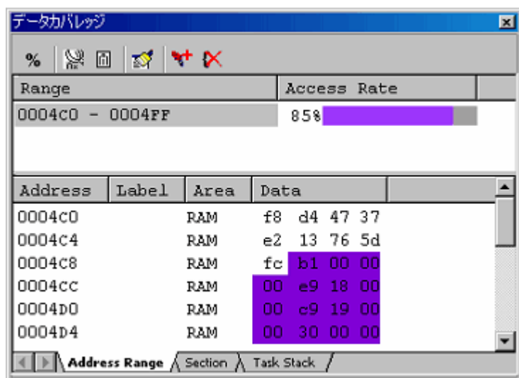
図5.107 [データカバレッジ] ウィンドウ (アドレス指定)
