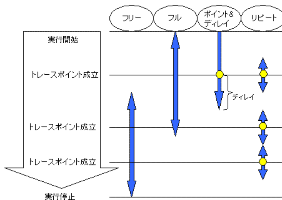
図5.49 トレースモードによる違い
