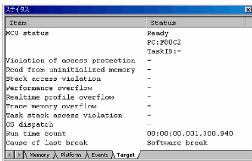
図5.13 [ステイタス] ウィンドウ
