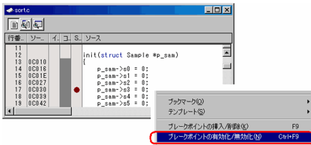
図5.21 [エディタ] ウィンドウとポップアップメニュー
