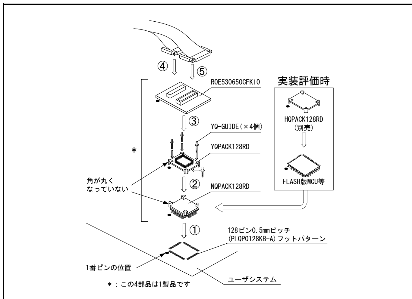
図2.14 128ピン0.5mmピッチフットパターンへの接続
