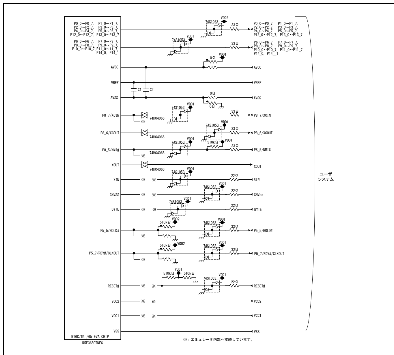
図7.1 R0E530650MCU00の接続図(一部)
