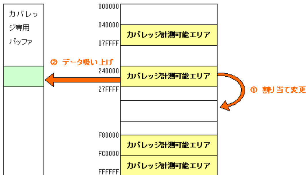
図5.75 [コードカバレレッジメモリ] の割り当て変更概略図
