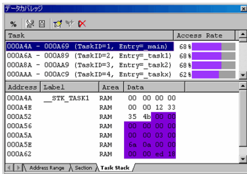
図5.124 [データカバレッジ] ウィンドウ (タスクスタック指定)
