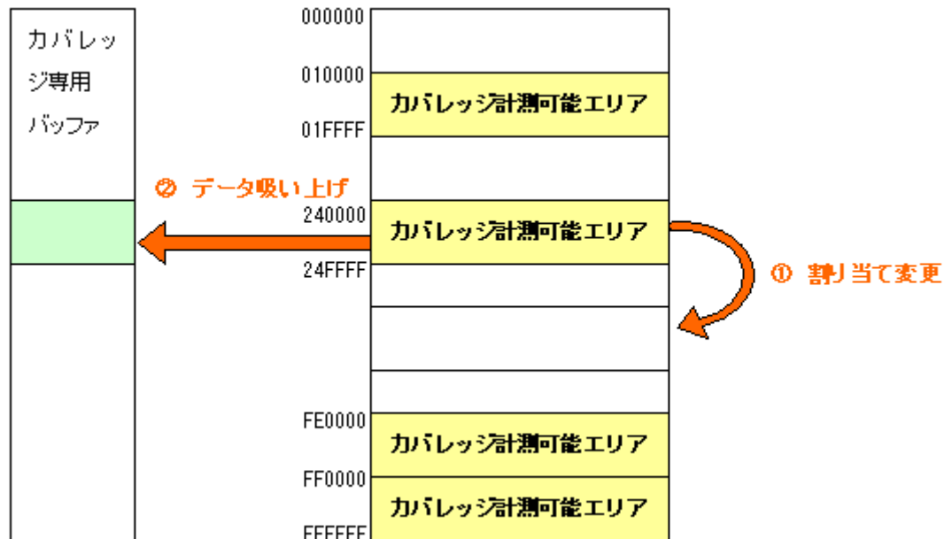
図5.106 [データカバレッジメモリ] の割り当て変更概略図
