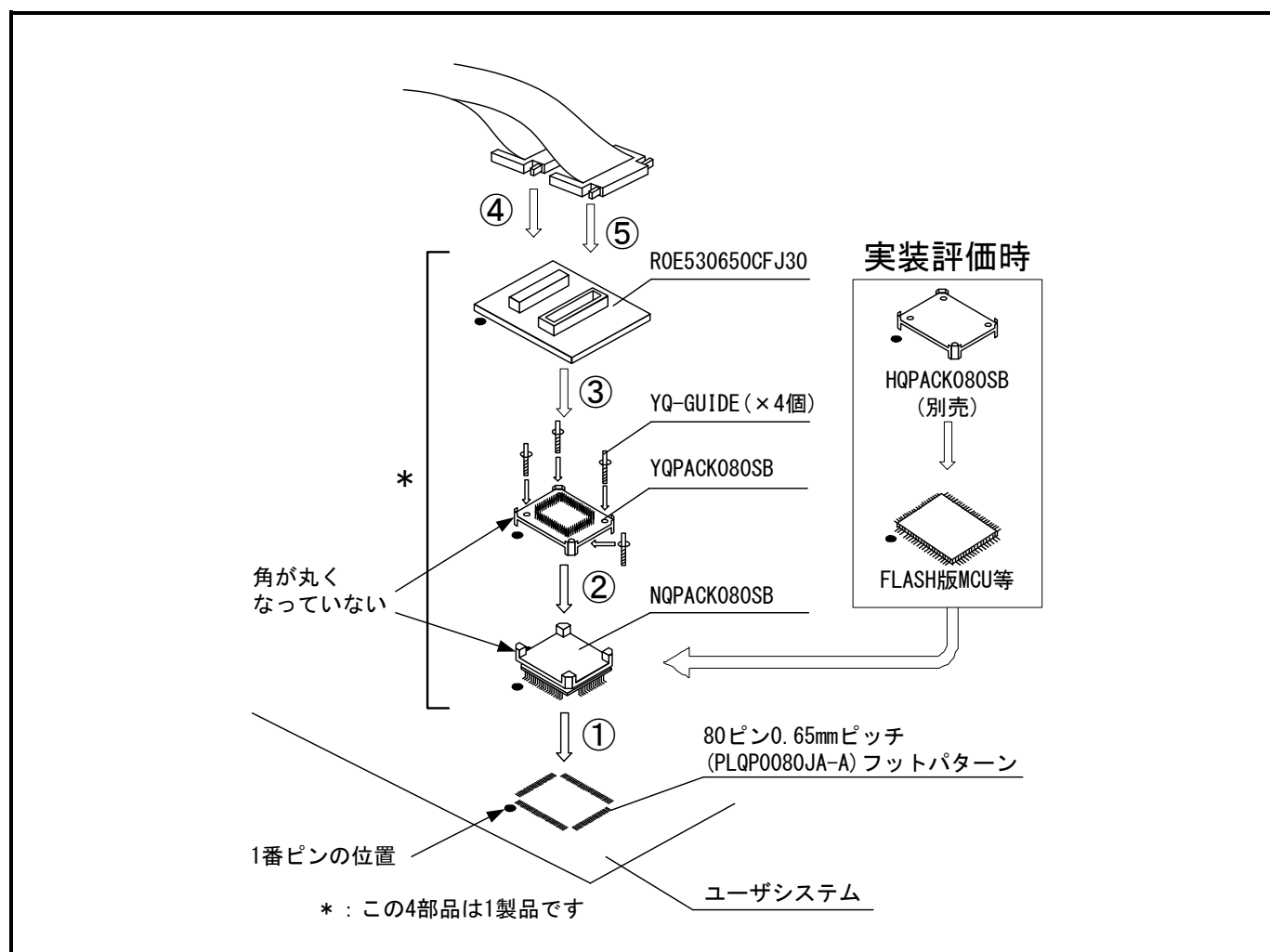
図2.13 80ピン0.65mmピッチフットパターンへの接続
