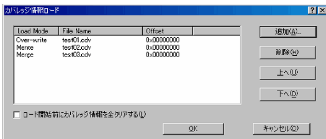
図5.127 [カバレッジ情報ロード] ダイアログボックス
