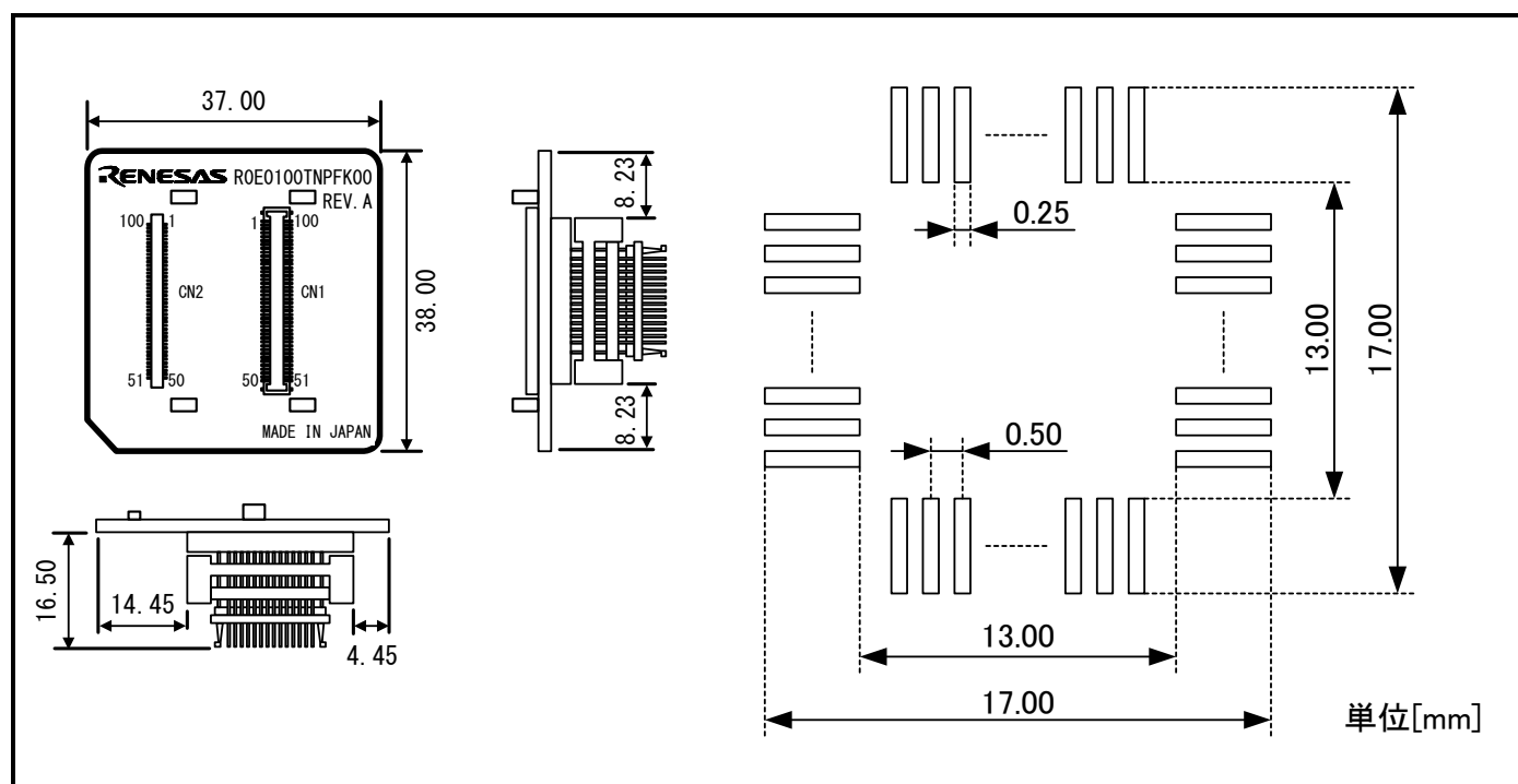
図7.4 R0E0100TNPFK00ユーザシステム接続部の寸法図および参考フットパターン
