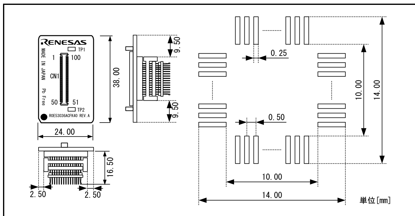
図7.4 R0E53036ACFK40ユーザシステム接続部の寸法図および参考フットパターン
