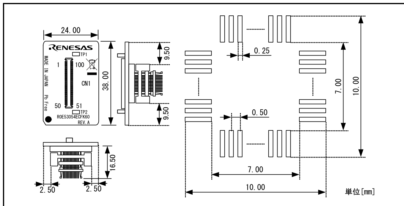
図7.3 R0E53054ECFK60ユーザシステム接続部の寸法図および参考フットパターン
