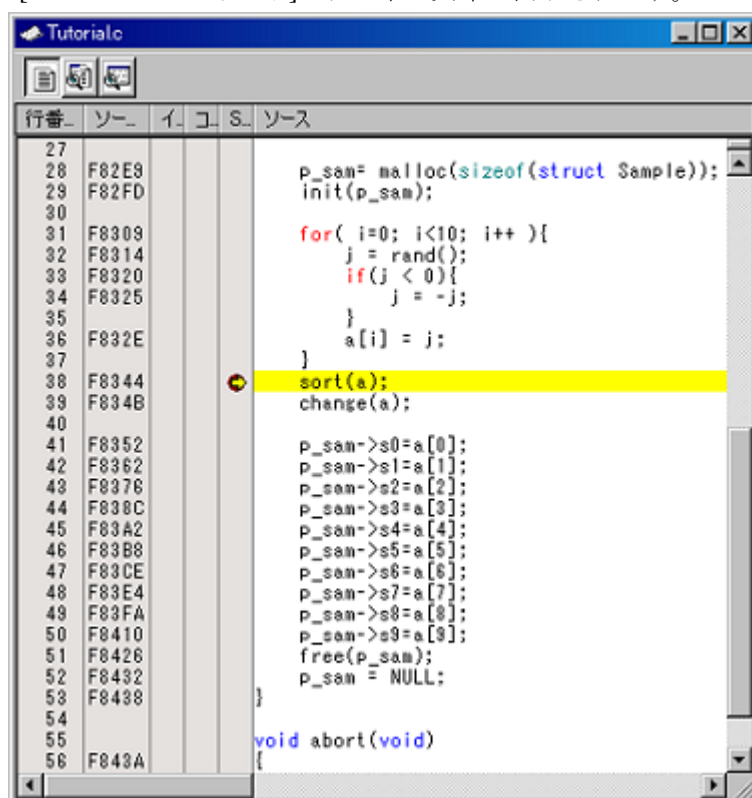
図3.5 [エディタ]ウィンドウ（ブレーク状態）
