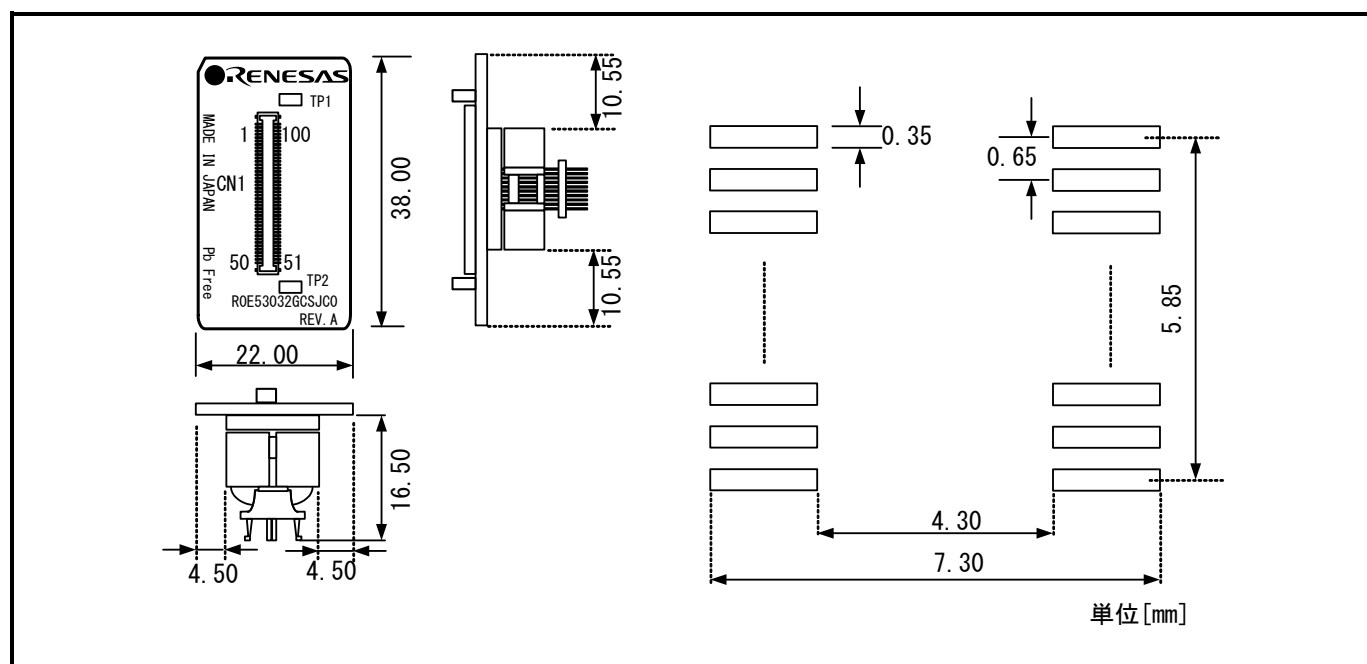
図7.4 R0E53032GCSJC0 ユーザシステム接続部の寸法図および参考フットパターン
