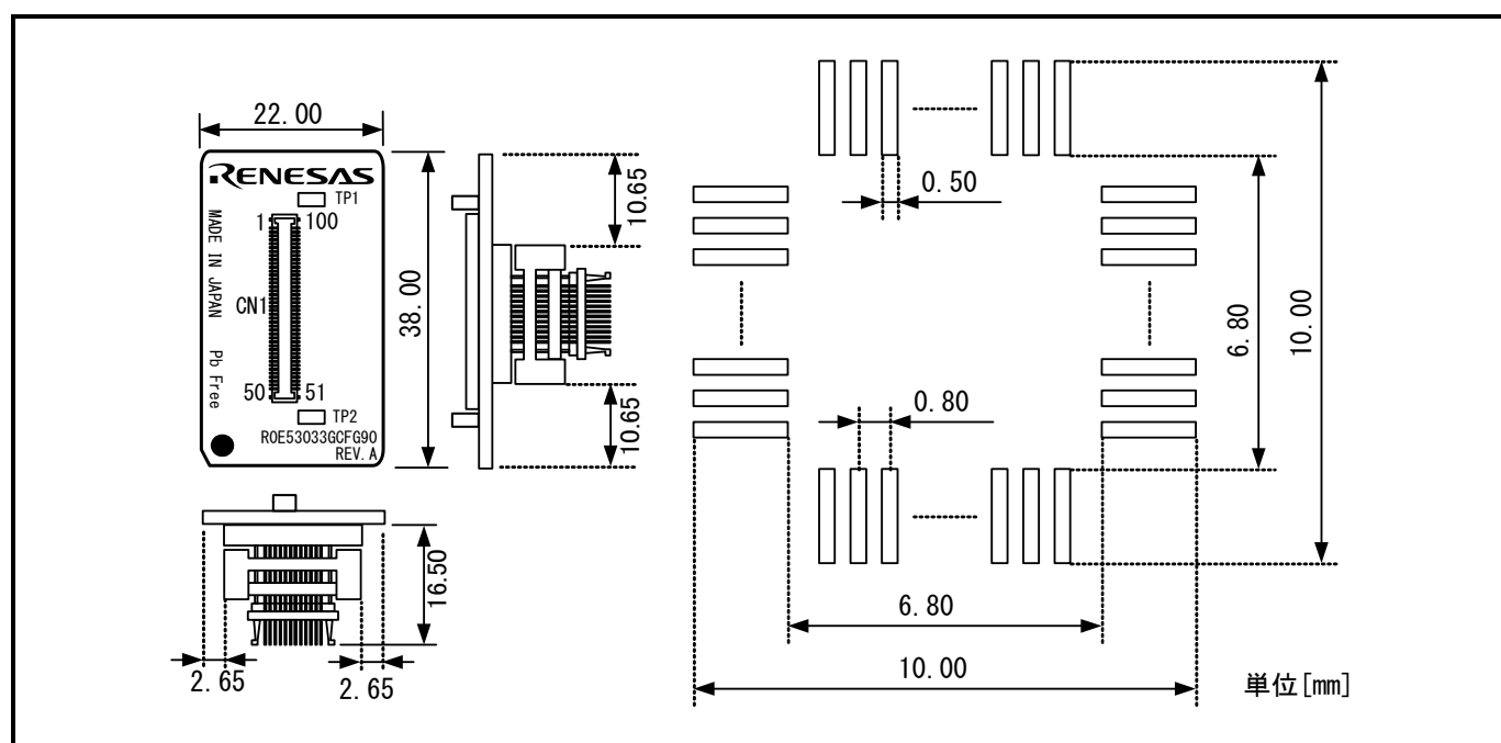
図7.6 R0E53033GCFG90ユーザシステム接続部の寸法図および参考フットパターン
