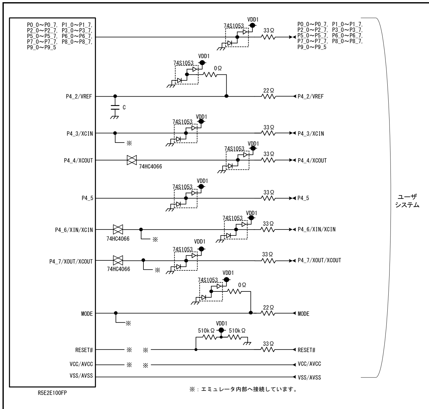
図7.1 R0E521300MCU00の接続図(一部)
