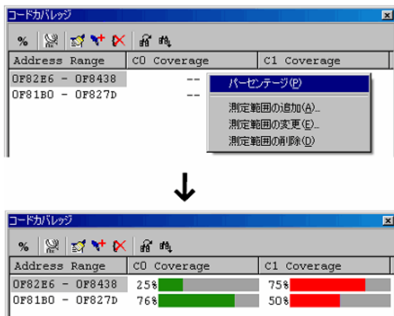
図5.92 [コードカバレッジ]ウィンドウ
