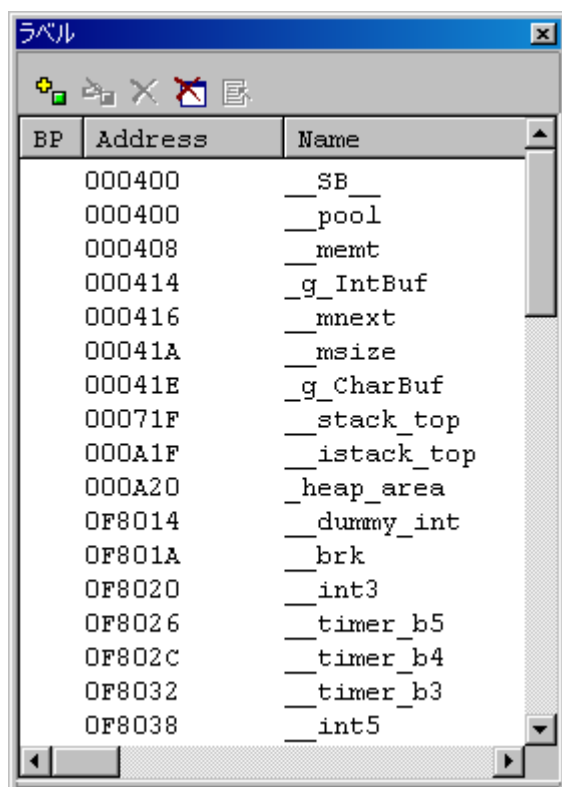
図3.10 [ラベル]ウィンドウ
