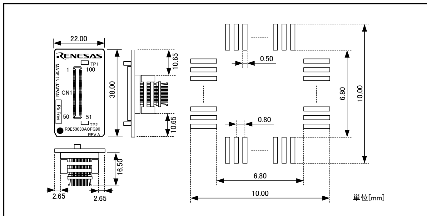
図7.5 R0E53033ACFG90ユーザシステム接続部の寸法図および参考フットパターン
