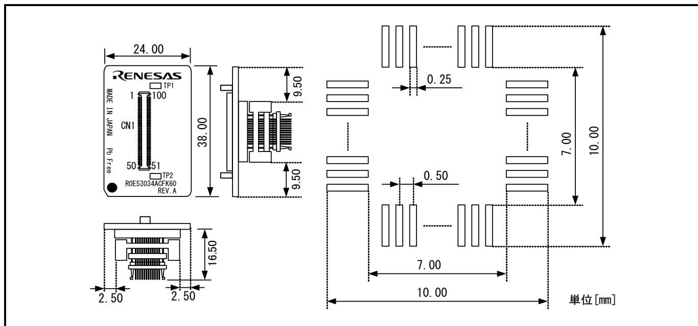
図7.7 R0E53034ACFK60ユーザシステム接続部の寸法図および参考フットパターン
