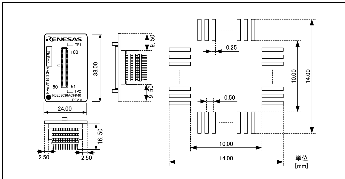
図7.10 R0E53036ACFK40ユーザシステム接続部の寸法図および参考フットパターン
