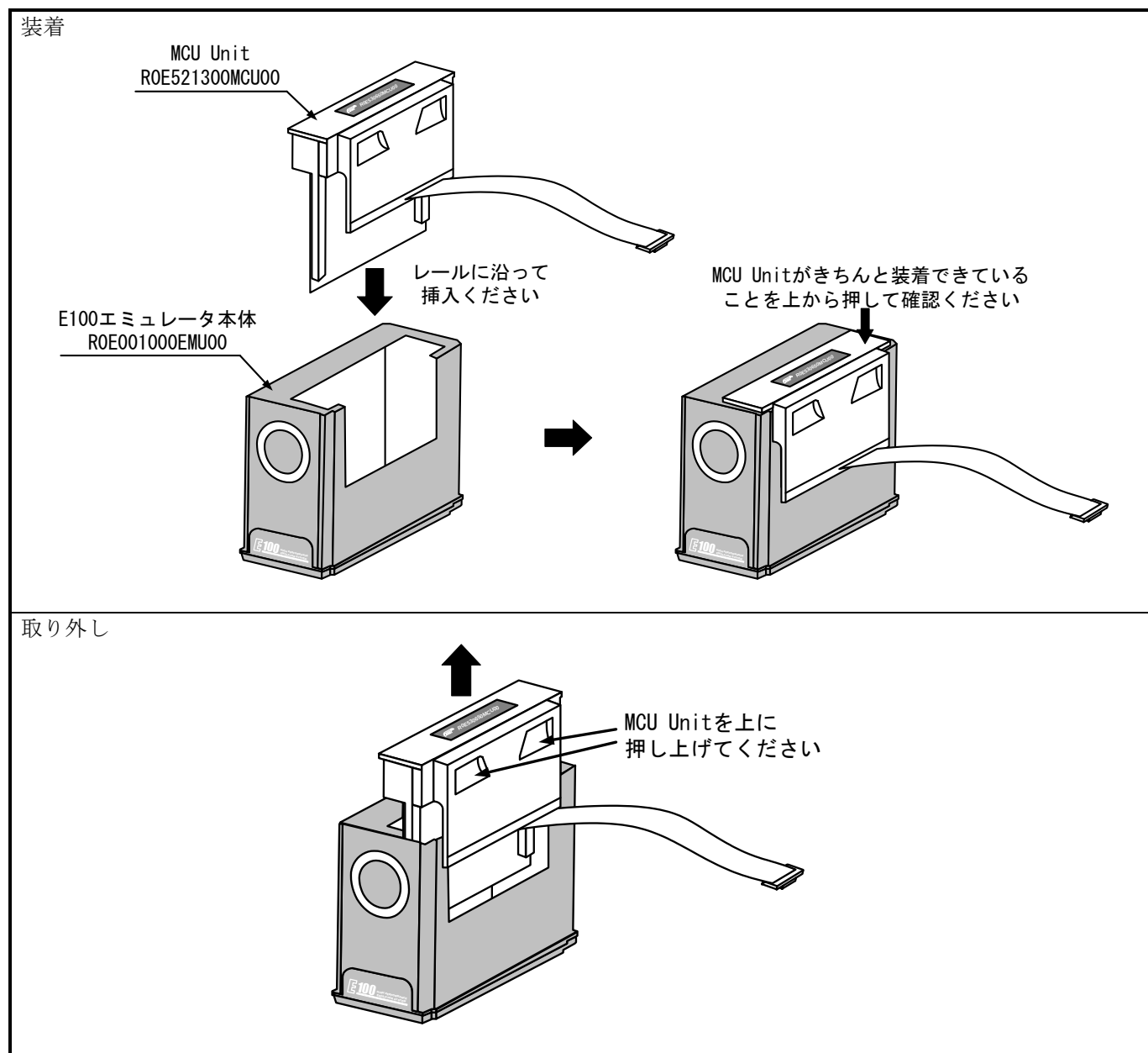
図2.3 E100エミュレータ本体とMCU Unitの着脱方法
