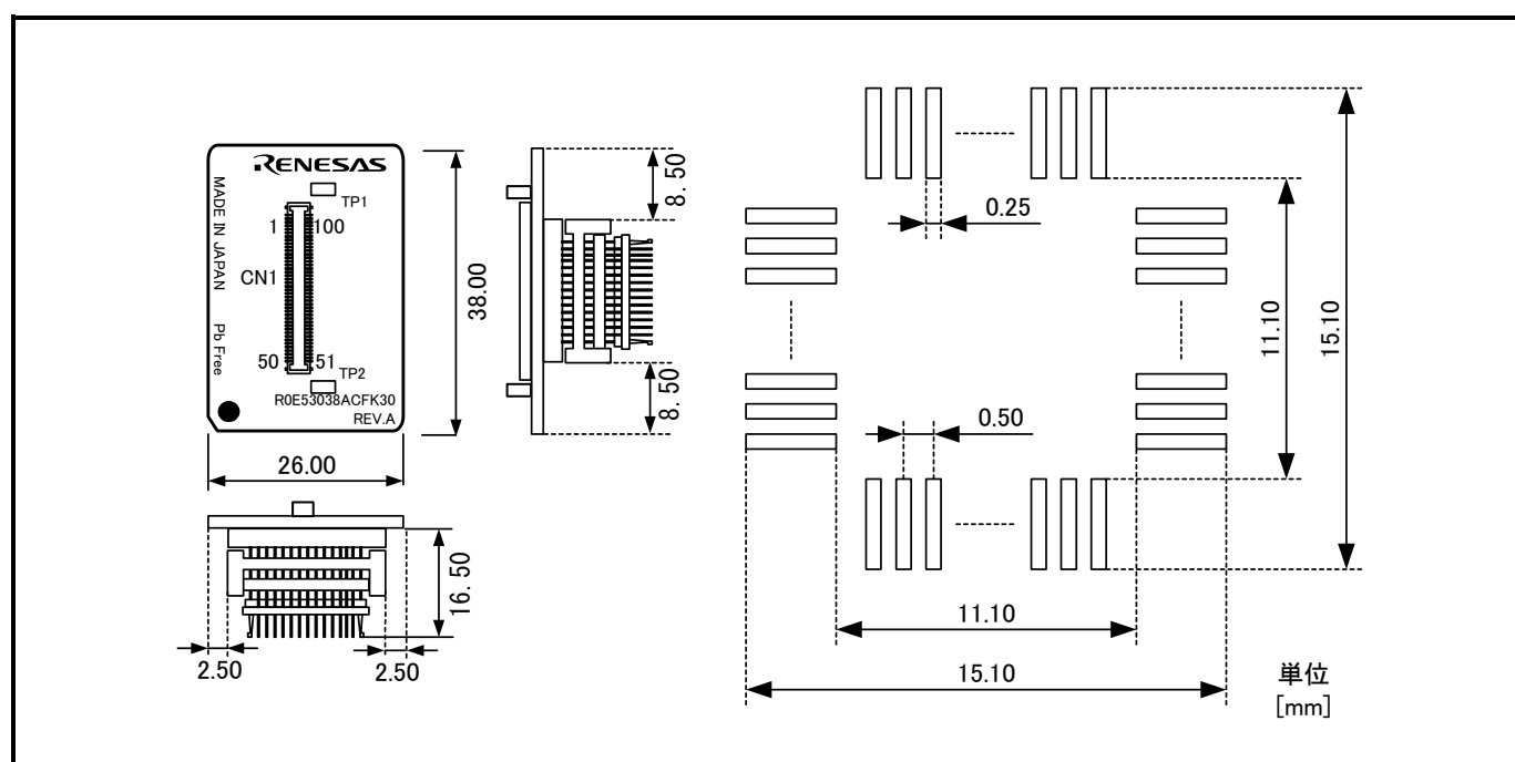
図7.12 R0E53038ACFK30ユーザシステム接続部の寸法図および参考フットパターン
