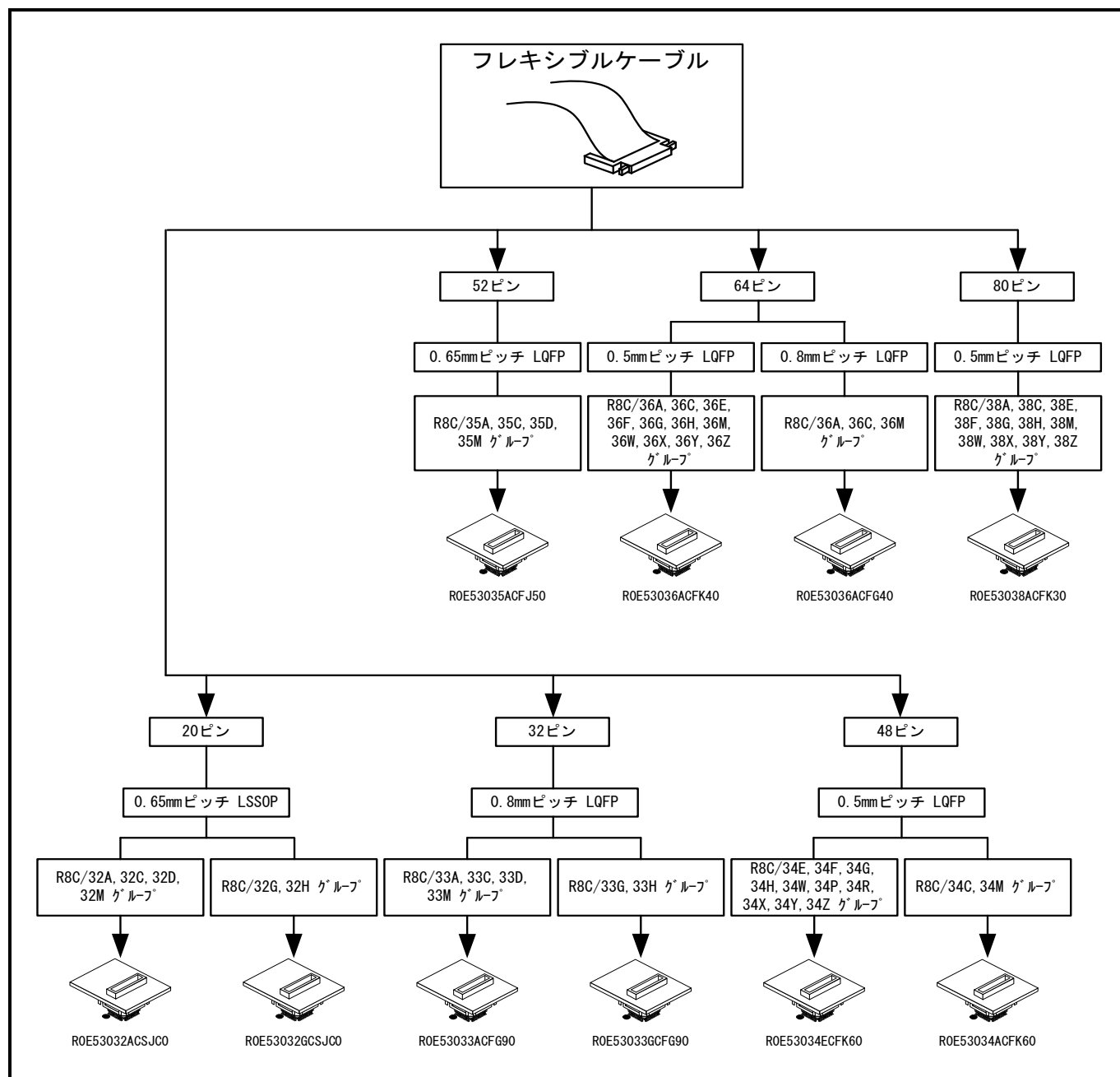
図2.10 本製品とユーザシステムとの接続
