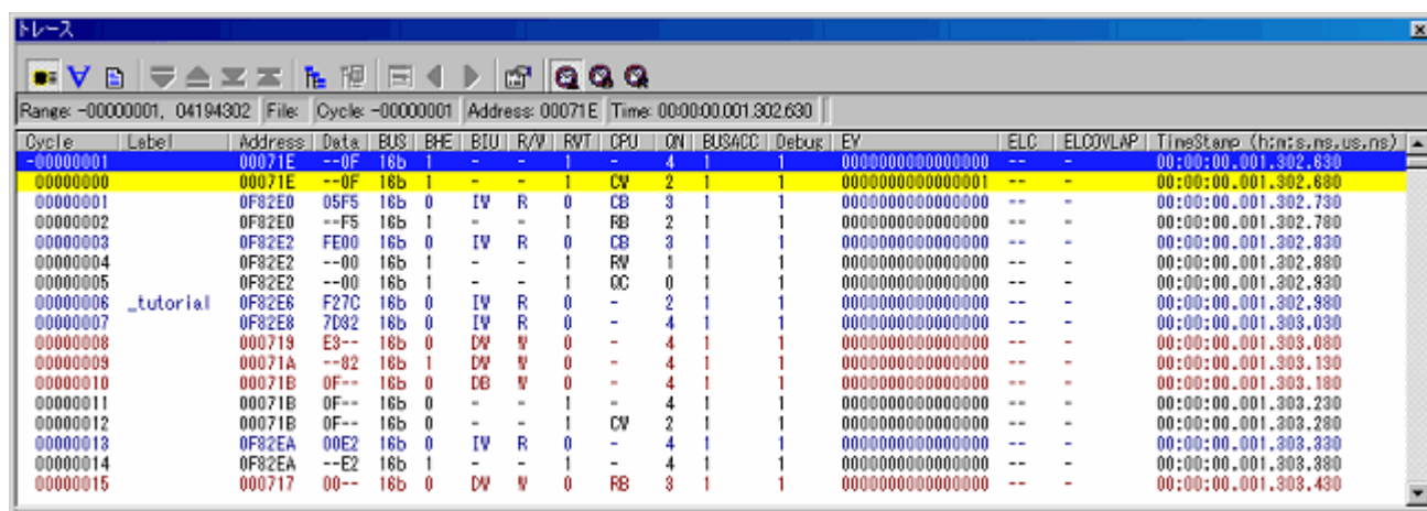
図3.36 [トレース]ウィンドウ (ポイント&ディレイ)
