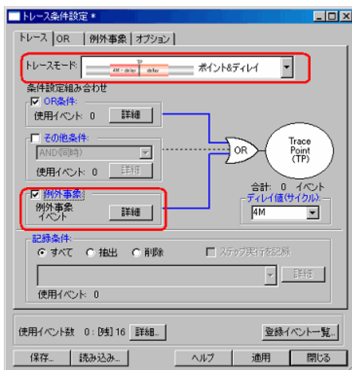
図5. 142 [トレース条件設定]ダイアログボックス
