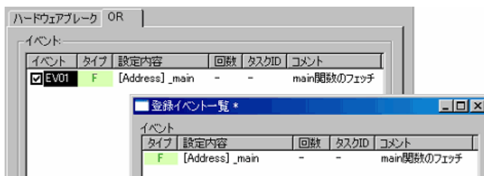
図5.37 [ハードウェアブレーク条件設定]ダイアログボックスと[登録イベント一覧]ダイアログボックス
