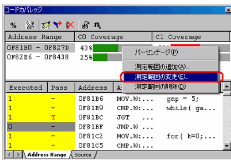
図5.79 [コードカバレッジ]ウィンドウ
