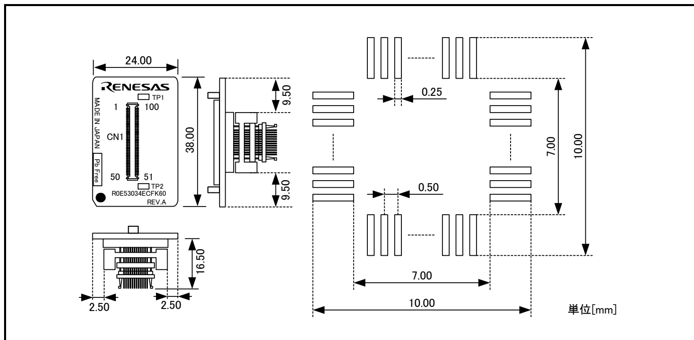
図7.8 R0E53034ECFK60ユーザシステム接続部の寸法図および参考フットパターン
