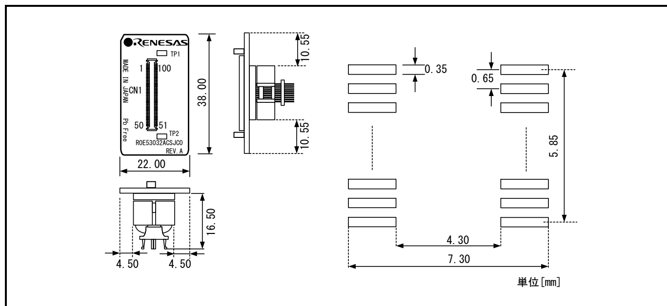
図7.3 R0E53032ACSJC0 ユーザシステム接続部の寸法図および参考フットパターン
