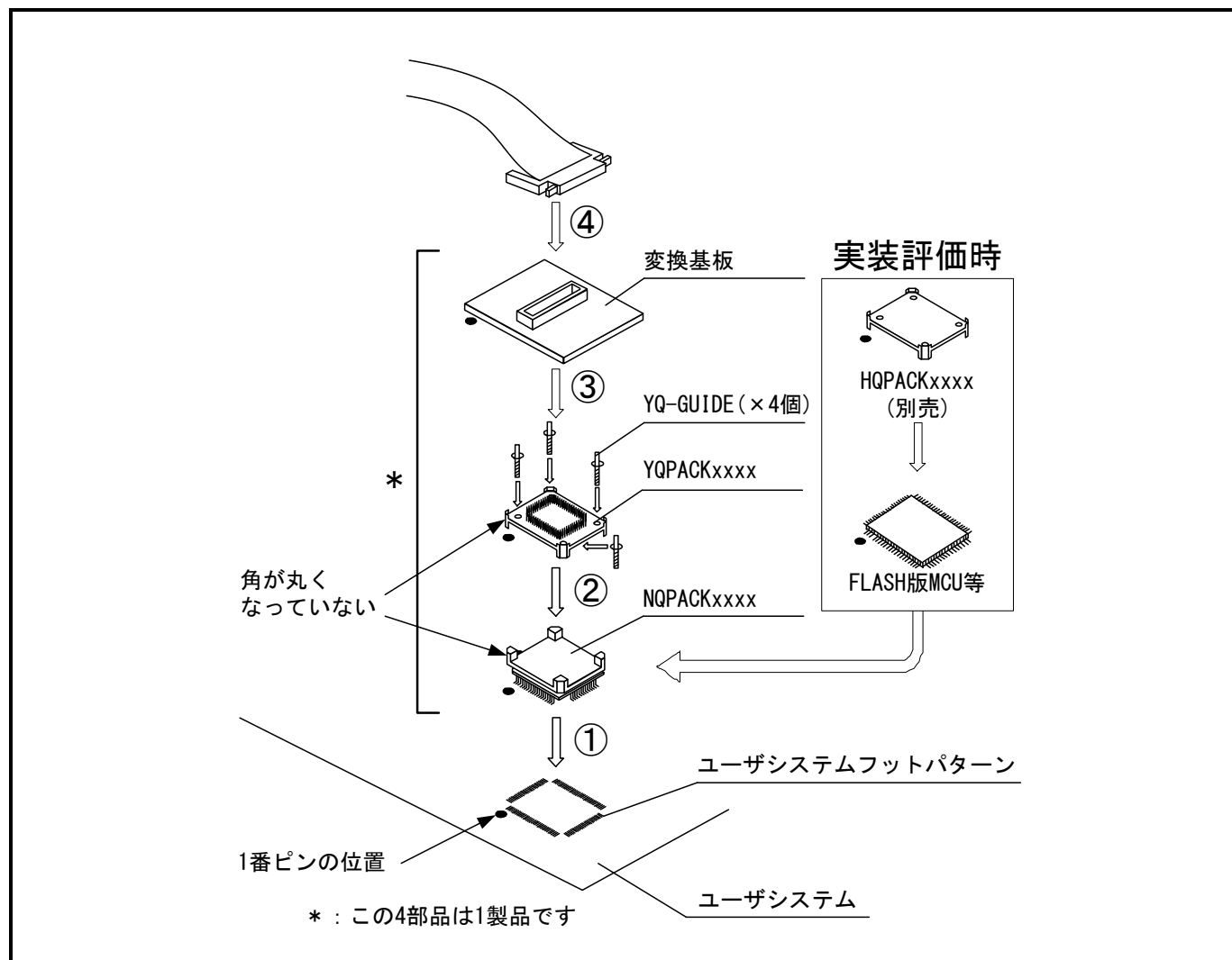
図2.11 ユーザシステムへの接続
