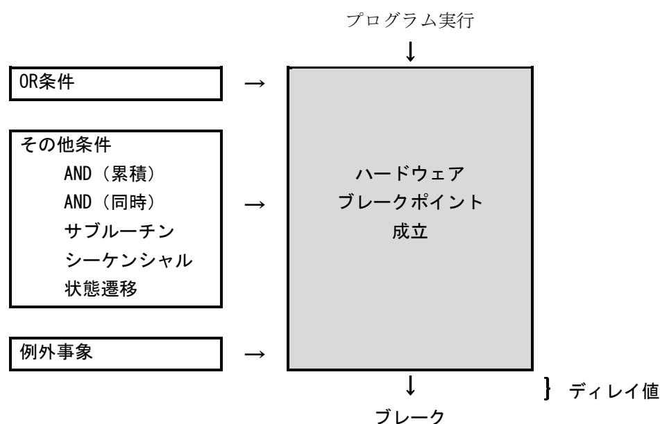
図5.41 ハードウェアブレイク概要
