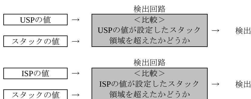
図5.145 スタックアクセス違反検出方法の概要
