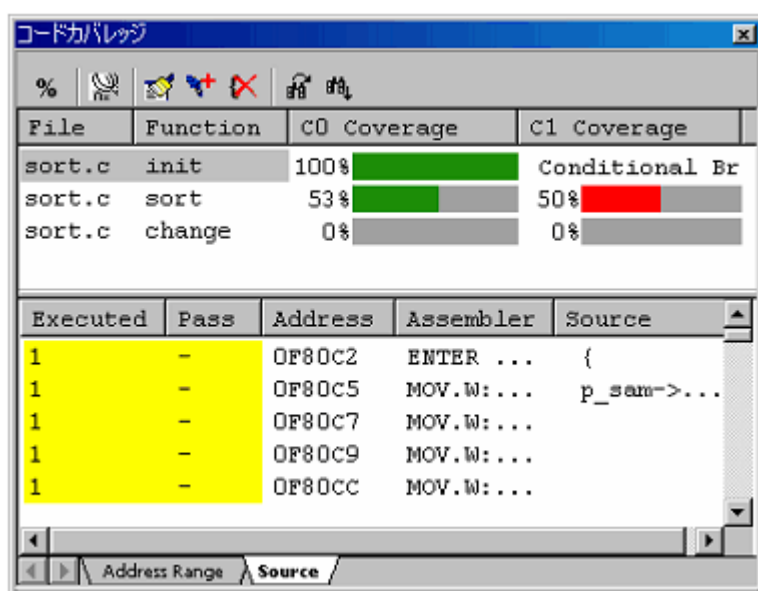
図5.85 [コードカバレッジ]ウィンドウ
