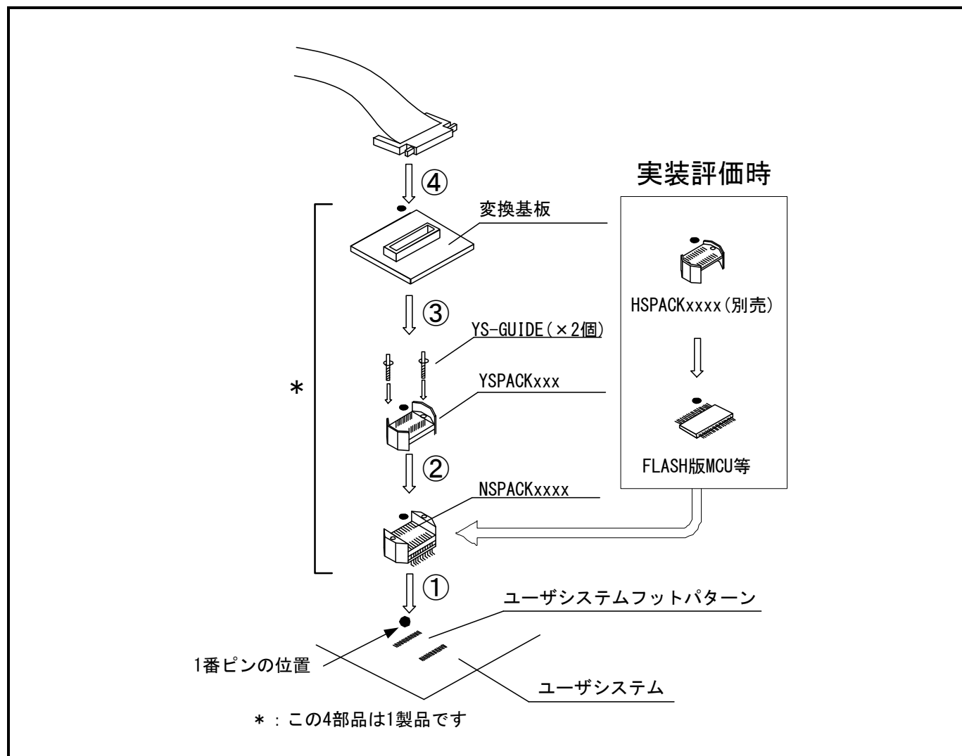
図2.12 ユーザシステムへの接続
