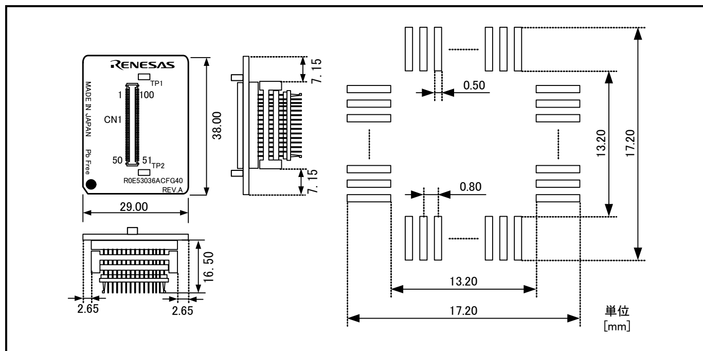
図7.11 R0E53036ACFG40ユーザシステム接続部の寸法図および参考フットパターン
