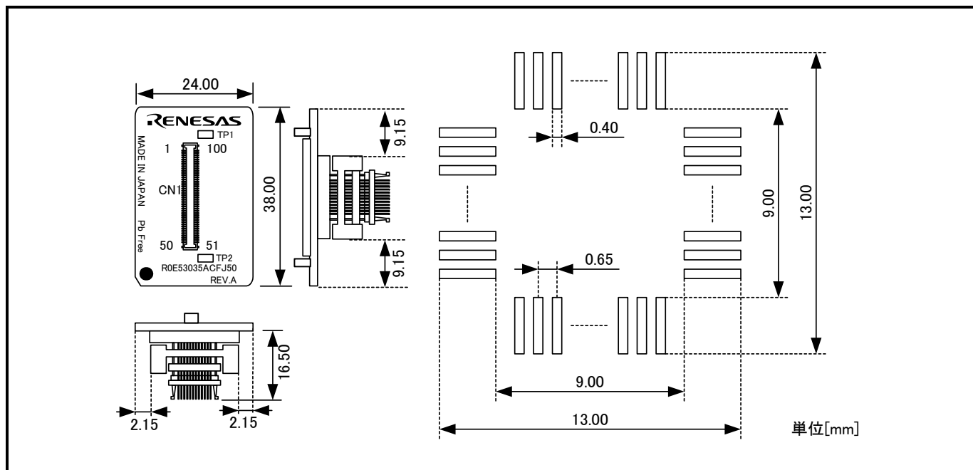
図7.9 R0E53035ACFJ50ユーザシステム接続部の寸法図および参考フットパターン
