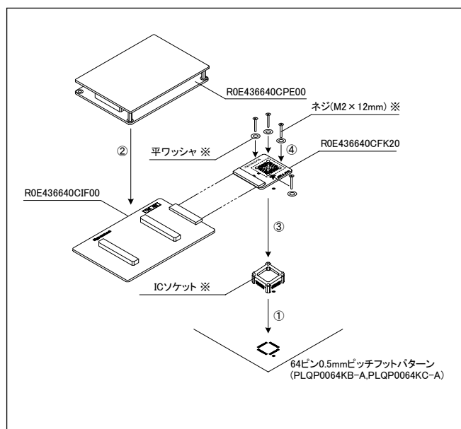
図3 R0E436640CFK20の装着手順
