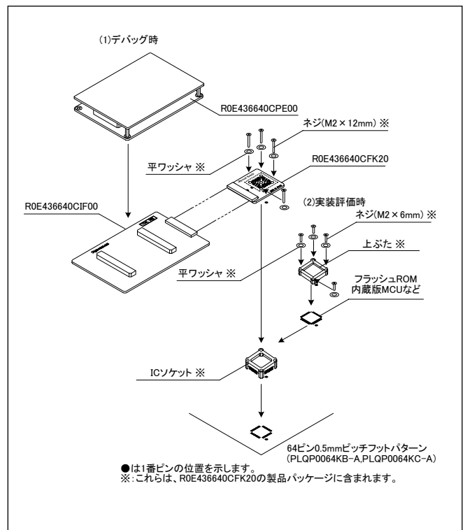
図2 R0E436640CFK20の使用方法
