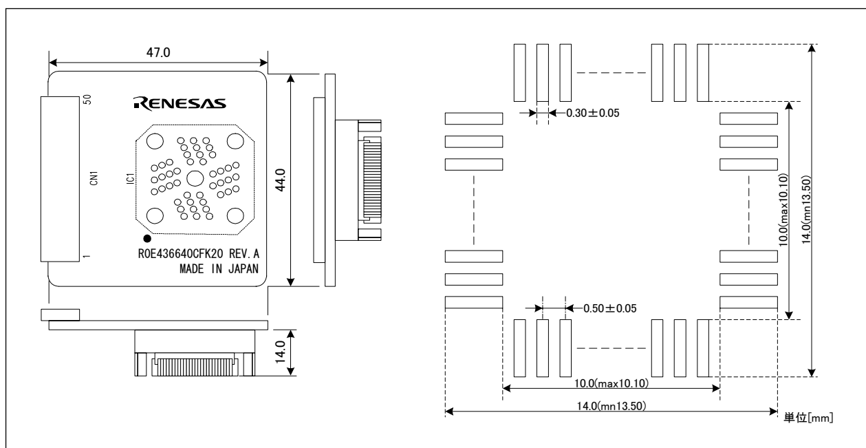
図4 R0E436640CFK20ターゲット接続部の寸法図および推奨フットパターン
