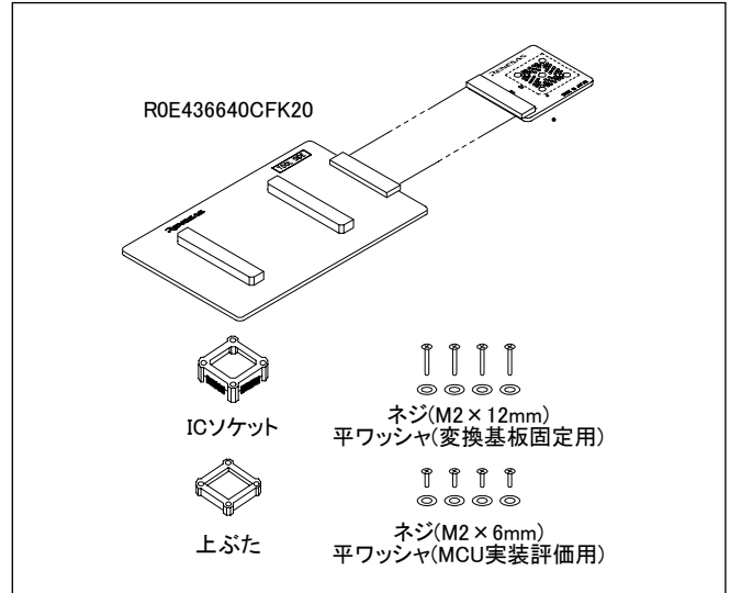
図1 R0E436640CFK20の製品内容
