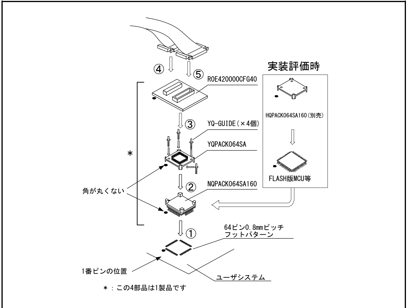
図2.13 64ピン0.8mmピッチフットパターンへの接続
