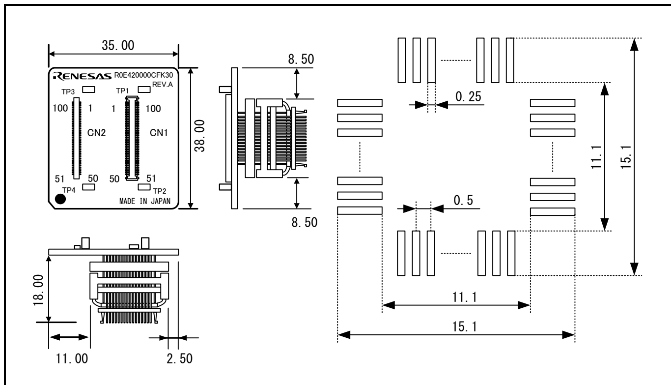
図7.4 R0E420000CFK30ユーザーシステム接続部の寸法図および参考フットパターン
