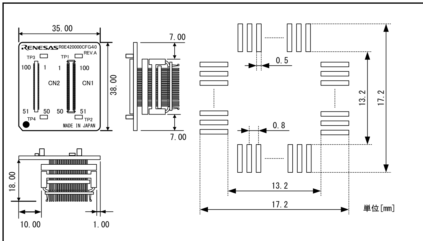
図7.5 R0E420000CFG40ユーザーシステム接続部の寸法図および参考フットパターン
