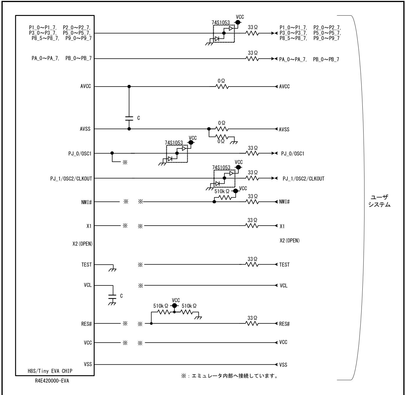
図 7.1 R0E420000MCU00の接続図(一部)
