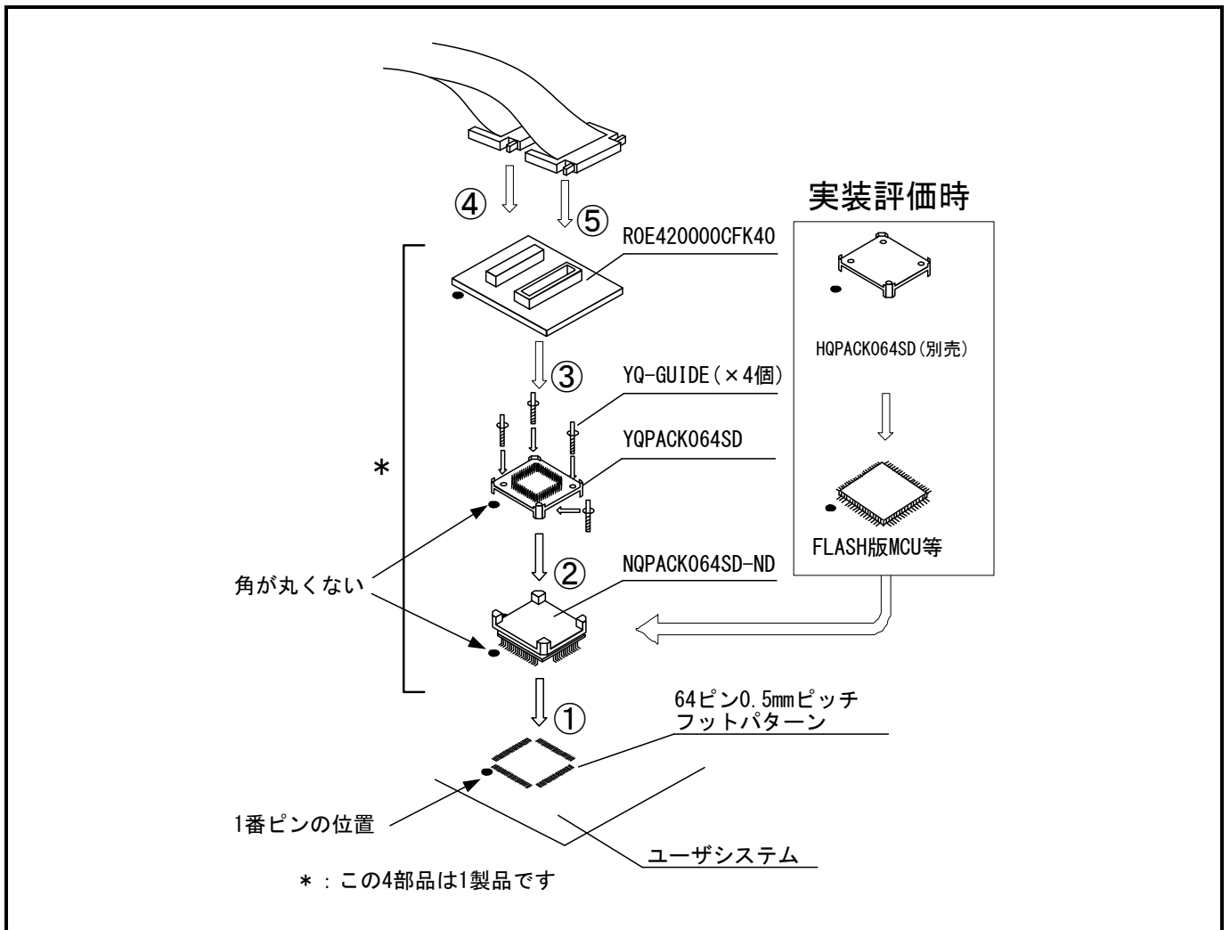
図2.14 64ピン0.5mmピッチフットパターンへの接続
