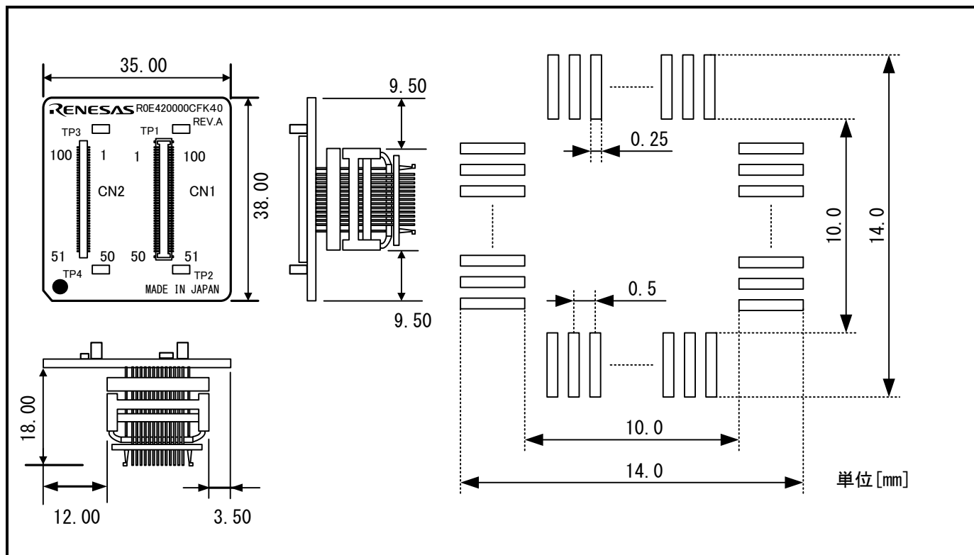
図7.6 R0E420000CFK40ユーザーシステム接続部の寸法図および参考フットパターン
