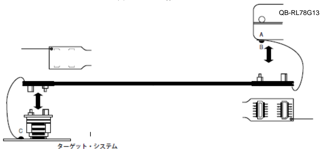
図2-8 GND線
