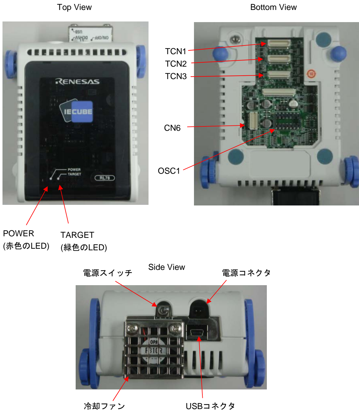
図1-1 QB-RL78G13の各部の名称
