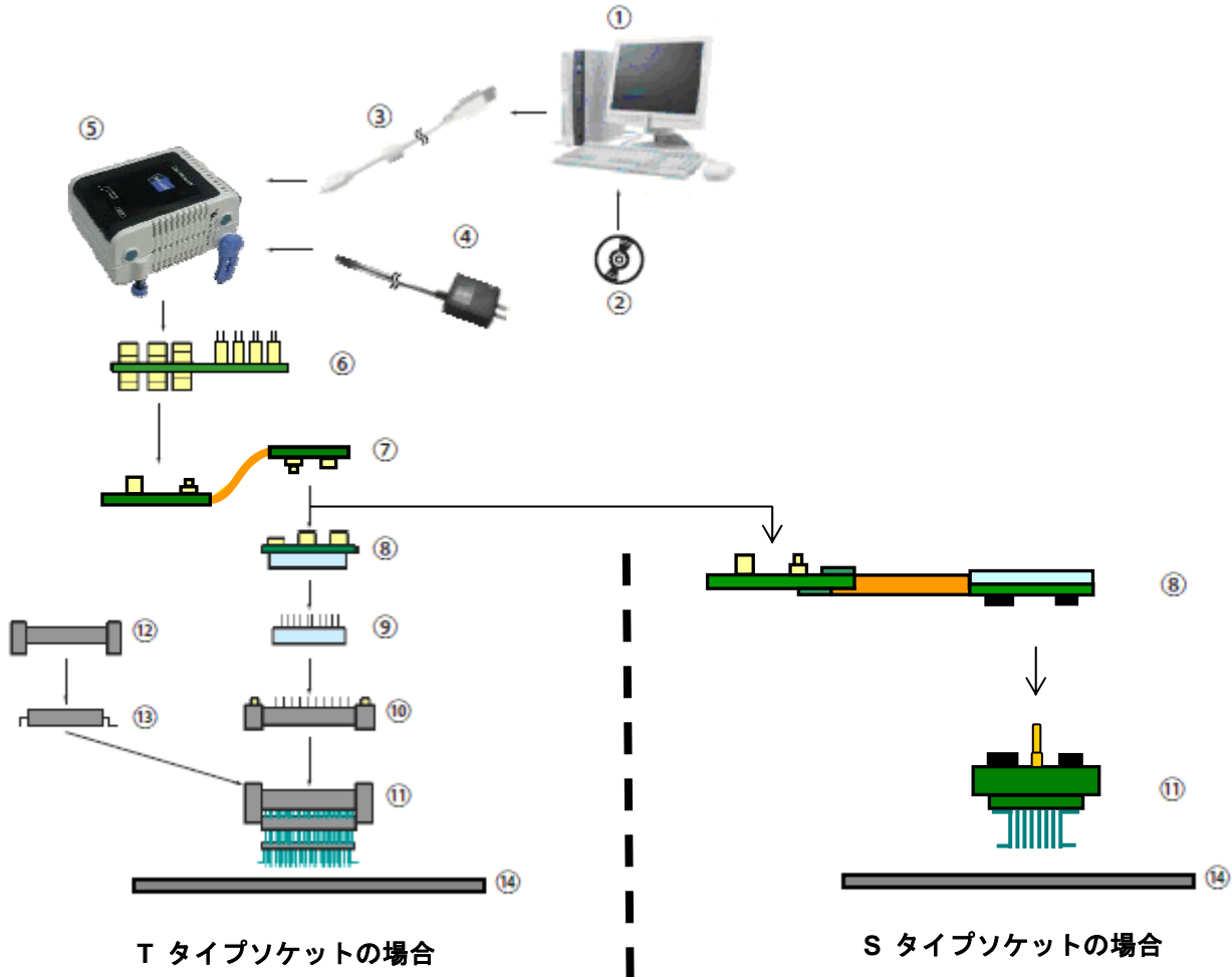
図1-2 システム構成
