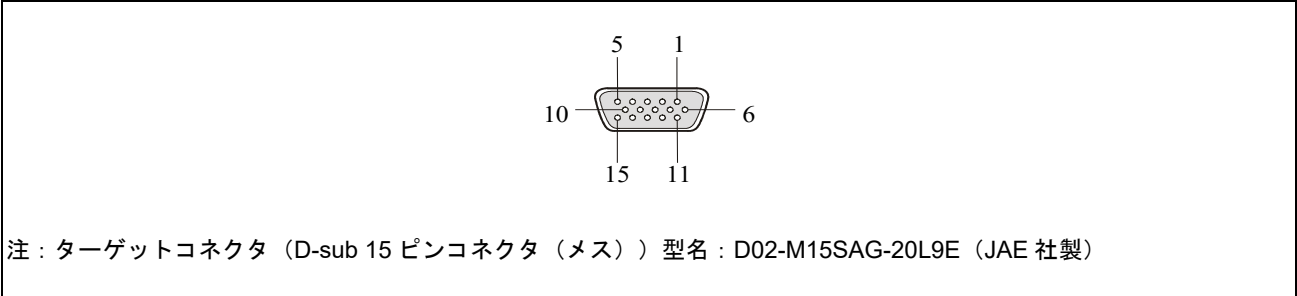
図10.9 ターゲットコネクタ（D-sub 15 ピンコネクタ（メス））のピン配置
