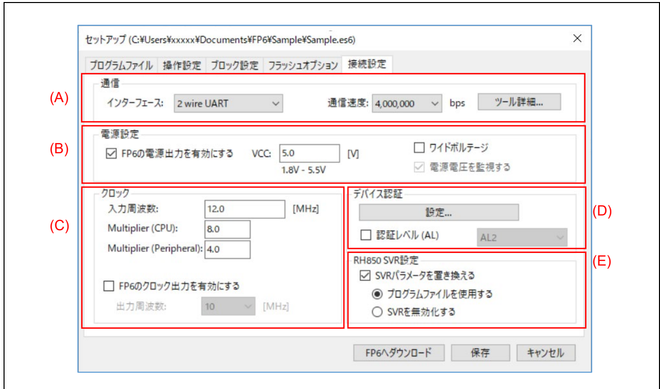
図 4.11 [接続設定]タブ
