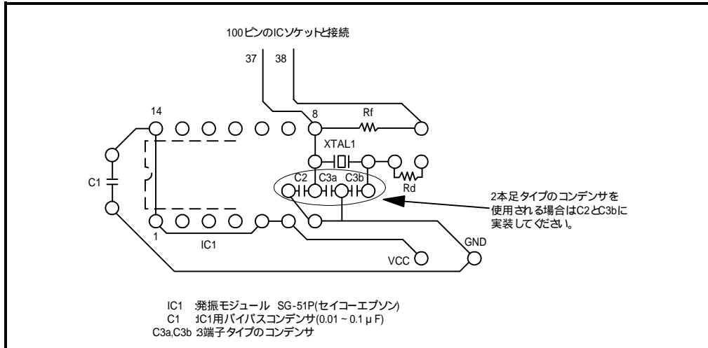
図1 発振回路パターン
