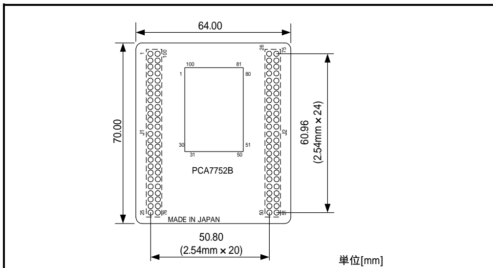
図2 PCA7752B寸法図
