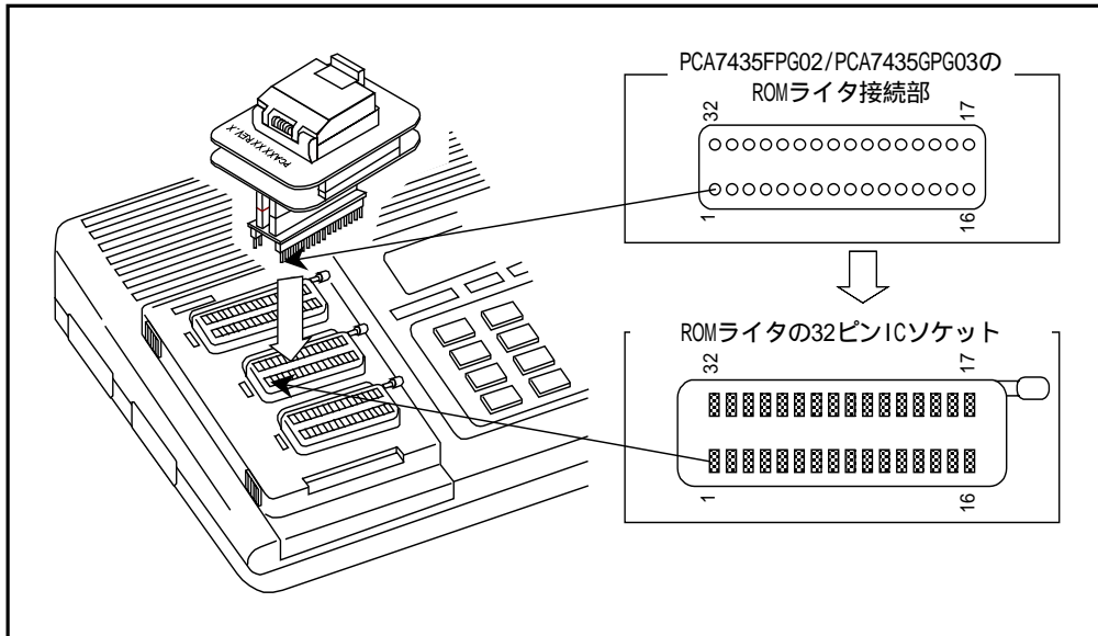
図 4.1 ROMライターへのセット方法(PCA7435FPG02/PCA7435GPG03 の場合)
