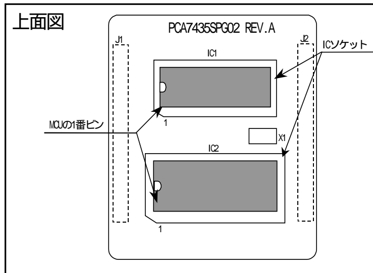
図 4.4 MCU のセット方法(PCA7435SPG02 の場合)
