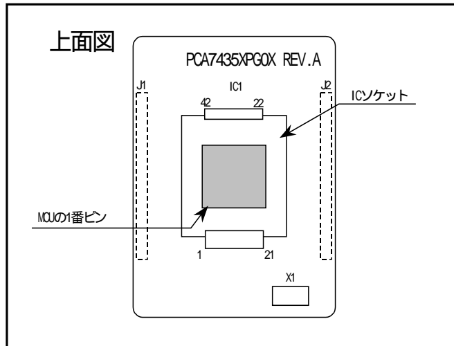
図 4.3 MCU のセット方法(PCA7435FPG02/PCA7435GPG03 の場合)
