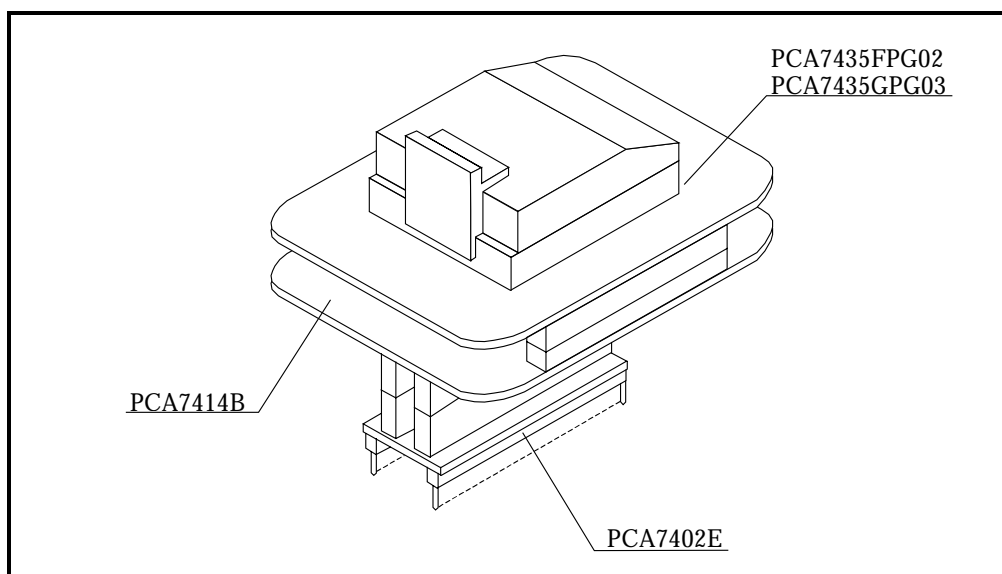
図 2.1 外形と構成部品(PCA7435FPG02/PCA7435GPG03 の場合)
