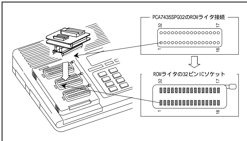
図 4.2 ROMライターへのセット方法(PCA7435SPG02 の場合)
