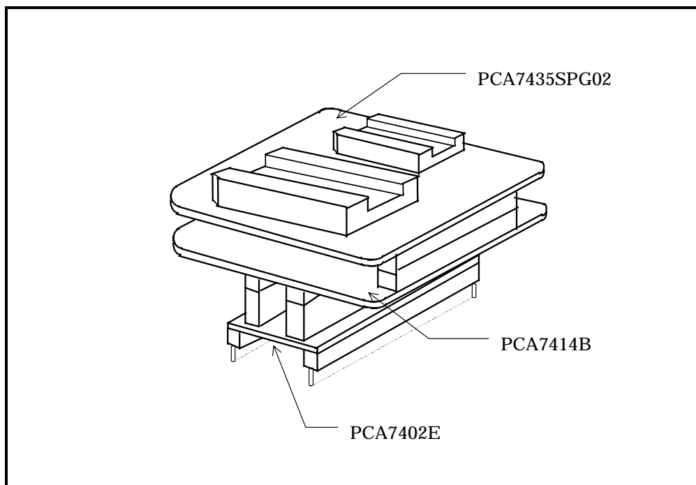
図 2.2 外形と構成部品(PCA7435SPG02 の場合)
