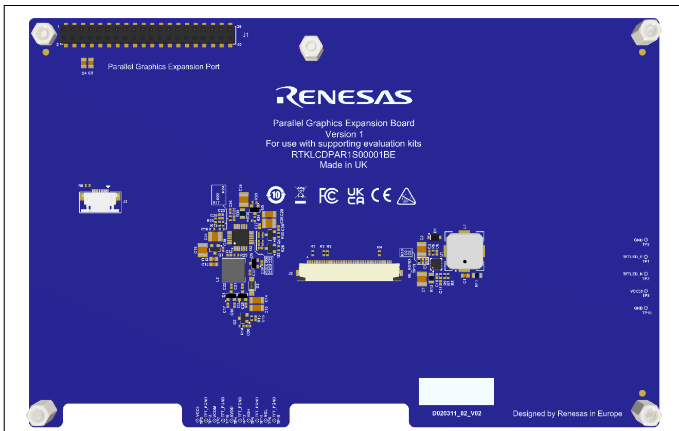
図 2. パラレルグラフィックス拡張ボード 1 (裏面)
