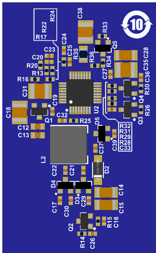
図 8. 車載グレード TFT-LCD 電源
