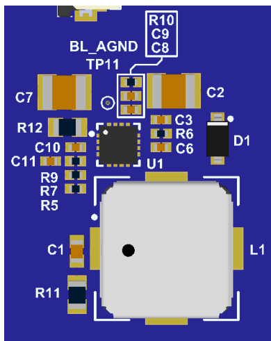
図 7. LCD バックライトコントローラ
