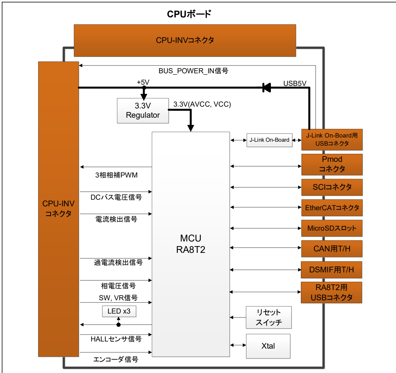
図 4-1 CPU ボードのブロック図
