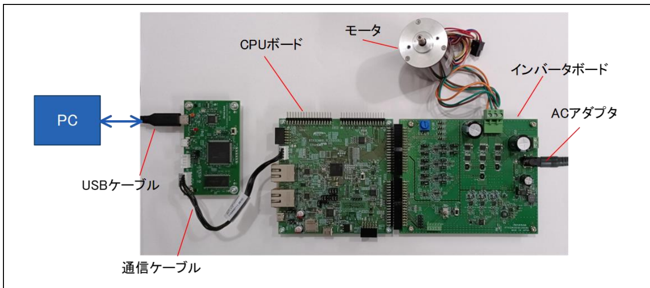
図 4-5 ボード接続例
