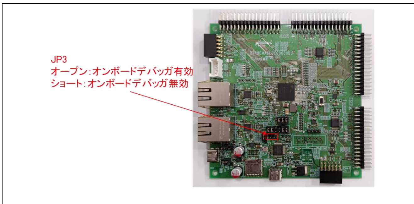
図 5-1 ジャンパーJP3 の設定
