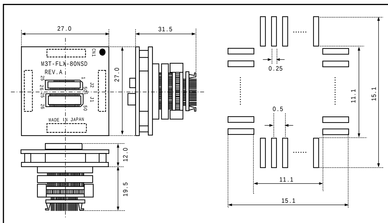
図4 M3T-FLX-80NSD寸法図及び参考フットパターン
