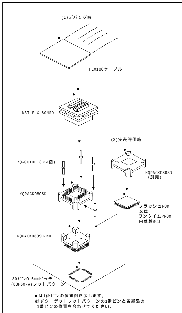
図2 M3T-FLX-80NSDの用途
