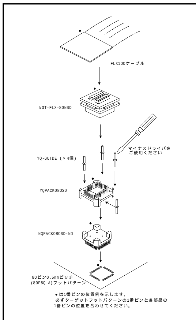
図3 M3T-FLX-80NSD装着手順
