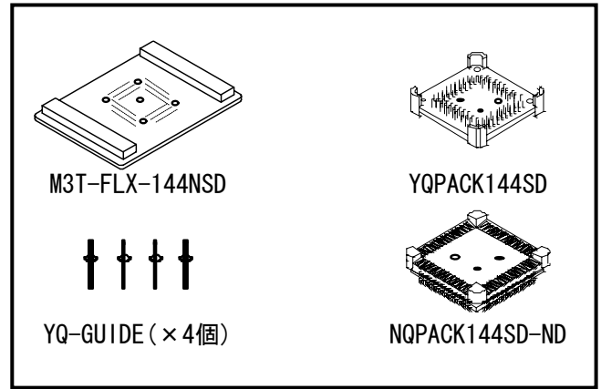
図1 M3T-FLX-144NSDの製品内容
