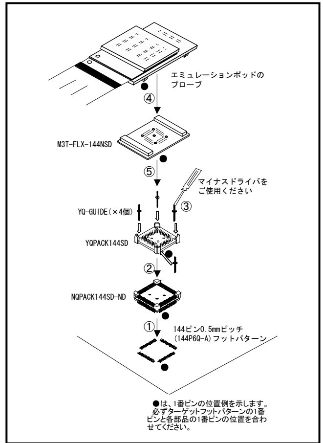
図3 M3T-FLX-144NSD装着手順
