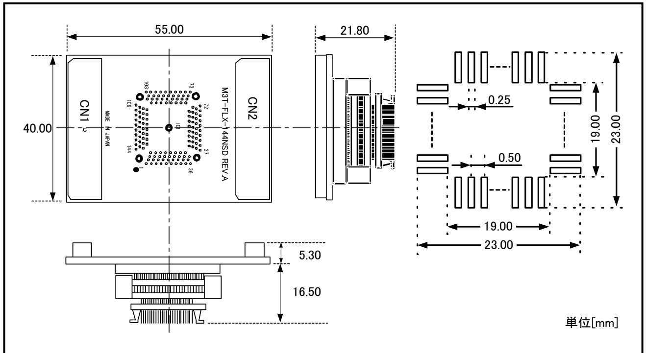
図4 M3T-FLX-144NSD寸法図及び参考フットパターン
