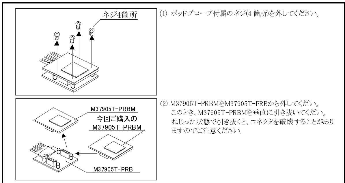
図1 MCU基板の交換方法
