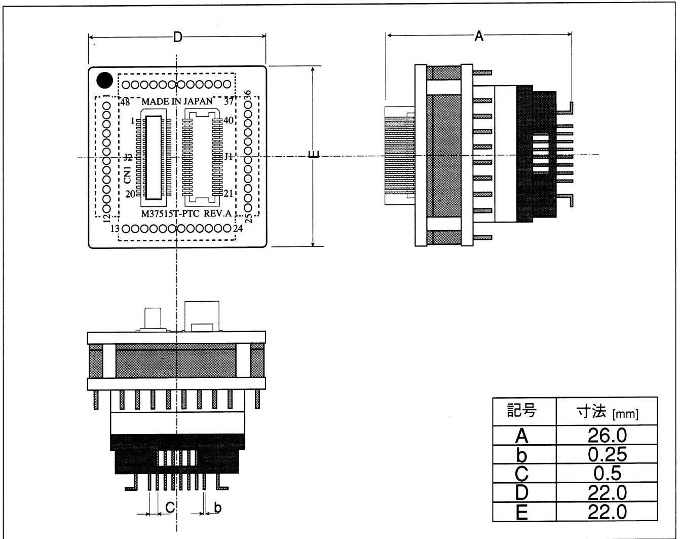
図4 M37515T-PTCの寸法
