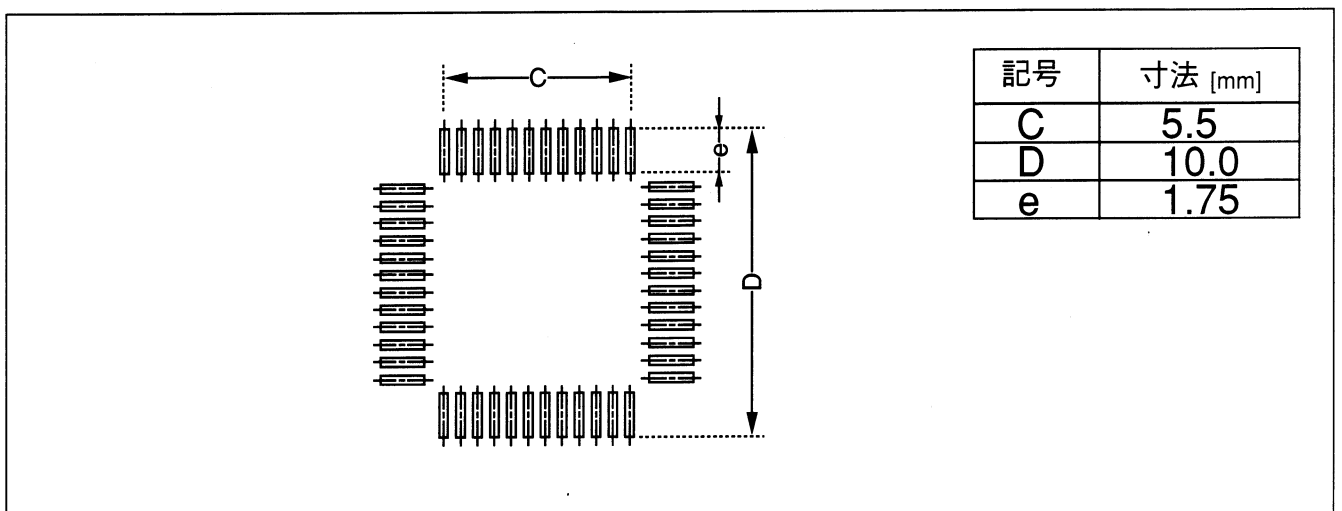
図5 ターゲットフットパターン寸法(東京エレテック TQPACK製品一覧表より転載しています。)
