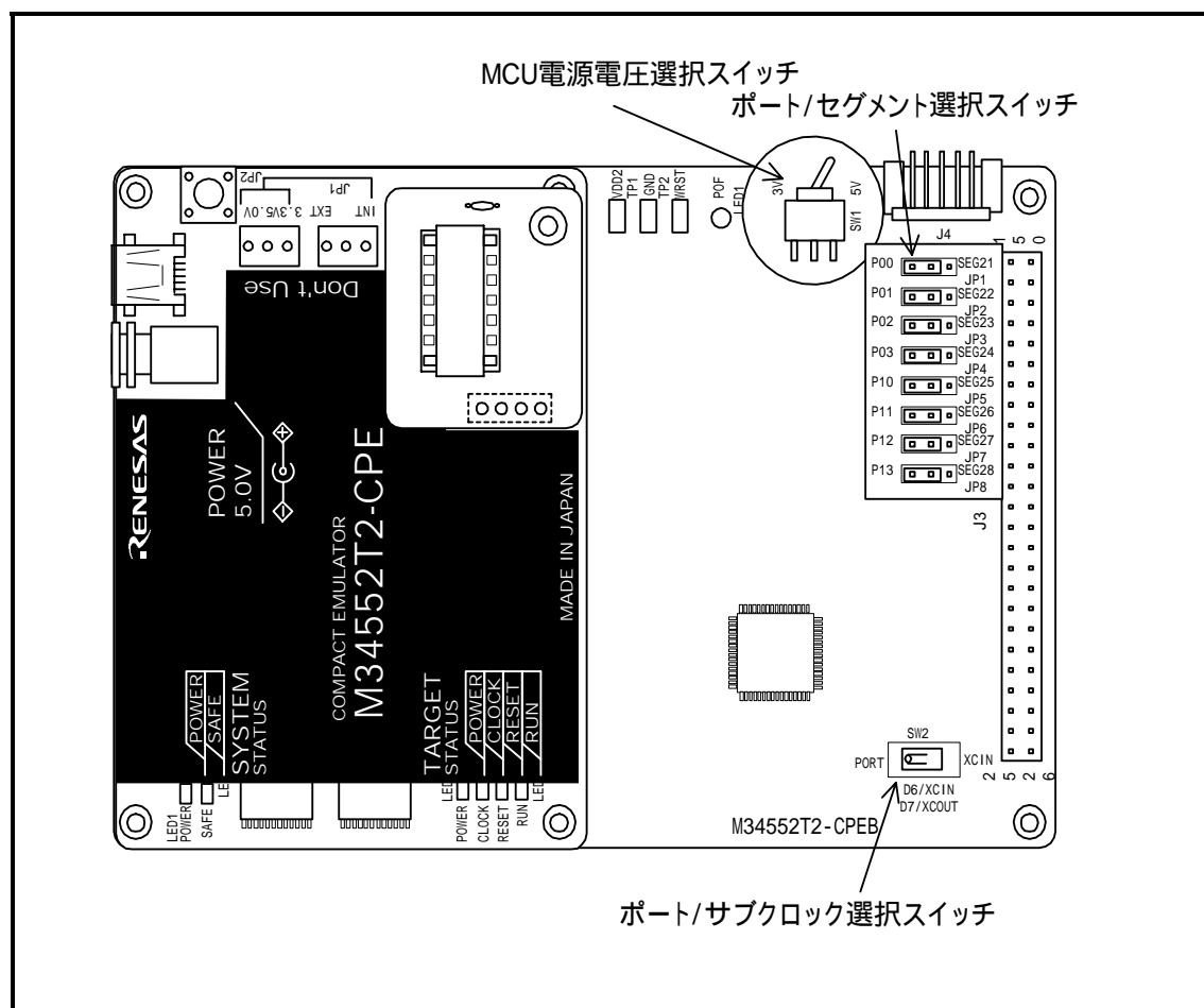
図 2.5 エミュレータのスイッチ位置
