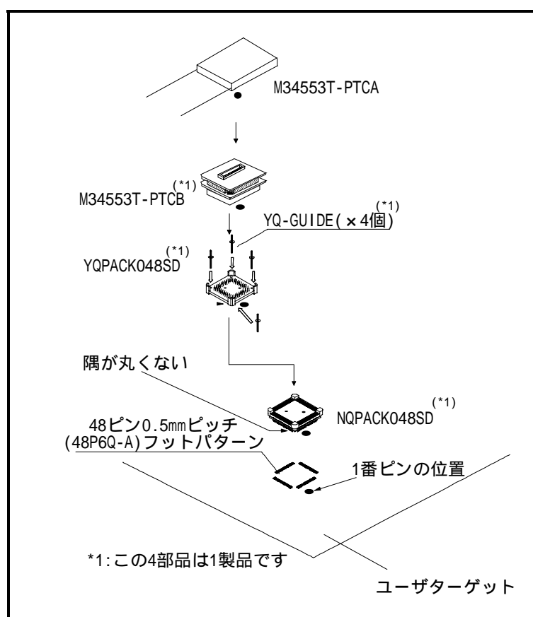
図 2.14 48ピン0.5mmピッチLQFPパッケージフットパターンとの接続
