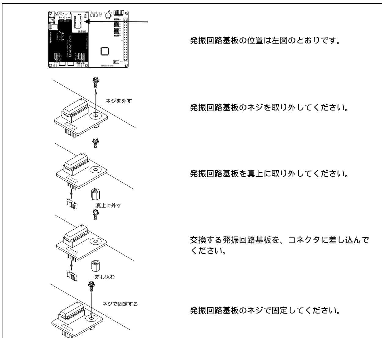
図 2.15 発振回路基板の交換手順
