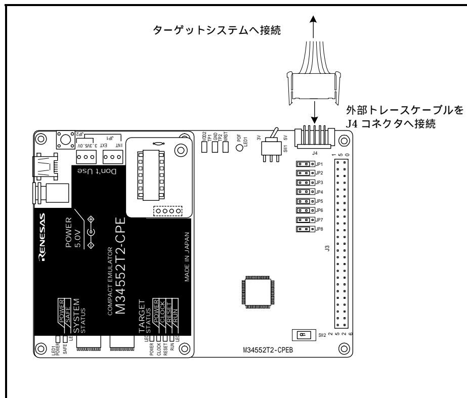
図 2.18 外部トレース/トリガケーブルの接続
