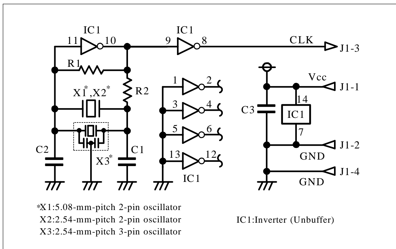
図 2.17 発振回路基板ペアボードOSC-2の回路図
