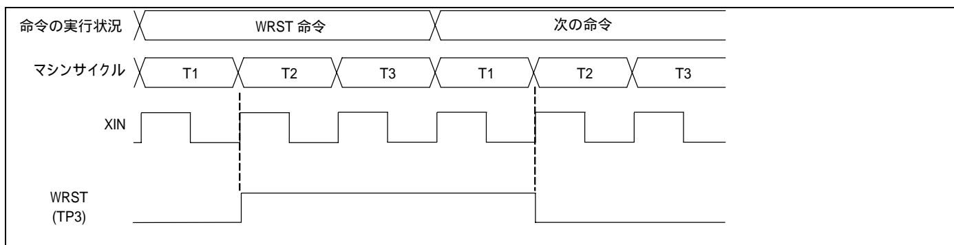
図 2.23 チェック端子WRSTの出力波形
