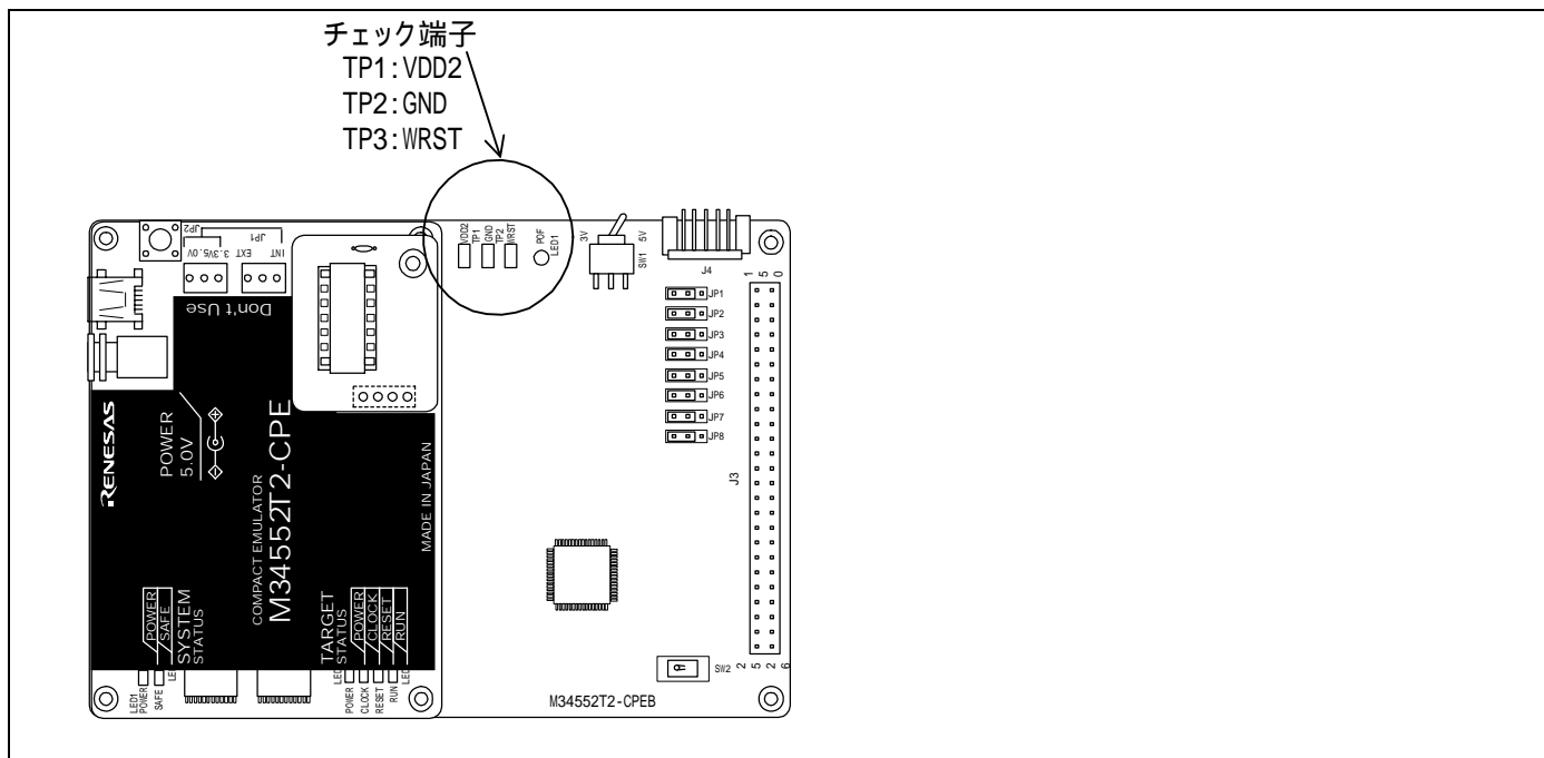
図 2.22 チェック端子の位置
