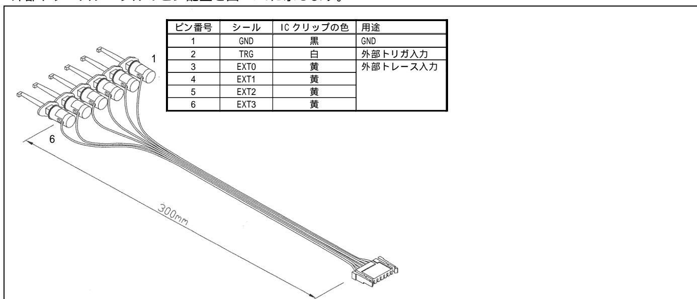
図 2.19 外部トレースケーブルのピン配置
