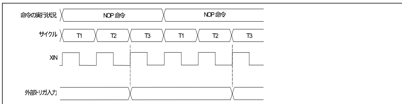
図 2.21 外部トリガ入力タイミング
