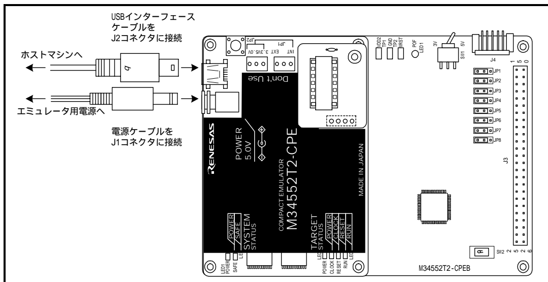
図 2.4 エミュレータシステムの接続
