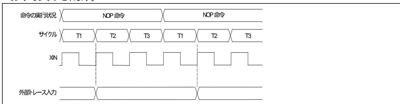
図 2.20 外部トレース入力タイミング
