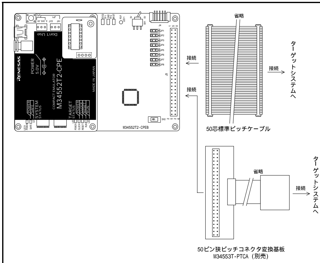
図 2.13 M34553T-PTCA接続方法
