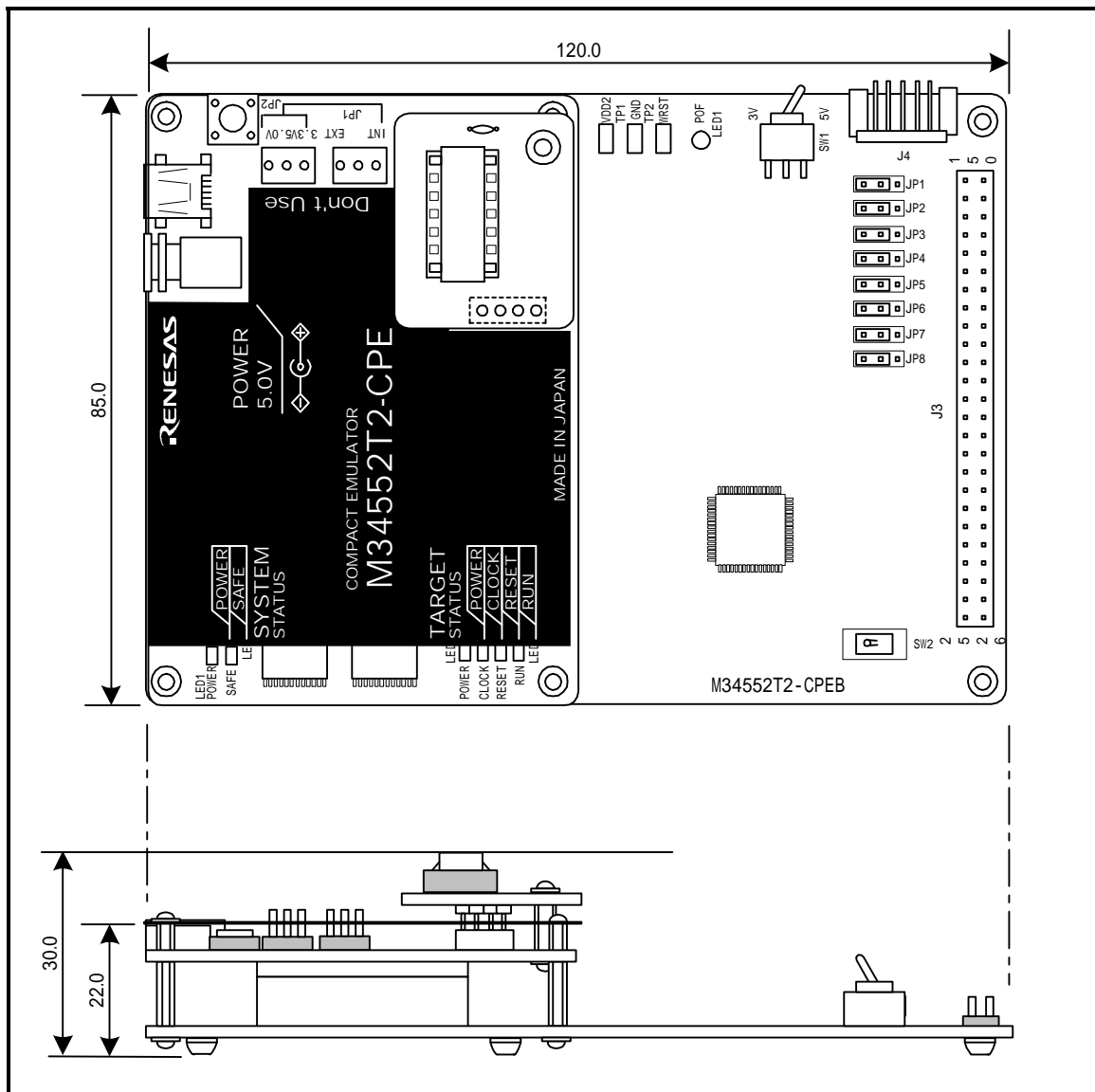
図 4.3 コンパクトエミュレータ全体寸法図
