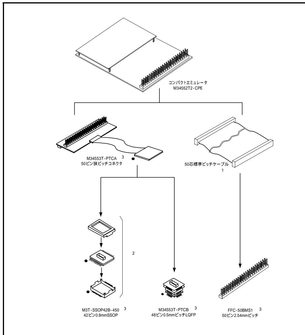
図 2.10 ユーザシステムとの接続
