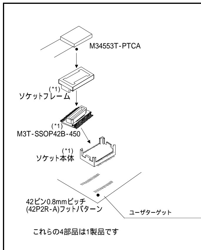
図 2.12 42ピンSSOPフットパターンの接続
