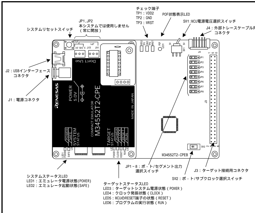
図 1.2 エミュレータ各部の名称(M34552T2-CPE上面)
