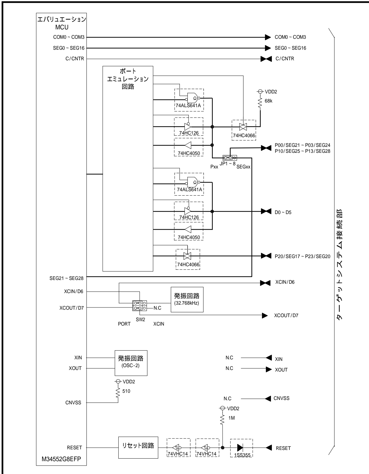
図 4.2 M34552T2-CPEの接続図(一部)
