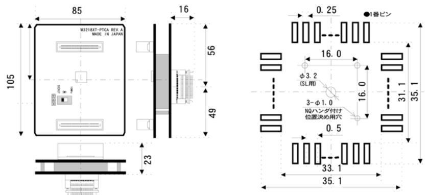
M32180T2-PTC 寸法図およびフットパターン参考寸法図(単位 mm)
