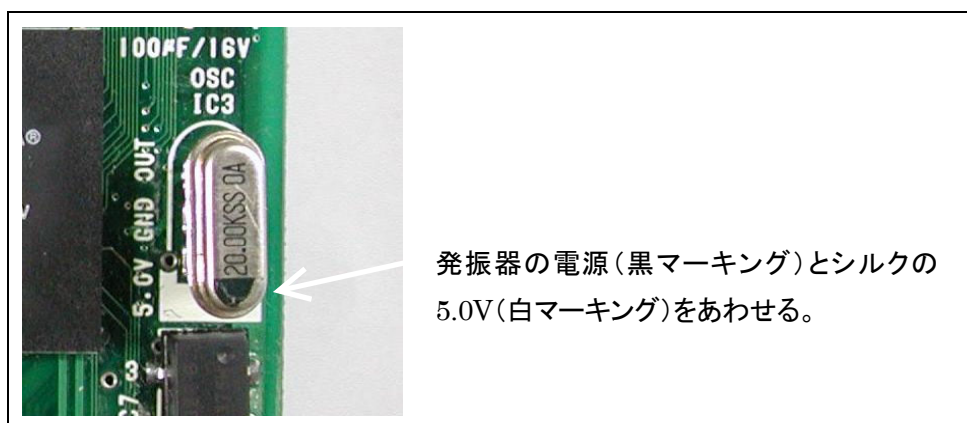
図 3.4 発振器の取り付け方向
