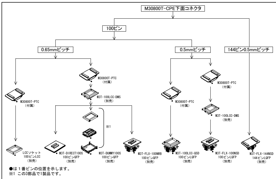
図 2.9 ターゲットシステムとの接続
