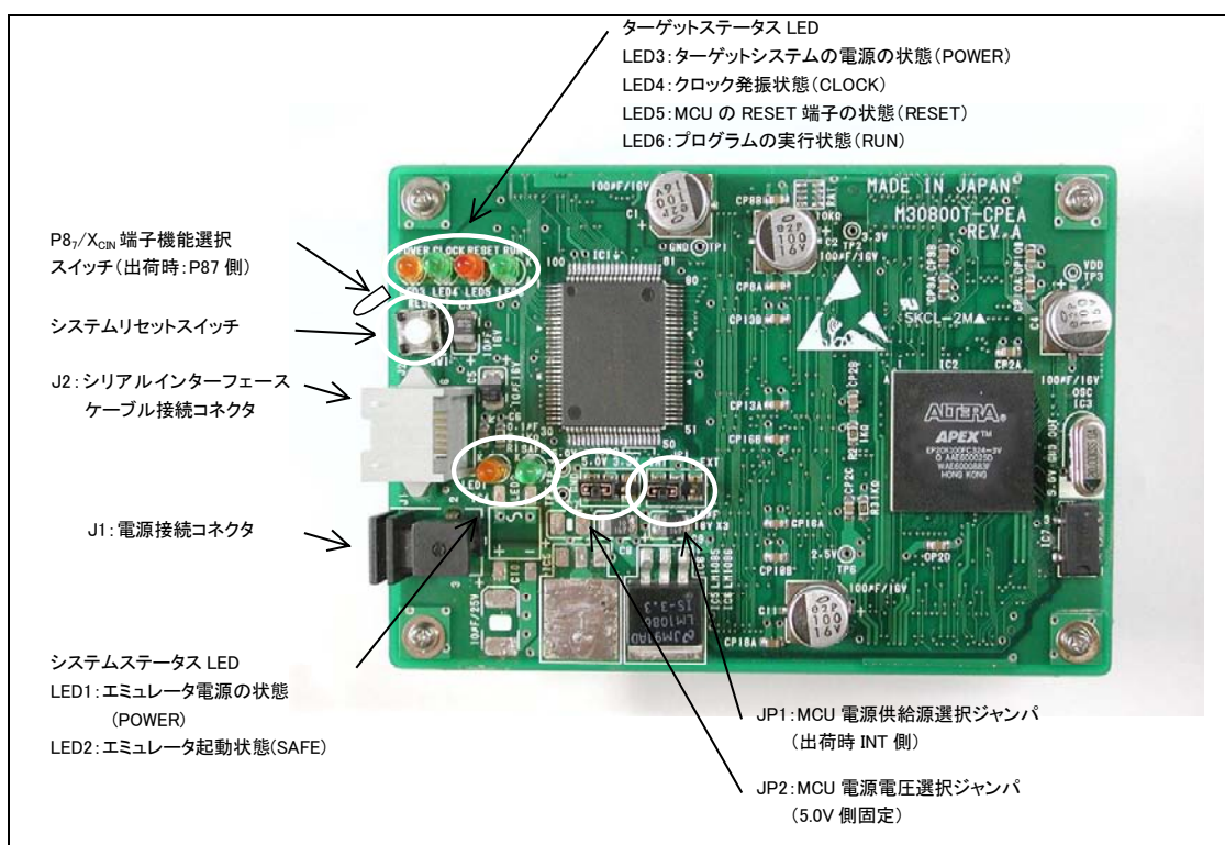
図 2.2 エミュレータ各部の名称(M30800T-CPE 上面)
