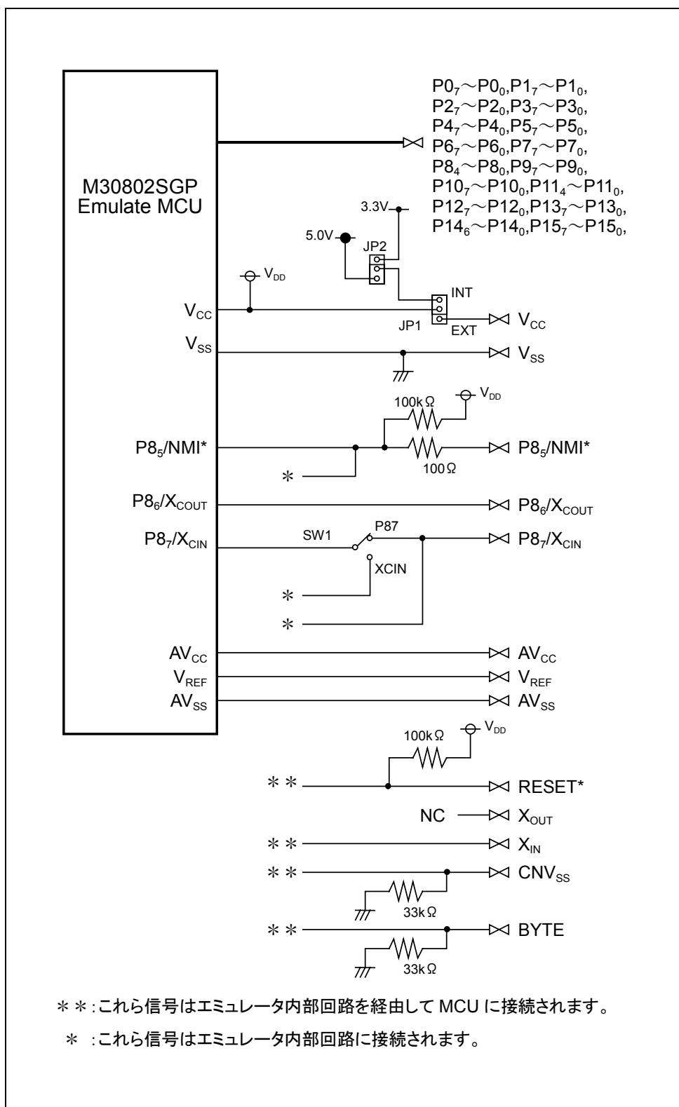
図 4.1 接続図(エミュレーション回路)
