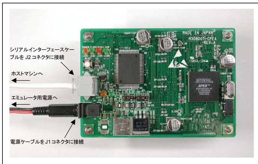
図 2.5 エミュレータシステムの接続
