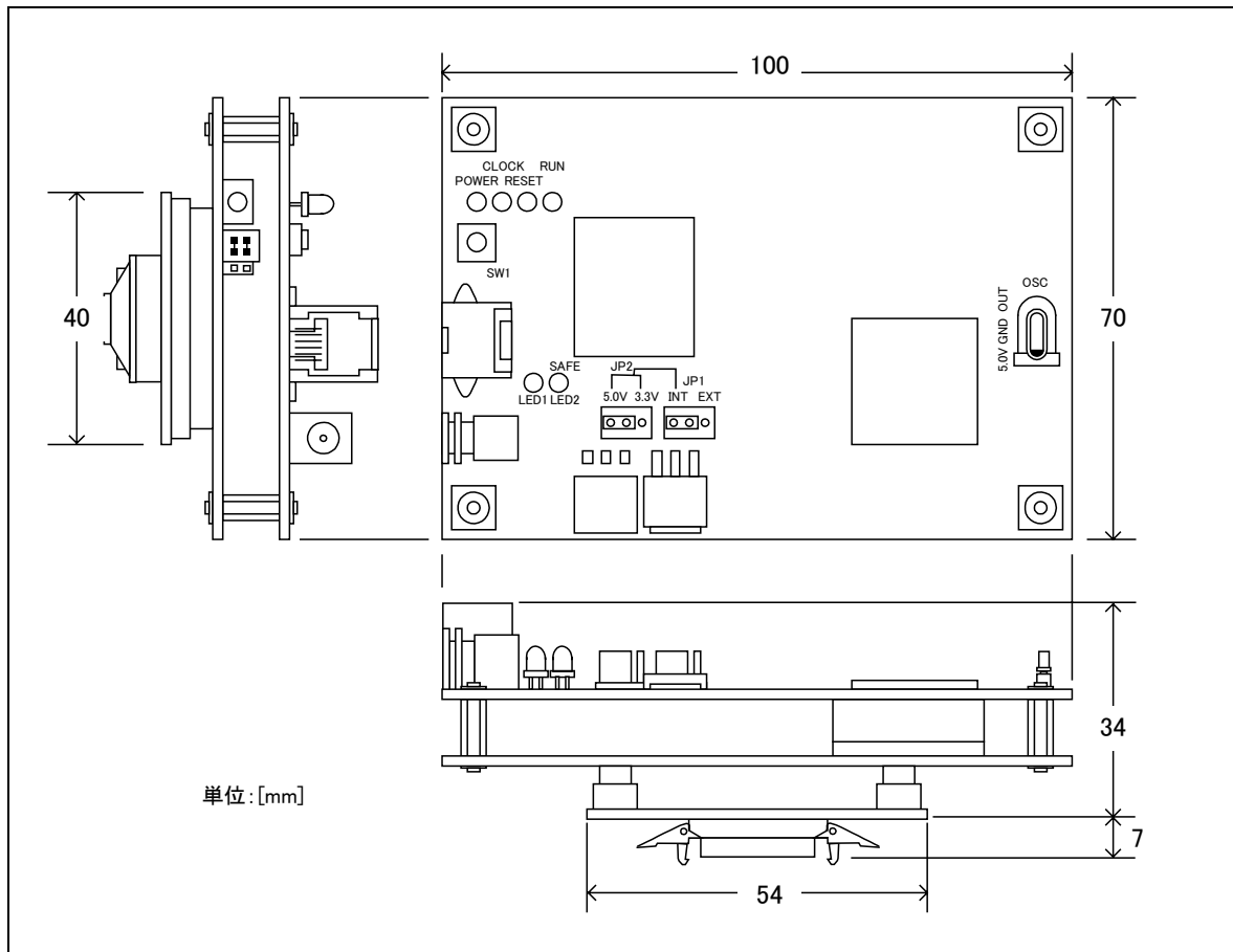
図 4.2 エミュレータ寸法図
