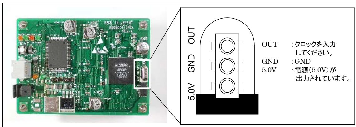
図 3.3 エミュレータ内蔵クロックの位置と回路仕様
