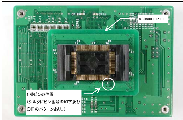
図 2.8 エミュレータ下面の LCC プローブ
