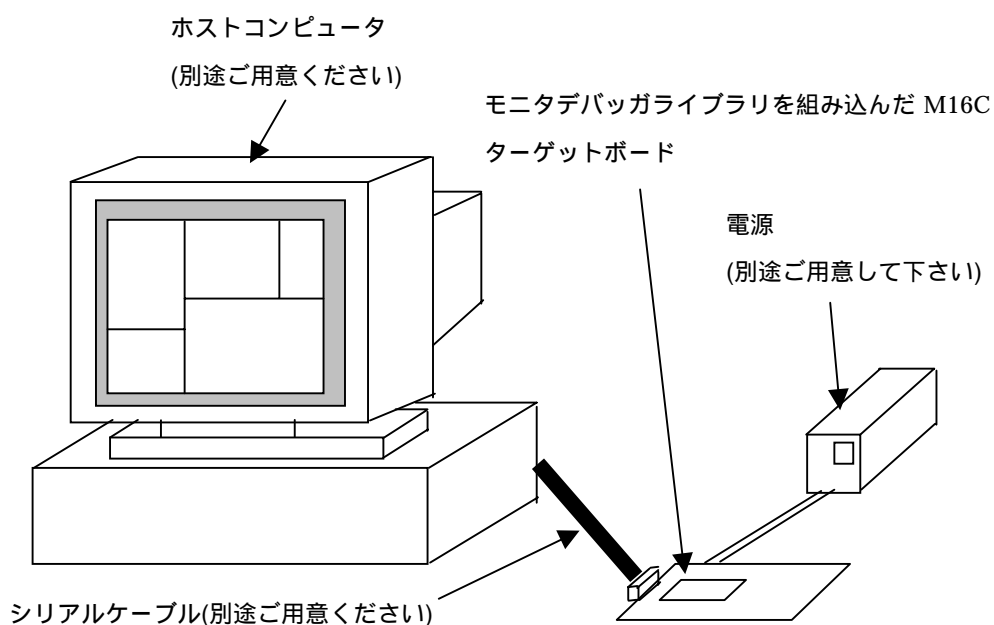
図 3-1 M16C/62N モニタデバッガライブラリのシステム構成図
