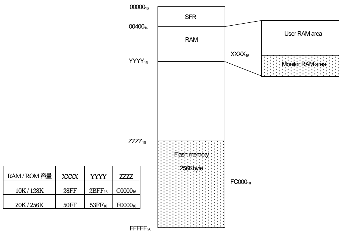
図 6-1 M16C/62N モニタデバッガメモリマップ
