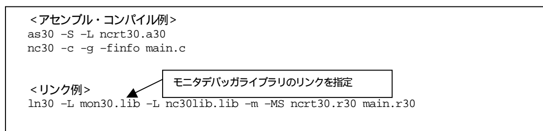
図 5-5 モニタデバッグライブラリのリンク例
