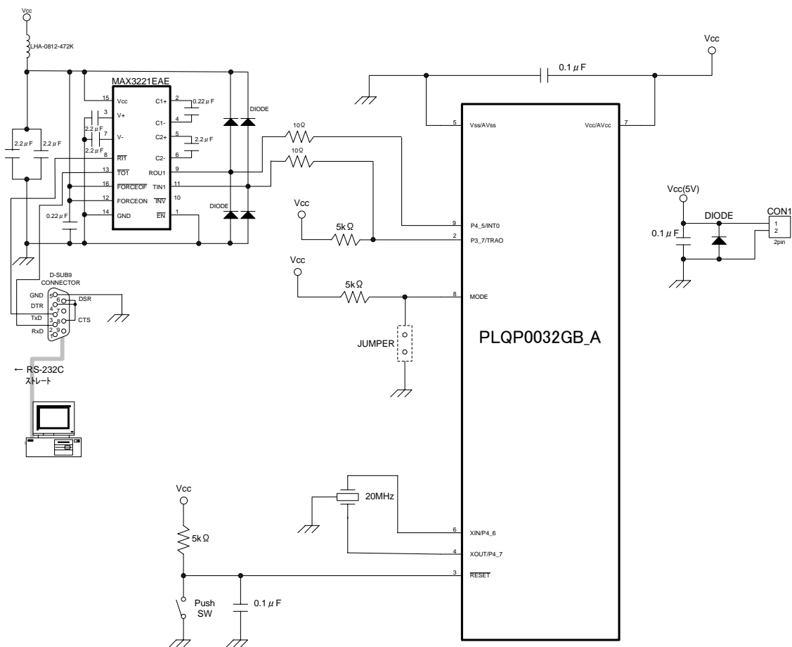
図 2 RS-232C ケーブルを使用した回路例(R8C/2E,2F グループ)
