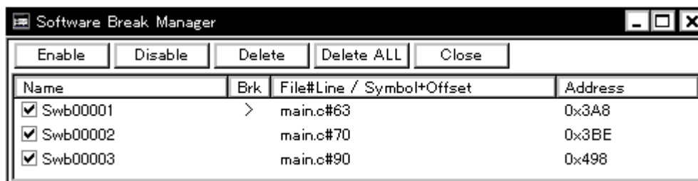
図 5-3 ソフトウェア・ブレークの管理
