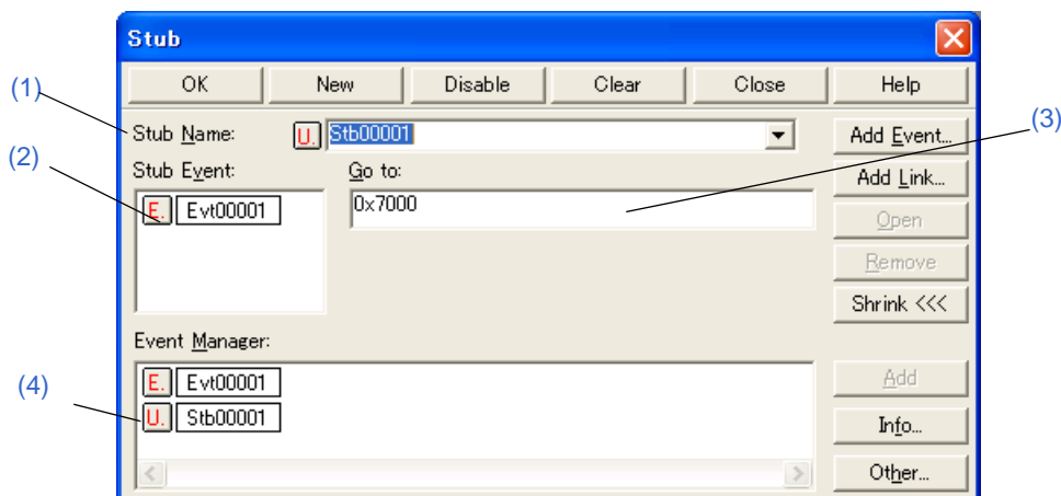
図 6 - 62 スタブ・ダイアログ
