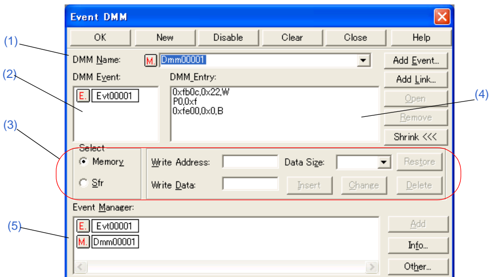
図 6 - 63 イベント DMM ダイアログ（メモリ選択時）
