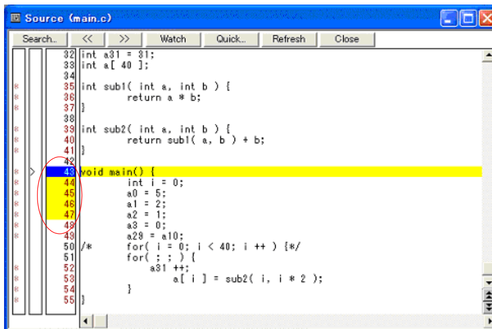
図 5 - 20 カバレッジ実行／未実行箇所の表示
