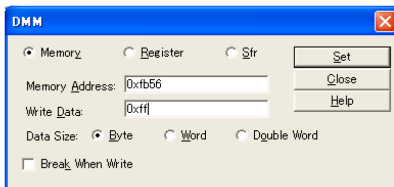
図 5 - 27 DMM ダイアログ
