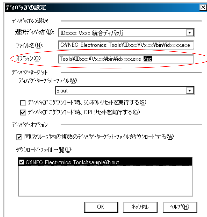
図 3-1 [ デバッグの設定 ] ダイアログ (PM+)
