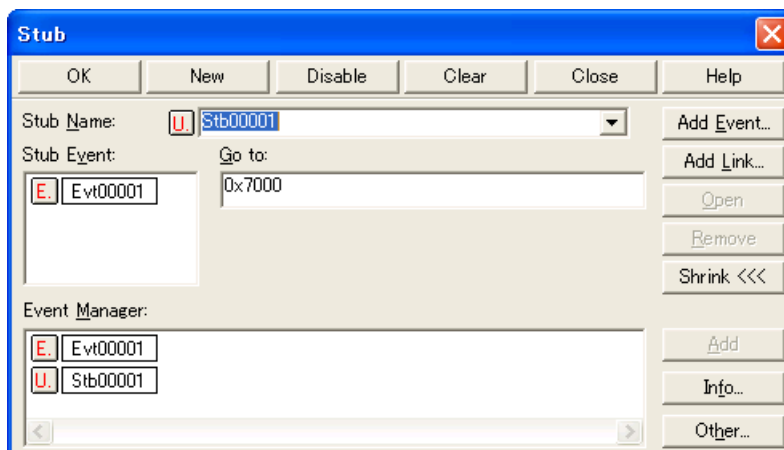
図 5 - 24 スタブ・イベント条件の設定
