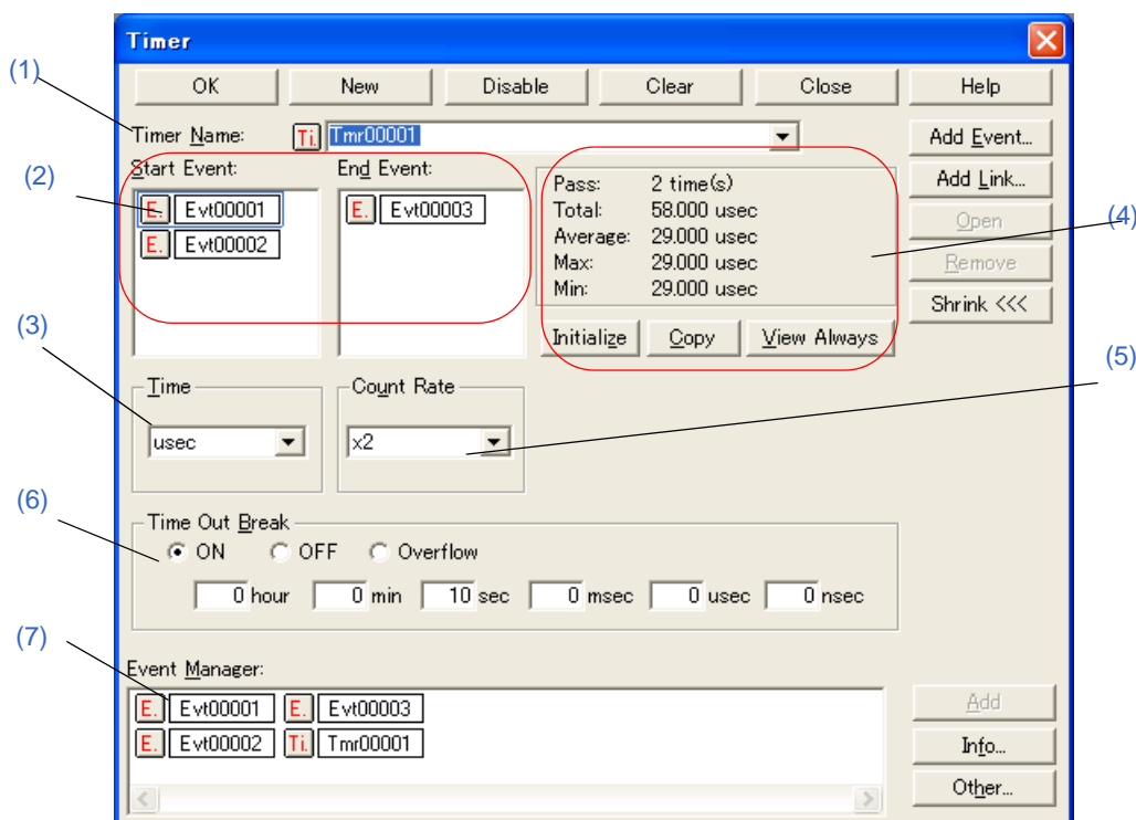
図 6 - 46 タイマ・ダイアログ
