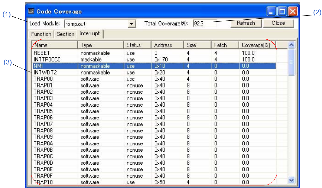
図 6 - 54 コード・カバレッジ・ウィンドウ
