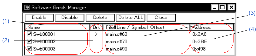
図 6 - 55 ソフトウェア・ブレーク・マネージャ
