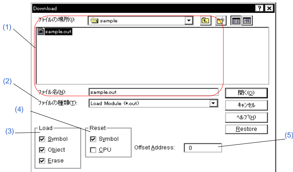
図 6 - 19 ダウンロード・ダイアログ
