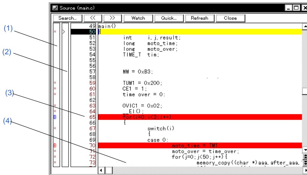
図 6-22 ソース・テキスト・ウィンドウ
