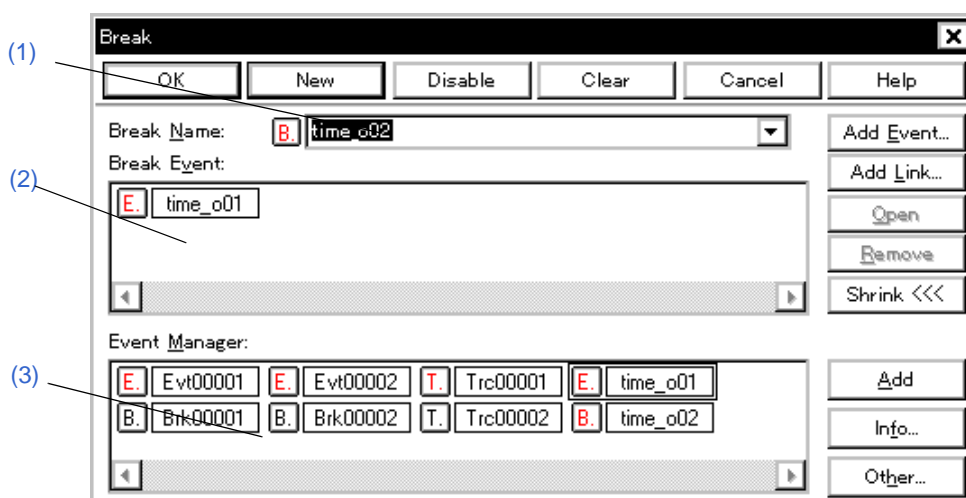
図 6 - 60 ブレーク・ダイアログ
