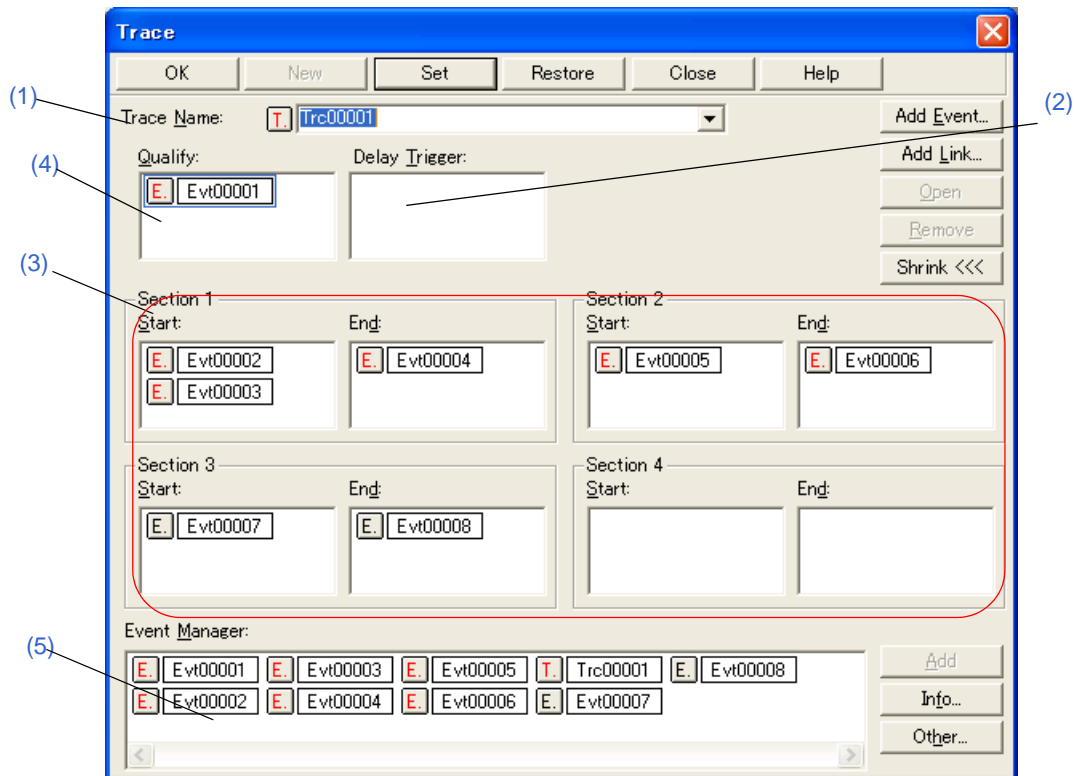
図 6 - 52 トレース・ダイアログ
