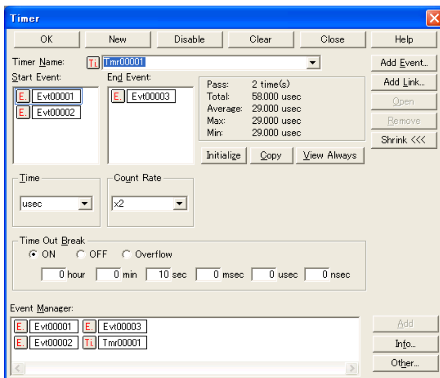
図 5 - 17 タイマ・イベントの設定, 表示 (タイマ・ダイアログ)
