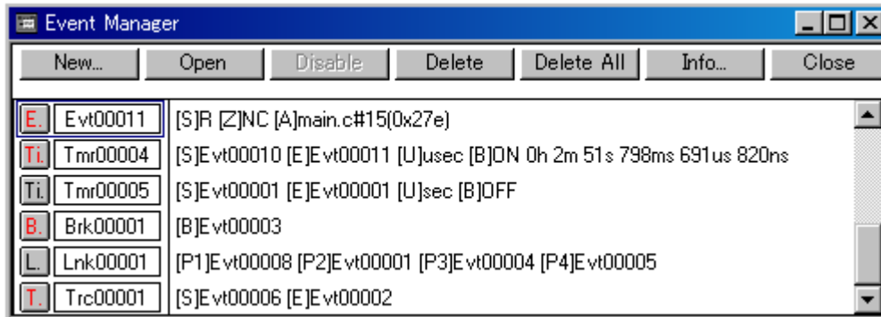
図 6 - 56 イベント・マネージャ（詳細表示時）
