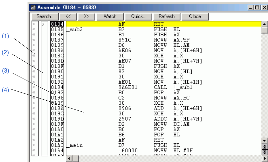
図6-25 逆アセンブル・ウィンドウ
