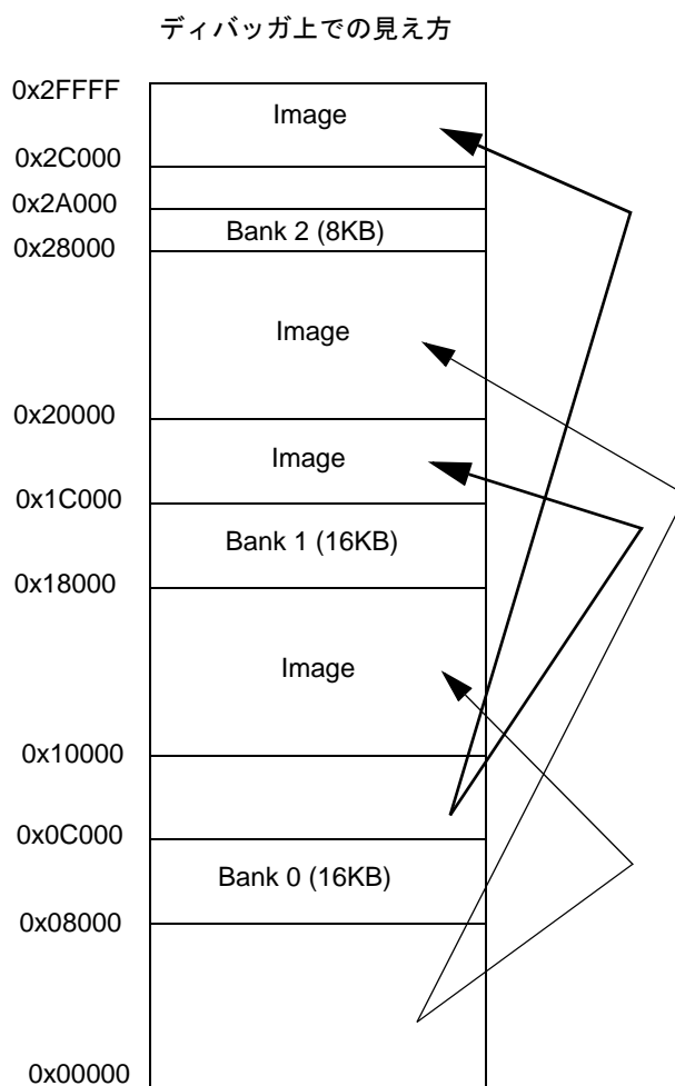
図6-7 内部ROMバンクを使用する場合のアドレス空間（内部バンクROMサイズ：40Kバイト）
