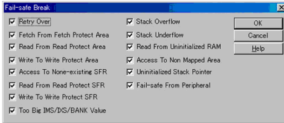
図 5 - 4 フェールセーフ・ブレイク設定
