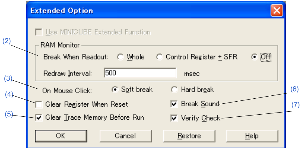
図 6 - 8 拡張オプション設定ダイアログ（IECUBE 接続時）
