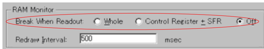
図 5 - 26 疑似リアルタイム RAM モニタ機能の指定
