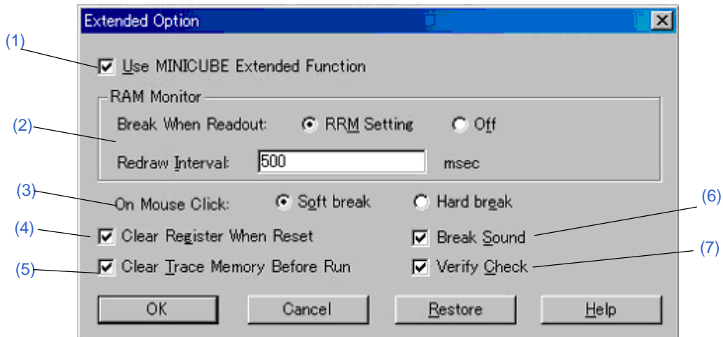
図 6 - 9 拡張オプション設定ダイアログ（MINICUBE 接続時）
