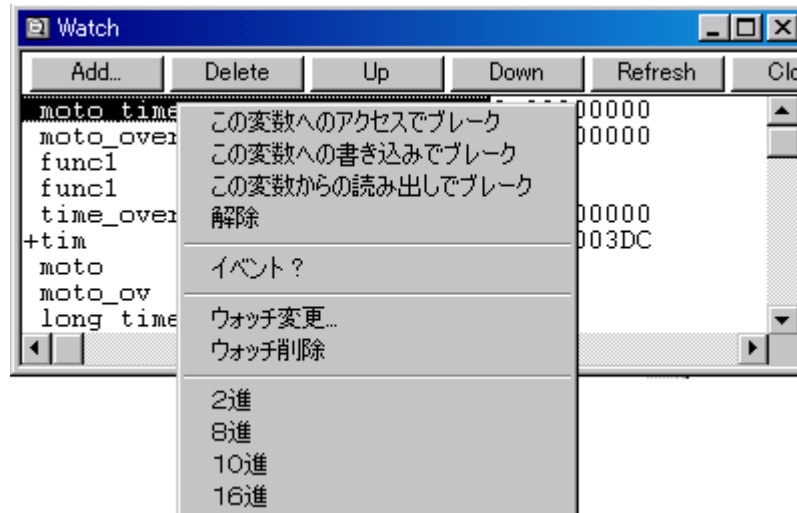
図5-2 変数へのブレーク設定
