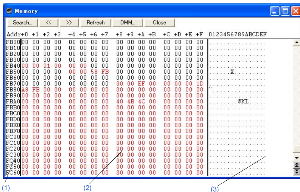
図 6 - 35 メモリ・ウィンドウ
