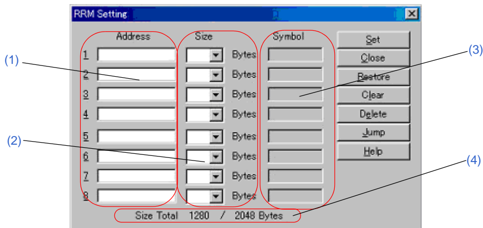
図 6 - 11 RRM 設定ダイアログ
