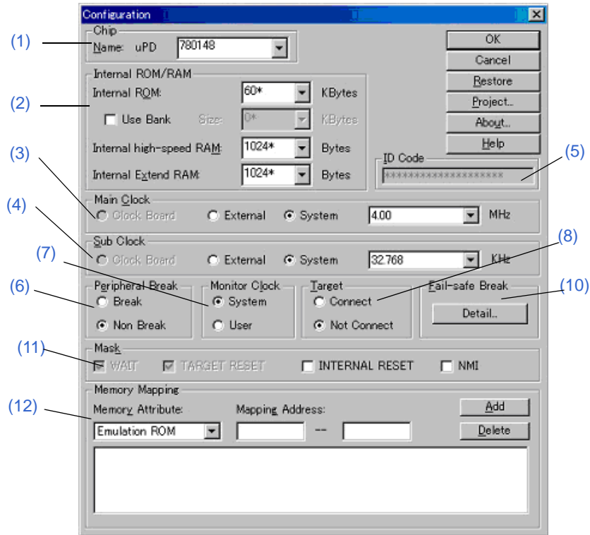
図 6-5 コンフィグレーション・ダイアログ（IECUBE 接続時）
