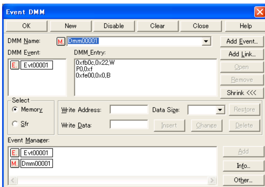
図 5 - 28 イベント DMM ダイアログ
