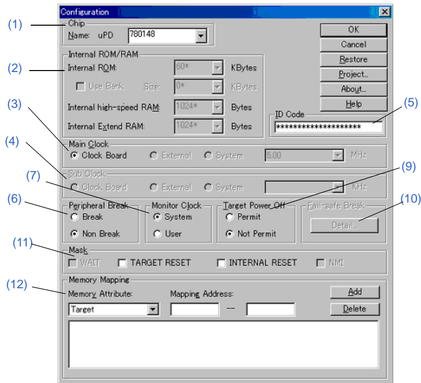
図 6 - 6 コンフィグレーション・ダイアログ (MINICUBE 接続時)
