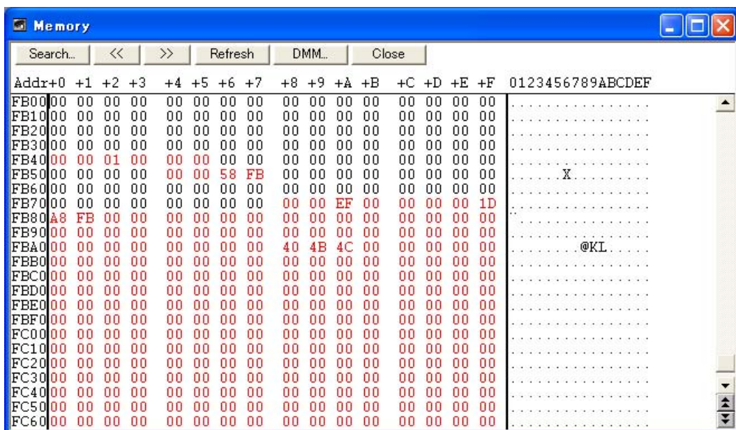
図 5 - 13 アクセス・モニタ機能 (メモリ・ウィンドウ)
