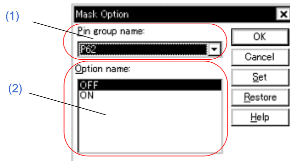
図 6 - 12 マスク・オプション設定ダイアログ
