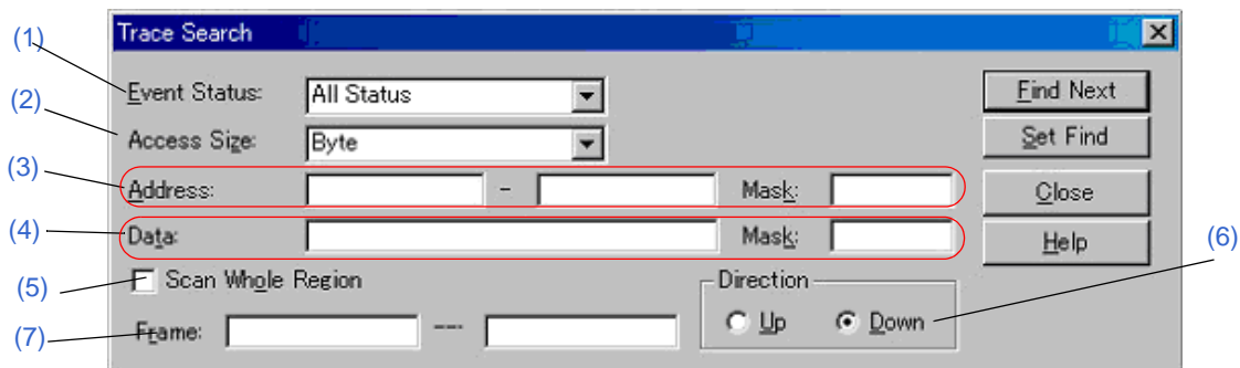
図 6-49 トレース・サーチ・ダイアログ
