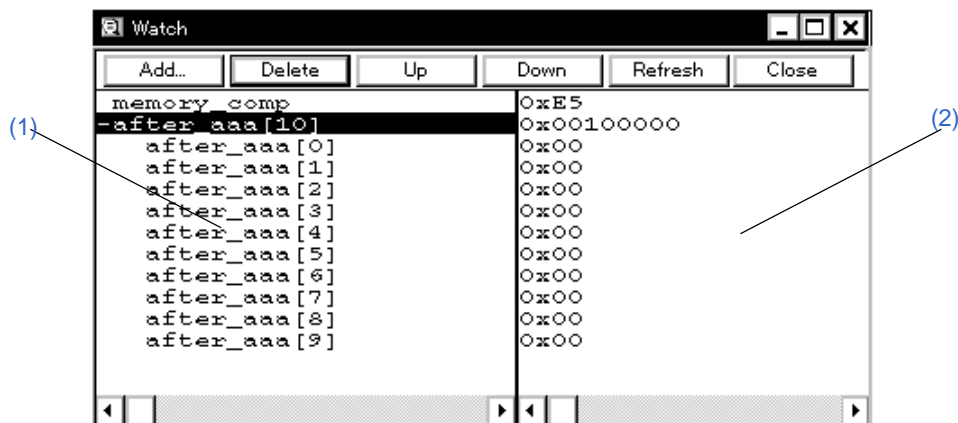
図 6 - 29 ウォッチ・ウィンドウ
