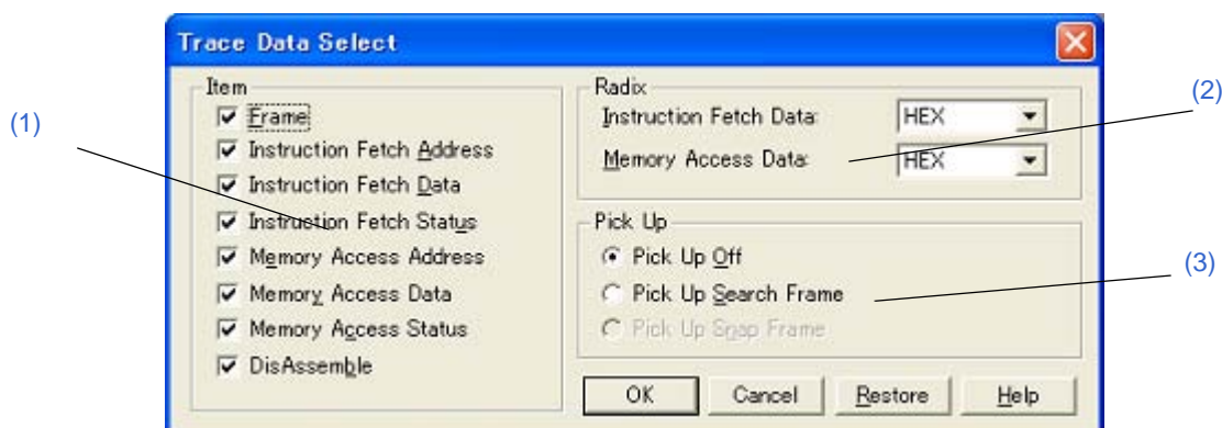
図 6 - 51 トレース表示選択ダイアログ
