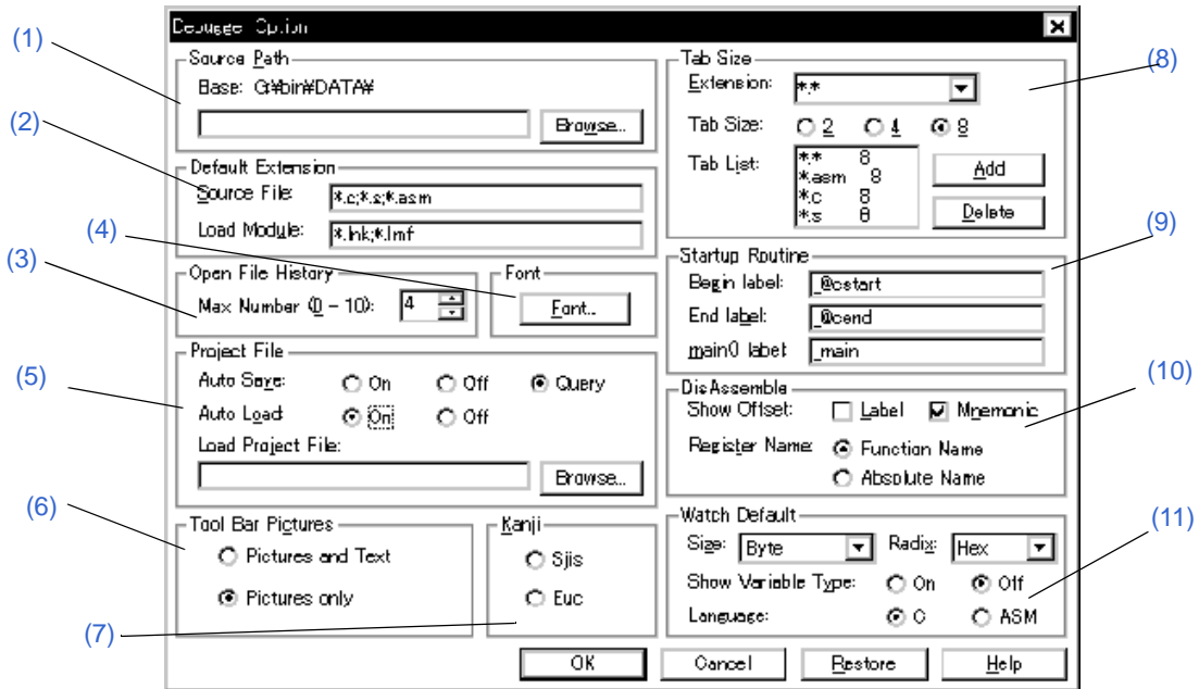
図 6 - 14 ディバッガ・オプション設定ダイアログ
