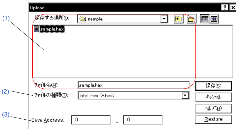
図 6 - 21 アップロード・ダイアログ
