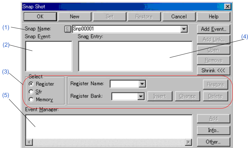
図 6 - 61 スナップショット・ダイアログ（Register 選択時）
