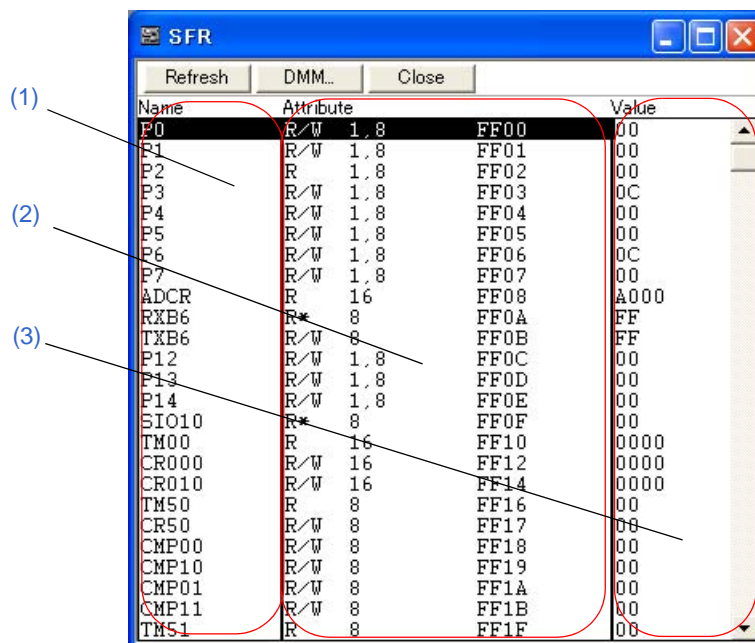
図 6 - 43 SFR ウィンドウ
