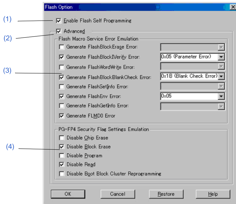
図 6 - 13 フラッシュ・オプション設定ダイアログ
