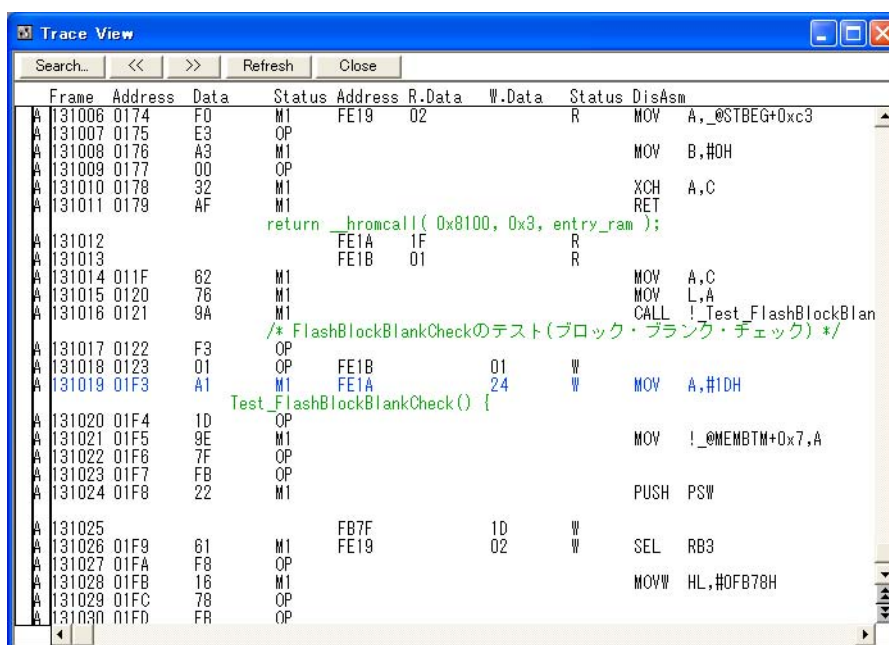
図 5 - 18 トレース・データの確認
