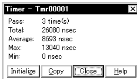
図 6 - 47 タイマ測定結果ダイアログ
