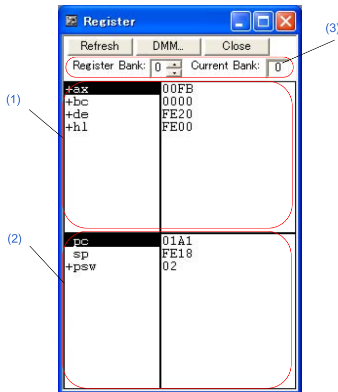
図 6 - 42 レジスタ・ウィンドウ
