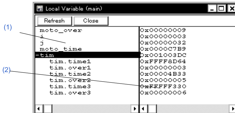
図 6 - 33 ローカル変数ウィンドウ
