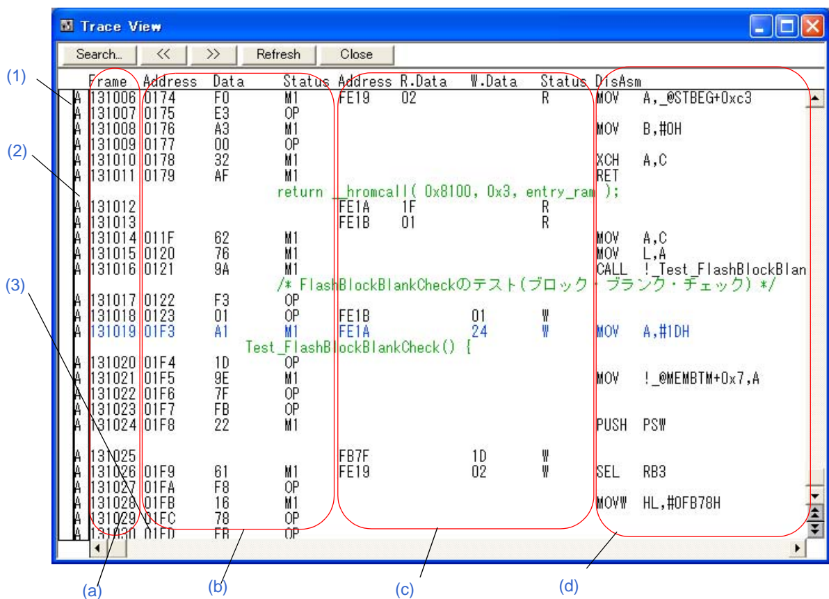
図 6-48 トレース・ウィンドウ
