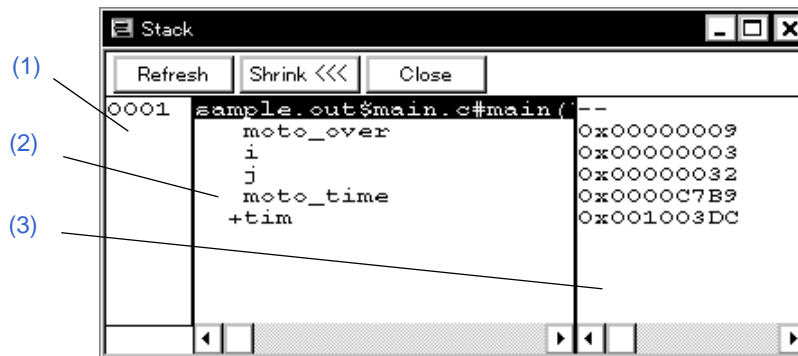
図 6 - 34 スタック・トレース・ウィンドウ
