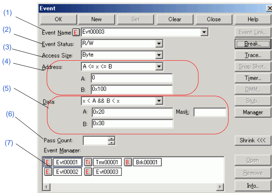
図 6 - 58 イベント・ダイアログ
